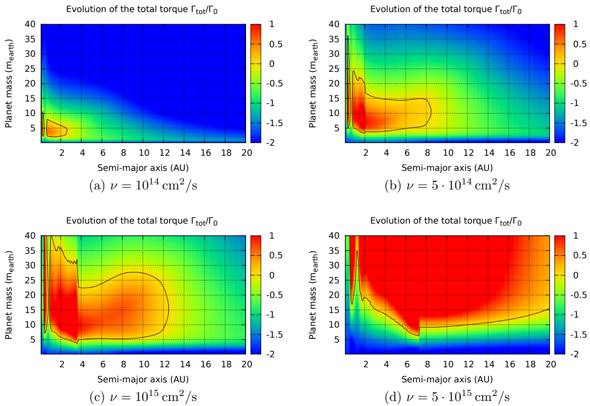
FIGURE 3.15 – Influence de la viscosité sur la carte de migration. Tous les autres paramètres sont identiques au disque de référence [§ 3.1 page 78].
