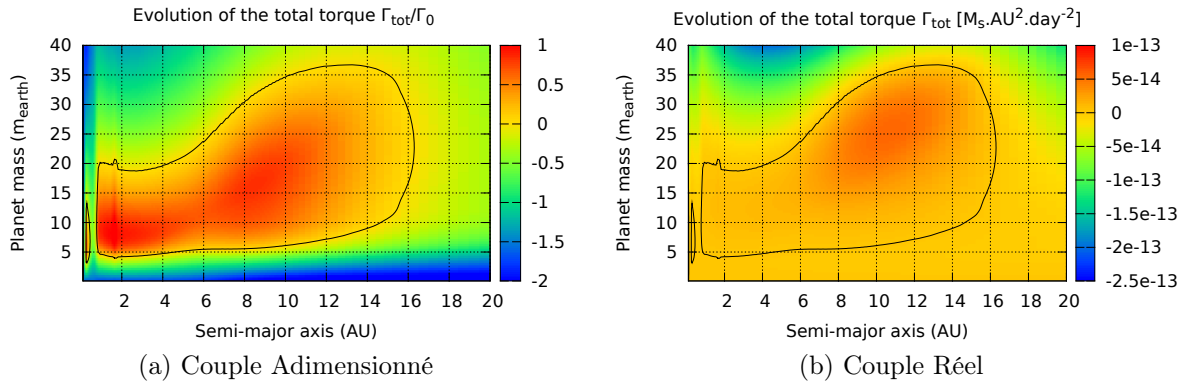
FIGURE 3.1 – Carte de migration pour le disque de référence. Cette carte montre le sens de migration d’une planète en fonction de sa position (abscisse) et de sa masse (ordonnée). La 3 e coordonnée est le couple total exercé par le disque sur la planète, exprimé en unité de \Gamma_0 = \left(\frac{q}{h}\right)^2 \Sigma_p r_p^4 \Omega_p^2 pour la carte de gauche, et en M_{\odot}\text{UA}^2/\text{jour}^2 pour la carte de droite. Quand le couple est positif (resp. négatif), la migration est vers l’extérieur (resp. intérieur). La ligne noire représente la zone de couple nul, où la planète ne migre plus. Des masses jusqu’à 40 M_{\oplus} sont affichées, dans l’unique but d’afficher des contours fermés. Il est probable qu’à de telles masses, une cavité s’ouvre autour de la planète, limitant la validité des formules de migration de Type I implémentés ici [Paardekooper et al., 2011]. Le détail des paramètres du disque de référence est donné [TABLE 3.1].
