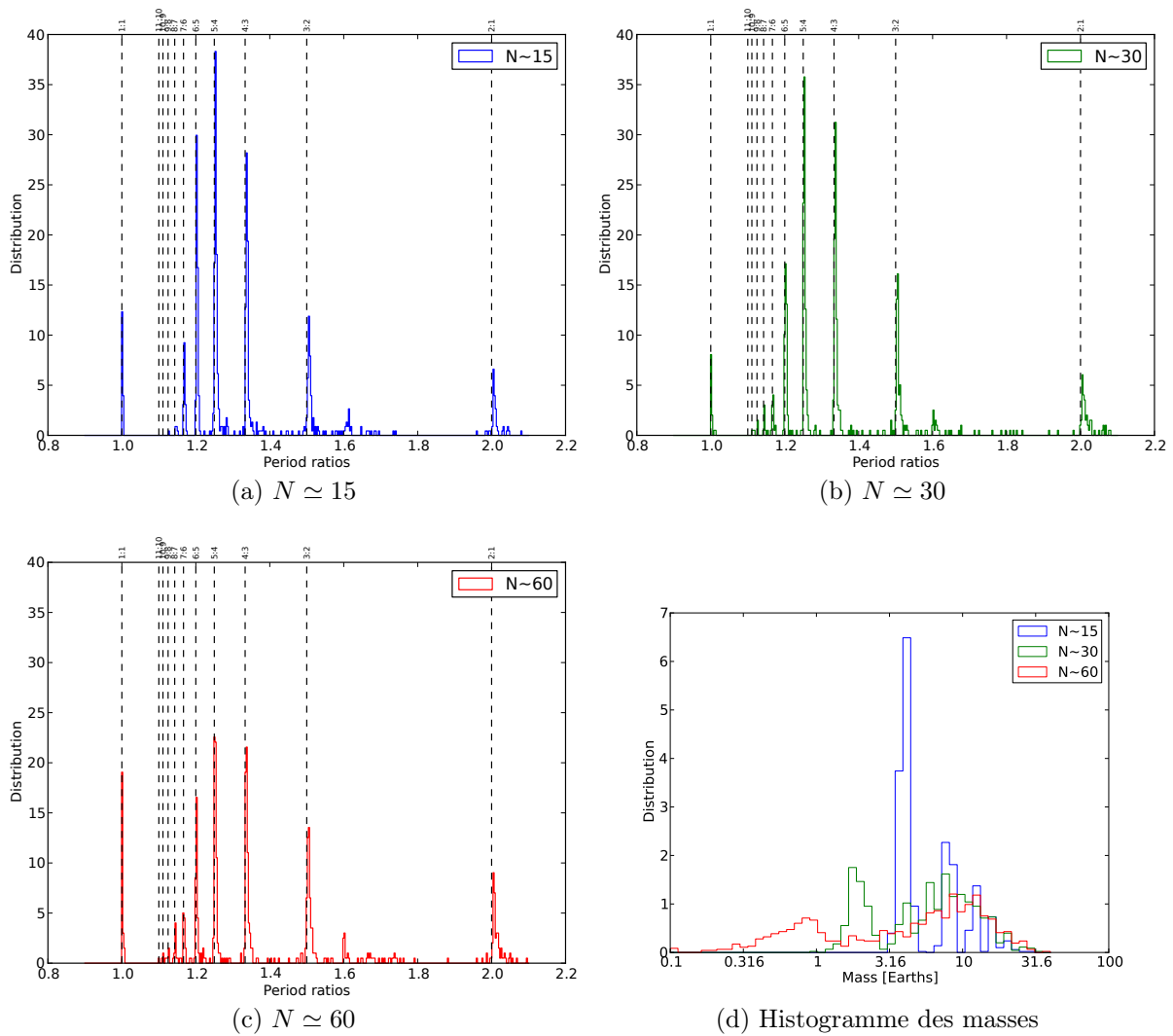
FIGURE 4.4 – Évolution des rapports de période orbitale et masses dans 100 systèmes planétaires où la masse totale est de 60 M_{\oplus} mais où le nombre total d’embryons varie autour de valeurs moyennes différentes (15, 30 ou 60).
