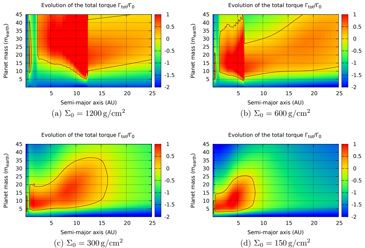
FIGURE 3.23 – Par rapport au disque de référence, possédant un profil de densité de surface \Sigma(R) = 300 \cdot R^{-1/2} \text{ g/cm}^2 nous représentons les cartes de migration pour des disques où nous avons changé la masse. D'en haut à gauche vers en bas à droite, ces cartes représentent les premiers stades de la dissipation du disque. Tous les autres paramètres sont identiques au disque de référence [§ 3.1 page 78].
