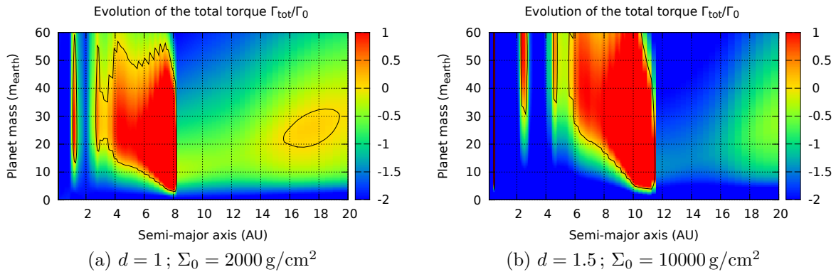
FIGURE 3.24 – Cartes de migration pour différents profils pour lesquels la masse du disque est constante entre R = 0.1 UA et R = 100 UA. La densité locale est la même pour R = 27 UA. Tous les autres paramètres sont identiques au disque de référence [§ 3.1 page 78].
