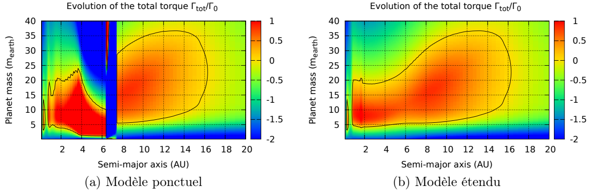
FIGURE 3.9 – Influence de la modélisation de l’ombre sur la carte de migration. Tous les autres paramètres sont identiques au disque de référence [§ 3.1 page 78].
