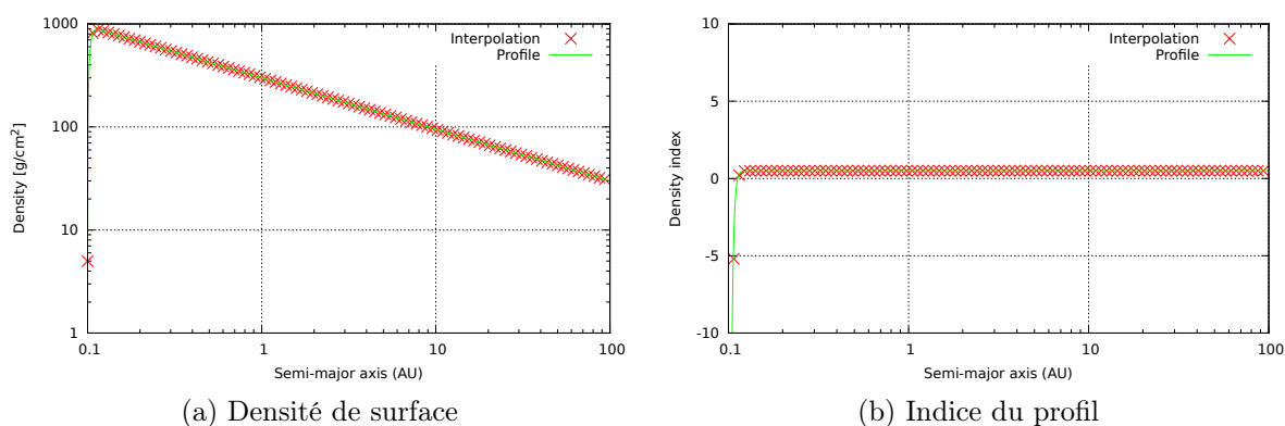
FIGURE C.5 – Résultat du test unitaire test_density_interpolation .
