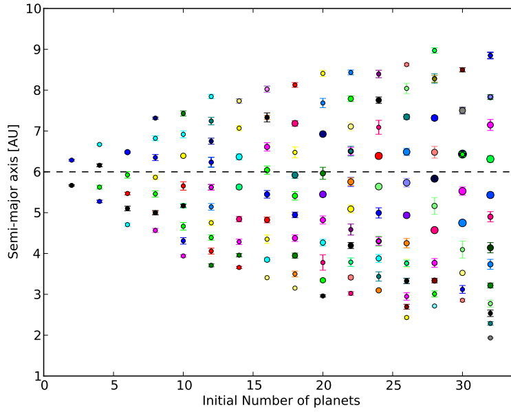
FIGURE 4.3 – Stabilisation d’un système planétaire autour d’une zone de convergence artificielle à 6 UA en fonction du nombre de planètes qui le compose initialement. Les excentricités sont représentées par les barres d’erreurs. Le diamètre des cercles représentant les planètes est proportionnel à leur rayon (en considérant qu’elles ont toutes la même densité).
