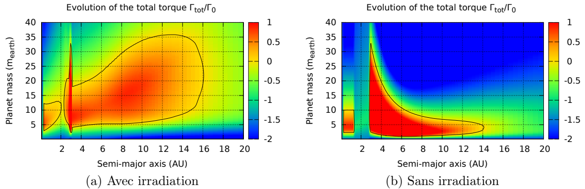
FIGURE 3.7 – Influence de l’irradiation sur la carte de migration à travers le profil de température. Afin de visualiser plus facilement les effets, l’opacité de Bell and Lin [1994] a été utilisée. Tous les autres paramètres sont identiques au disque de référence [§ 3.1 page 78].
