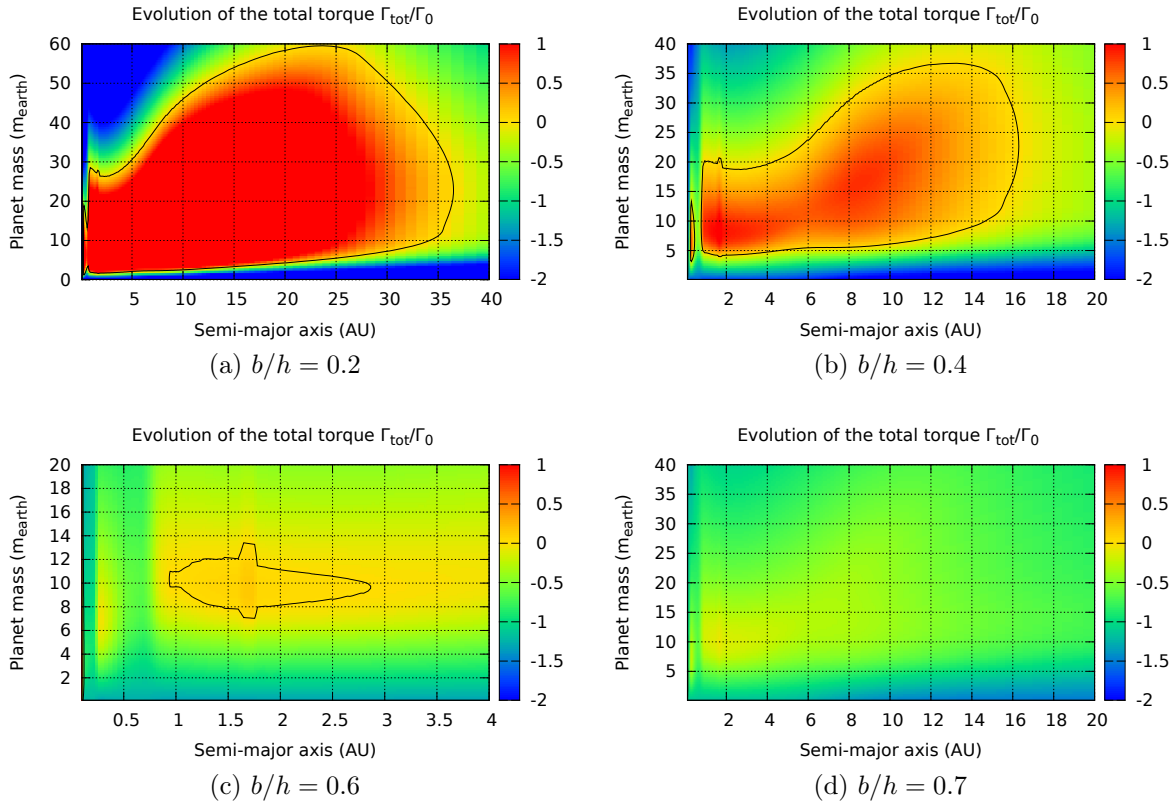
FIGURE 3.30 – Effet du paramètre de lissage b/h du potentiel gravitationnel sur la carte de migration du disque de référence. Tous les autres paramètres sont identiques au disque de référence [§ 3.1 page 78].
