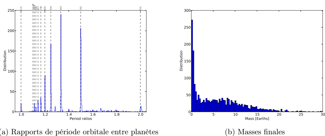
FIGURE 4.18 – Histogramme des rapports de périodes et des masses des planètes pour les 200 systèmes simulés.
