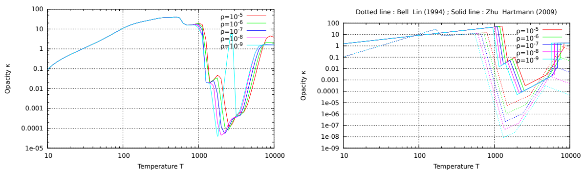
(a) Opacité de Huré [2000]
