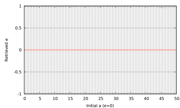
(b) Excentricité e
