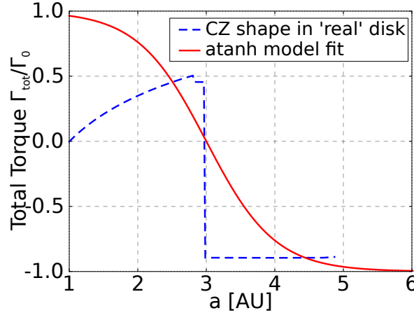
FIGURE 4.5 – Le couple total de notre disque standard est représenté en rouge. La ligne bleue pointillée représente le profil de couple ressenti par une planète de 10 M_{\oplus} autour d'une transition d'opacité, calculé à partir des équations de Paardekooper et al. [2011].
