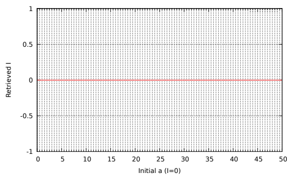
(c) Inclinaison I
