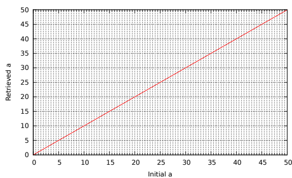
(a) Demi-grand axe a
