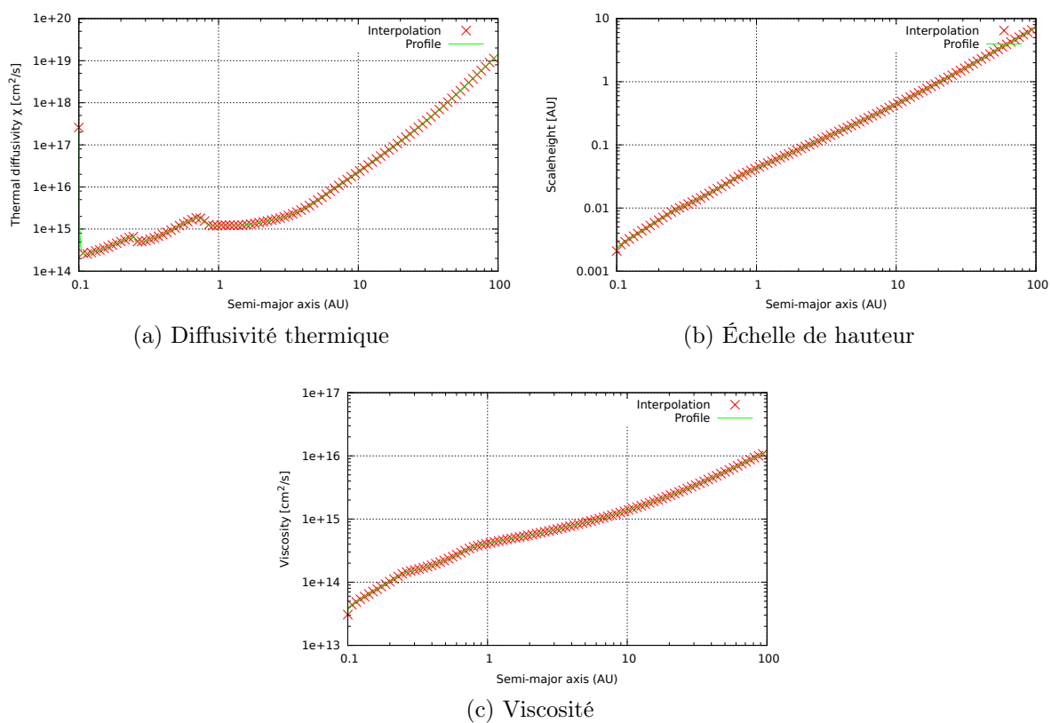
FIGURE C.11 – Autres profils du test unitaire test_temperature_interpolation .
