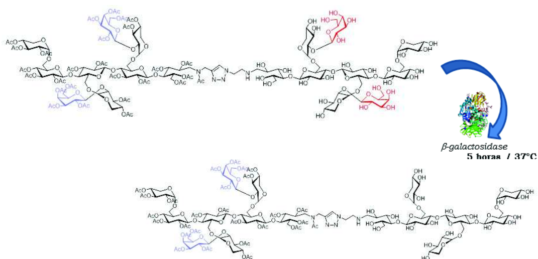
Figura 18. Digestão parcial do bloco hidrofílico do co-oligômero XGO- b -XGO,Ac por \beta -galactosidase ( 1\text{U mL}^{-1} , 5 horas, 37\text{ }^{\circ}\text{C} ).
