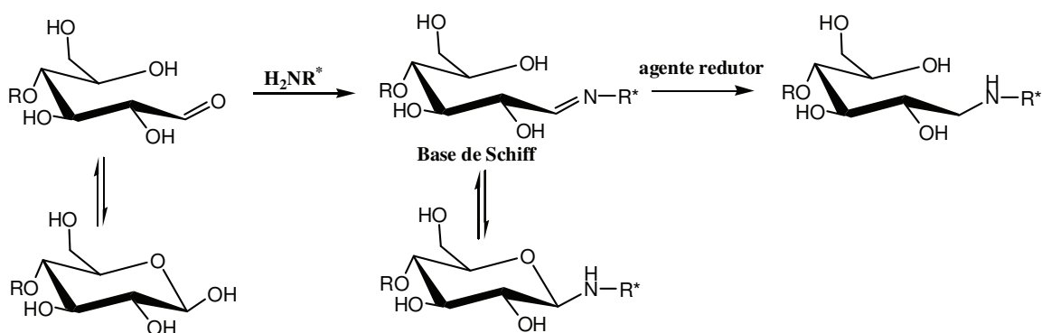
Figura 7. Aminoação redutiva de oligossacarídeos (DALPATHADO, JIANG, KATER, & DESAIRE, 2005).
