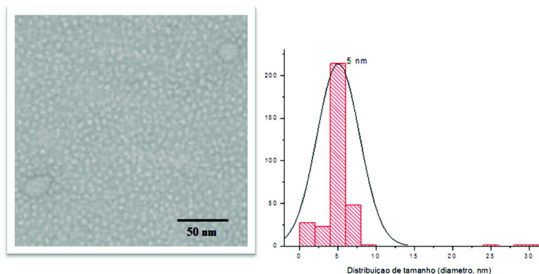
Figura 17. Micrografia de MET e distribuição médio do tamanho das micelas de DP7- b -DP7,Ac (3 mg mL -1 em água).
