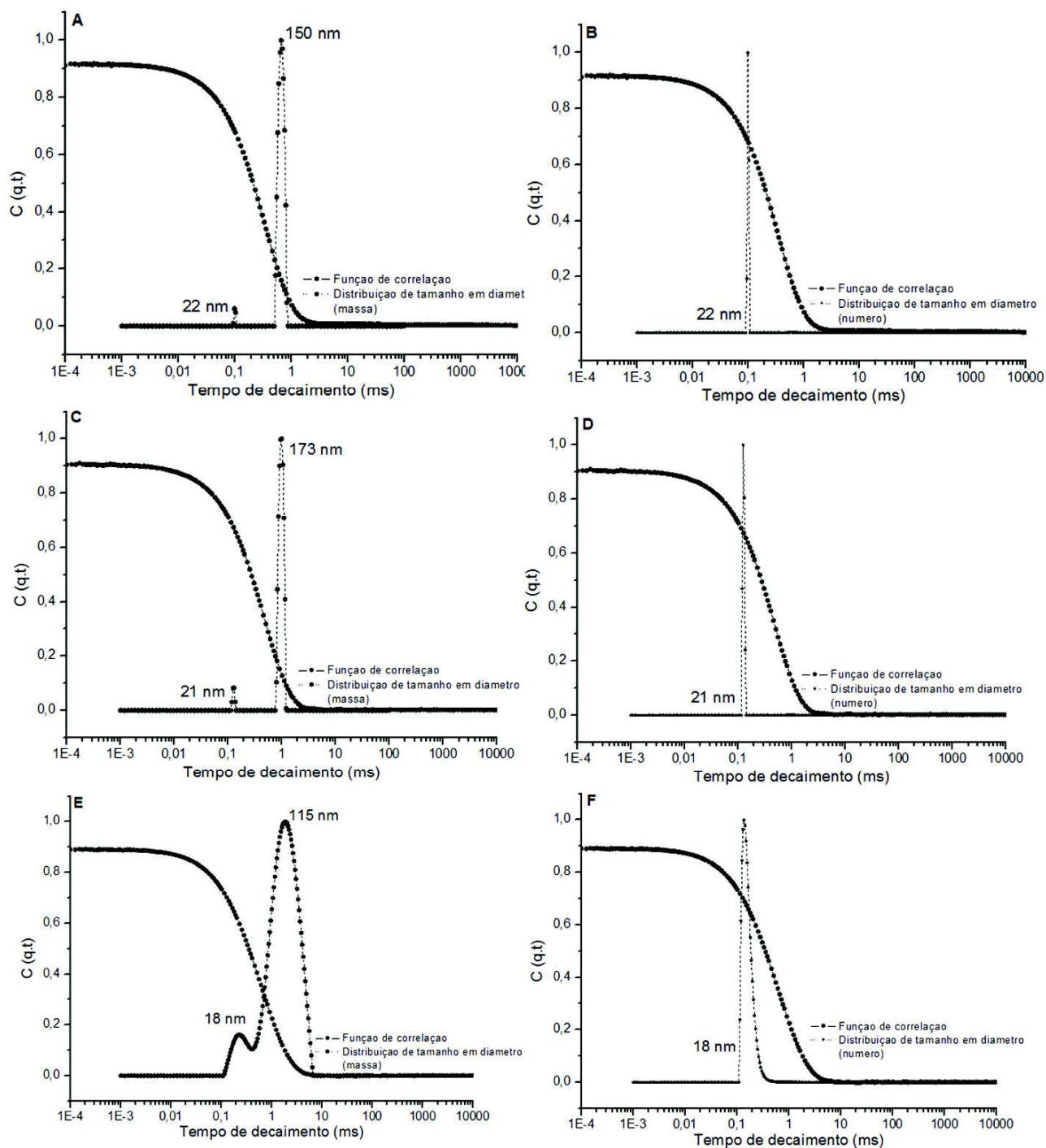
Figura 14. Função de correlação e distribuição do tamanho das micelas obtidas a partir da técnica de espalhamento de luz dinâmica para o co-oligômero XGO- b -XGO,Ac (A,B: 1 \text{ mg mL}^{-1} ; C,D: 3 \text{ mg mL}^{-1} ; E,F: 5 \text{ mg mL}^{-1} ).
