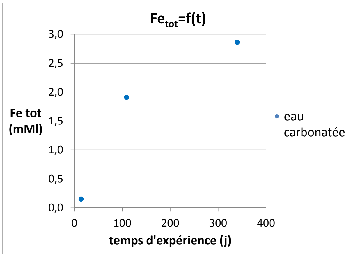
Figure 89: Fer total en solution des échantillons d'eau désaérée carbonatée non irradiée suivant la durée d'expérimentation
