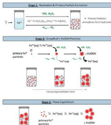
Figure 10: Mécanisme de formation de lépidocrocite colloïdale sous irradiation selon Yakabuskie[59]
