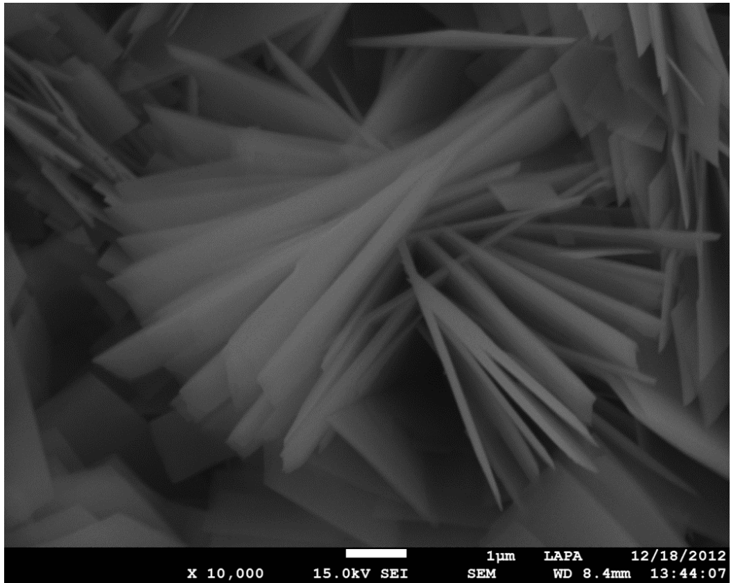
Figure 54: Cliché MEB-FEG des cristaux en rosace de la couche de produits de corrosion de l'échantillon A20 (395 kGy, 109 j)
