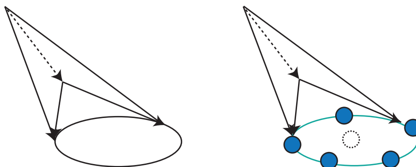
Figure 3.9. Cône catégoriel
