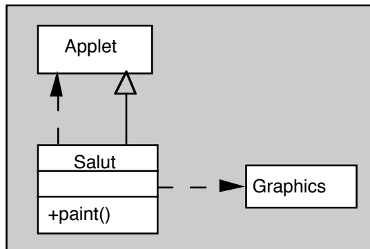
Figure 5.2. Eléments d'UML
