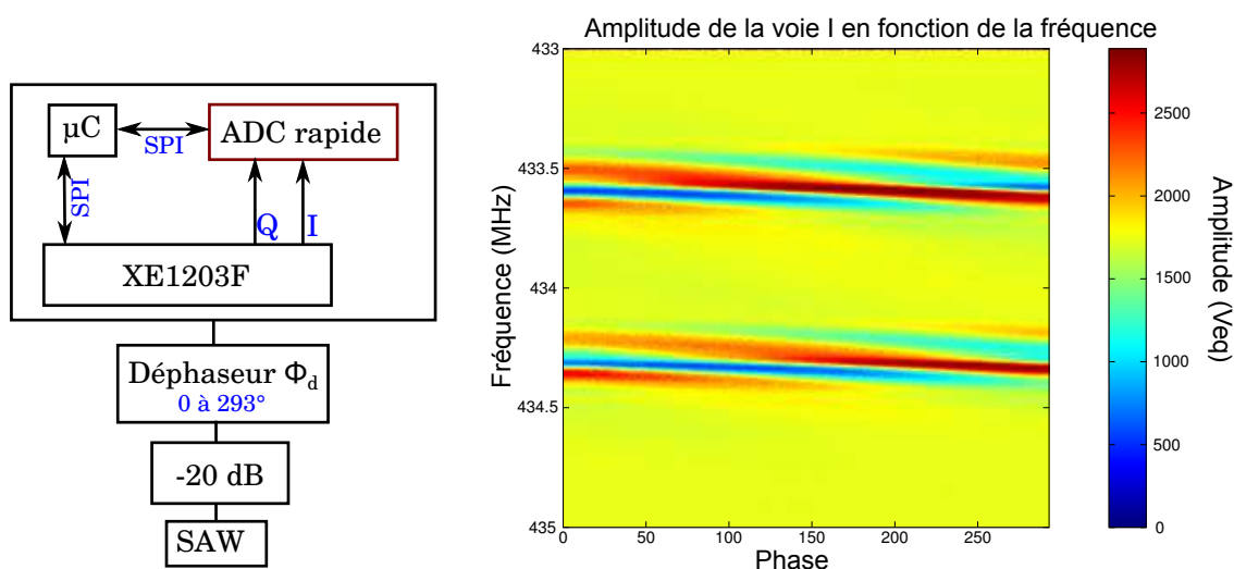
(a) Ajout d'un déphaseur et d'un ADC externe
