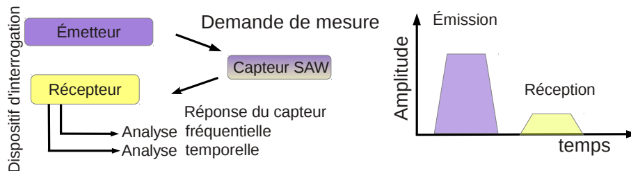
FIGURE 1.23 – Principe d'interrogation d'un capteur SAW
