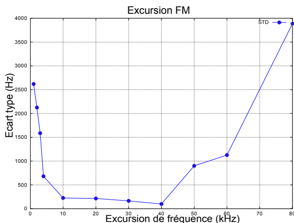
FIGURE 2.20 – Évolution de l'écart type de la fréquence en fonction de l'excursion du signal modulé. Pour une excursion trop faible ( < 10 kHz), le signal modulé est noyé dans le bruit. Pour une excursion trop grande ( \geq 50 kHz), le résonateur n'accumule pas suffisamment d'énergie. La valeur de l'excursion dépend du Q du résonateur : pour un résonateur de Q=10000 , l'excursion doit se trouver entre 10 kHz et 40 kHz.
