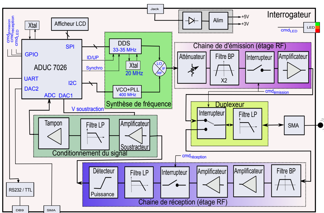
FIGURE 2.4 – Schéma bloc de l'interrogateur
