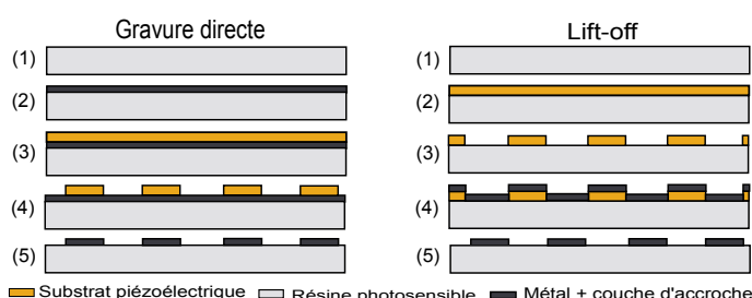
FIGURE 1.12 – Étapes technologiques pour la réalisation de peignes IDT à partir d'un wafer nu (1) : par gravure, (2) dépôt couche d'accroche et métal, (3) recouvrement de résine photosensible, (4) insolation et révélation de la résine, (5) gravure sèche ou humide de la couche métallique. Par lift-off : (2) recouvrement de résine photosensible, (3) structuration de la résine, (4) dépôt d'une couche d'accroche et de métal, (5) élimination de la résine et du métal qu'elle supporte.
