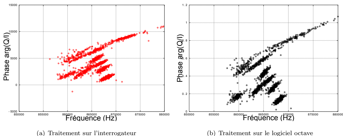
FIGURE 3.33 – Résultat fréquentiel de mesure d'un capteur SEAS10 dans une cavité fermée (abscisse) en fonction de la phase de l'intercorrélacion (mesurée par \arctan(Q0/I0) ) (en ordonnée); (a) Algorithme réalisé sur le lecteur; (b) Traitement réalisé avec les données du lecteur sur le logiciel octave. Dans les deux cas un biais fréquentiel apparaît en fonction de la position du capteur dans la cavité, créant des paliers de fréquences sur la mesure.
