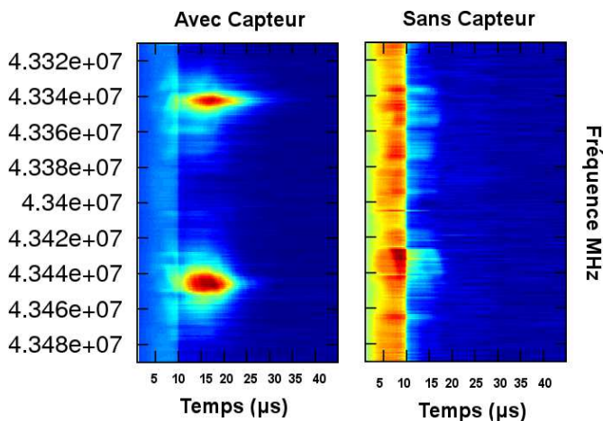
FIGURE 3.10 – En appliquant un filtre passe-haut pour enlever la composante continue suivi d'un redressement de la tension et d'un filtre passe-bas sur la valeur absolue du signal acquis, l'image de la réponse temporelle du capteur SAW peut être tracée avec le logiciel GNU/Octave pour déterminer les fréquence de résonance.
