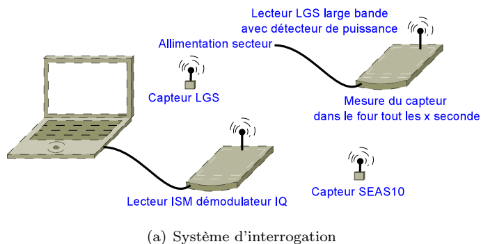
FIGURE 4.9 – (a) Schéma de principe de fonctionnement pour le multiplexage temporel ; (b) photo de la démonstration sur le salon Micronora : un système se trouve devant le four et un autre derrière le four pour sonder le capteur à l'intérieur de celui-ci.
