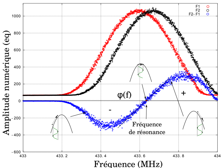
FIGURE 2.22 – Validation de l'apparition de la phase avec le mode deux points avec \Delta\omega = 10 \text{ kHz} . La soustraction F2-F1 permet d'obtenir le signe positif ou négatif de la phase.
