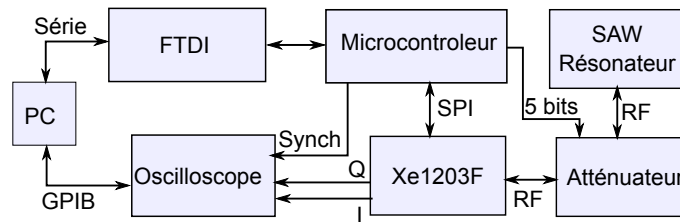
FIGURE 3.6 – Schéma de l'expérience de la validation du module Semtech pour l'interrogation d'un résonateur SAW. L'émission de fréquence dure 30 \mu\text{s} pour charger le résonateur, puis on passe en mode réception pendant 50 \mu\text{s} après commutation du switch, avec acquisition du signal I et Q par l'oscilloscope. Ce mode opératoire est répété pour couvrir toute la bande ISM par pas de fréquence prédéfini dans le but d'observer la réponse des résonateurs SAW.
