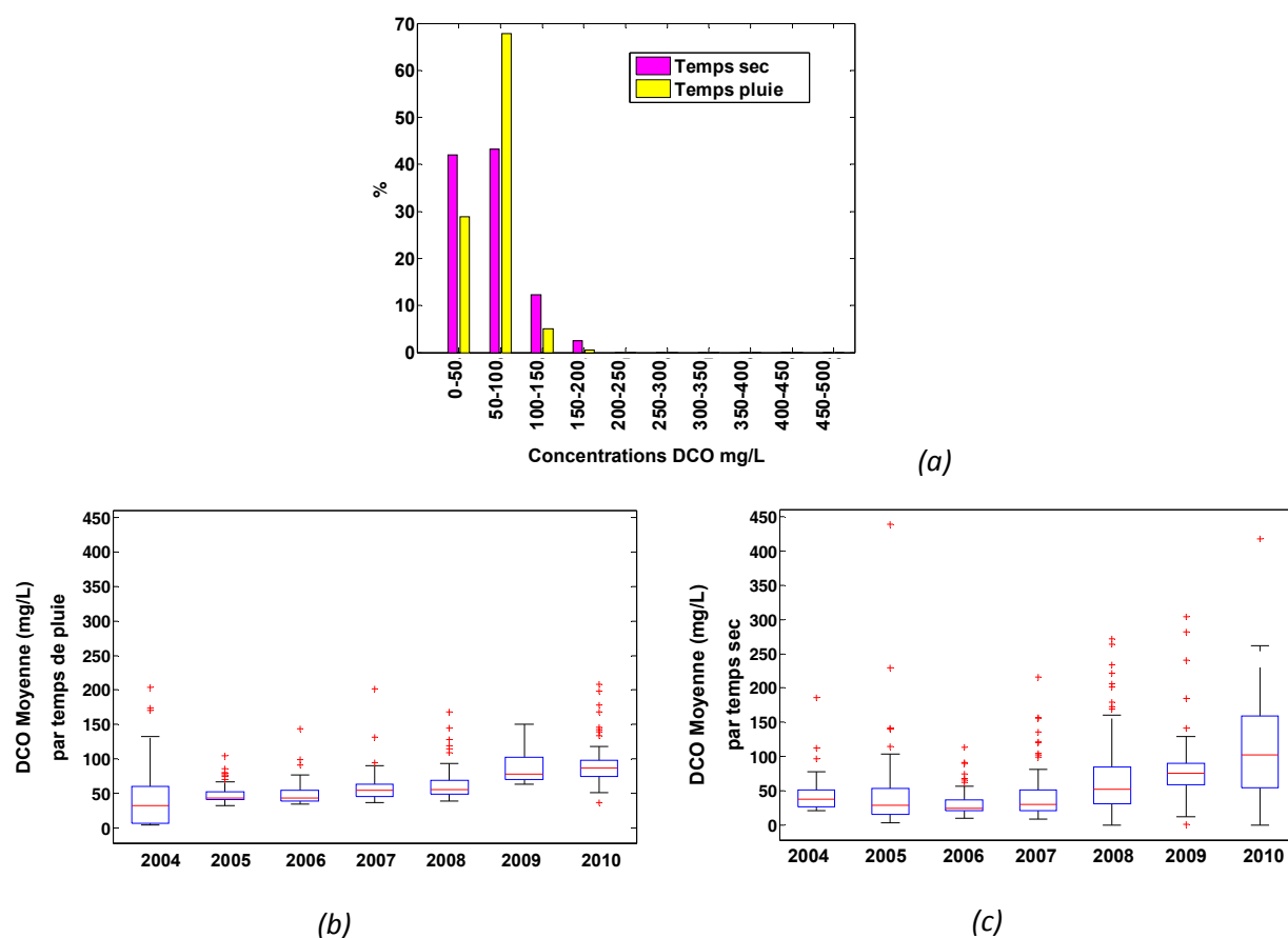
Figure 3-5. (a) Distribution des concentrations moyennes évènementielles de DCO (mg/L) apportées à l'ouvrage pour les évènements pluvieux et pour les périodes de temps sec. (b) Distribution des concentrations évènementielle de DCO apportées sur une année, pour les évènements pluvieux. (c) Distribution des concentrations de DCO apportées pour les périodes de temps sec à l'échelle de l'année.
