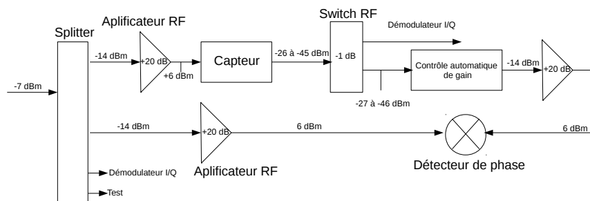
FIGURE 3.21 – Bilan de liaison de notre système pour l'utilisation du contrôle de gain automatique et du déphaseur.
