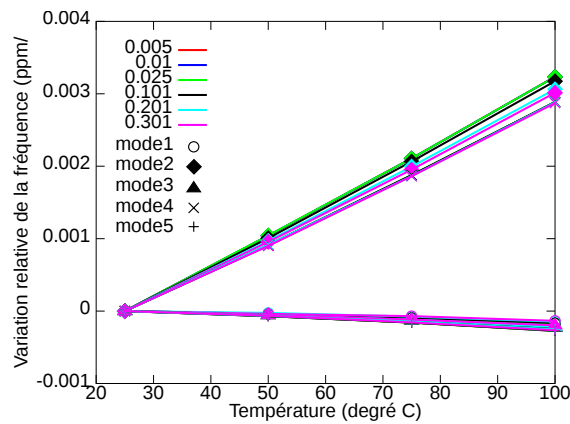
FIGURE 2.36 – Représentation des cinq modes choisis pour le calcul des sensibilités gravimétriques d’un HBAR \text{LiNbO}_3 (YX1)/163° sur quartz (YXlt)/34°/45° sur ces résonances. (a) Distribution spectrale considérée pour l’analyse. (b) Évolution de la sensibilité gravimétrique pour les cinq modes en fonction de l’épaisseur déposée et de la température.
