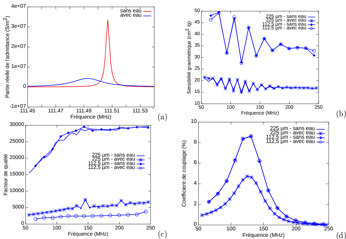
FIGURE 2.23 – Simulation d'un résonateur HBAR LiNbO 3 (YXl)/163° sur quartz (YXlt)/32°/90° pour une gamme de fréquence allant de 50 à 250 MHz. L'effet d'un ajout d'eau est représenté en (a), ainsi que la sensibilité gravimétrique (b), le facteur de qualité (c) et le coefficient de couplage (d) pour chaque résonance et pour deux épaisseurs de quartz, avec et sans eau.
