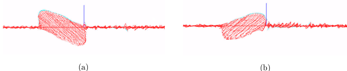
FIGURE 2.34 – Représentation du déplacement à la surface du substrat pour les ondes élastiques générées pour deux fréquences, 1,3892 (a) et 1,4114 GHz (b). La polarisation orthogonale des deux modes est ainsi visualisée, laissant présager d'une sensibilité différente aux conditions environnementales du capteur.
