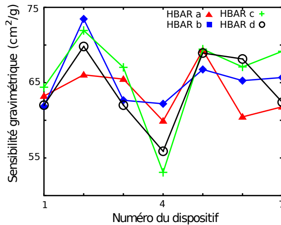
FIGURE 4.11 – Évolution de la sensibilité gravimétrique pour le premier dépôt en fonction des différents dispositifs pour quatre types de structure.
