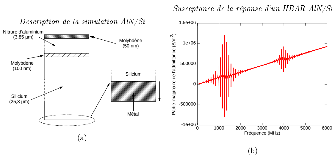
FIGURE 2.7 – Structure d'un résonateur HBAR à base d'AlN sur Si (a) et la partie imaginaire de l'admittance de la réponse d'un tel dispositif en fonction de la fréquence d'excitation (b).
