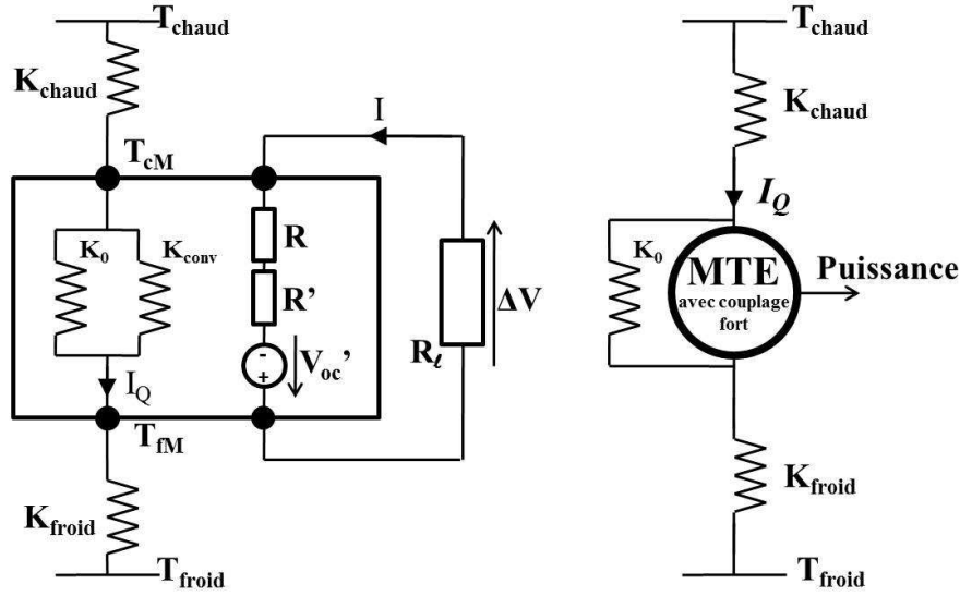
FIGURE 3.4 – Modélisation thermoélectrique (à gauche) et thermodynamique (à droite) de la machine thermoélectrique.
