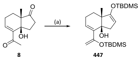
Schéma 119 : Synthèse du diénoles éthers silylé 447 . Réactifs et conditions : (a) TBDMSOTf, \text{Et}_3\text{N} , \text{CH}_2\text{Cl}_2 , TA, 1.5 h (100%).
