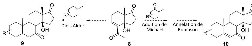
Schéma 4 : Chemins réactionnels envisagés.
