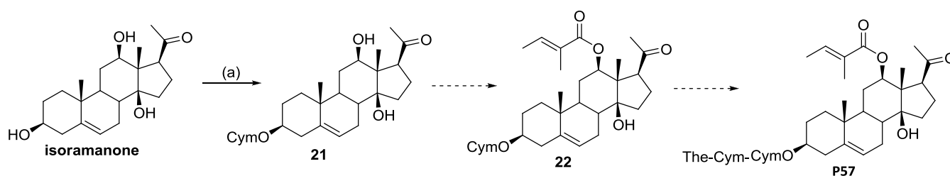
Schéma 7 : Vers la synthèse du P57. Réactifs et conditions: (a) SnCl 4 , Et 2 O, 3 jours, -15°C (15%).
