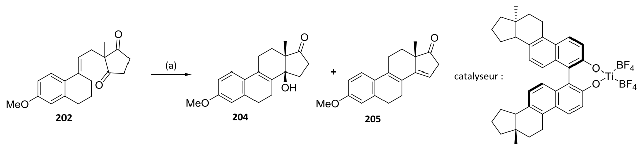
Schéma 72 : Cyclisation asymétrique. Réactifs et conditions : (a) catalyseur, tamis moléculaire (4 Å), \text{AgBF}_4 , toluène, -20^\circ\text{C} , 3 jours ( 204 : 20%, 36% ee; 205 : 72%, 70% ee).
