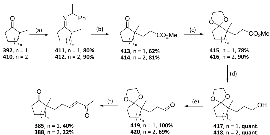
Schéma 112 : Synthèse des précurseurs 385 et 388 . Réactifs et conditions : (a) phényléthylamine, toluène, reflux, 15 h; (b) APTS, acrylate de méthyle, toluène, 50°C, 5 h; (c) tribromure de tétrabutylammonium, triméthyle orthoformate, éthylène glycol, 60°C, 15 h; (d) LAH, THF, TA, 10 min; (e) SO 3 .pyridine, Et 3 N, DMSO, CH 2 Cl 2 ; (f) i: Ph 3 P=CH 2 COMe, CH 2 Cl 2 , TA, 15 h; ii: HCl à 10%, THF, TA, 2.5 h.
