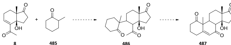
Schéma 141 : Démarche proposée pour accéder au tétracyclique 487
