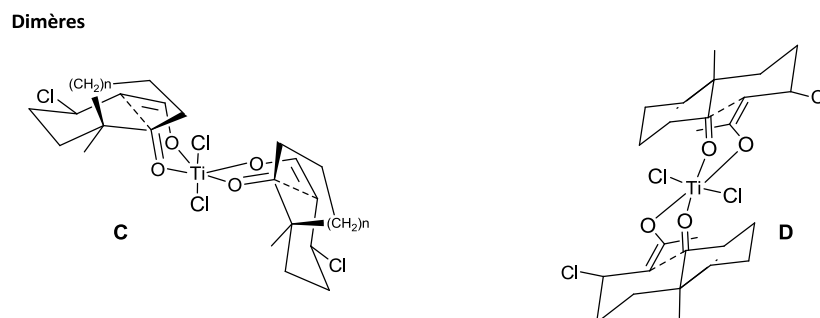
Schéma 115 : Intermediaires formés lorsque la réaction est effectuée avec 0.5 éq. de TiCl 4 .
