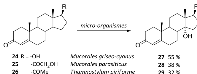
Schéma 10 : Monohydroxylation de stéroïde en position 14 en présence de micro-organisme.
