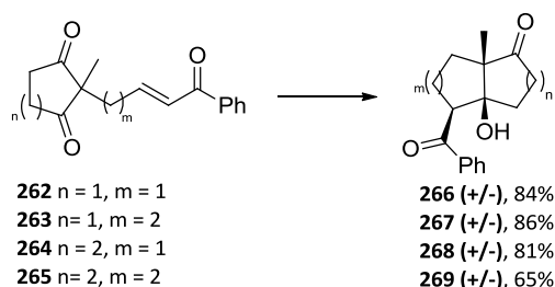
Schéma 84 : Cycloréduction de céto-énone. Réactifs et conditions : (a) Rh(COD) 2 OTf (10 mol%), PPh 3 (24 mol%), H 2 (1 atm), K 2 CO 3 (80 mol%), dichloroéthane, TA.
