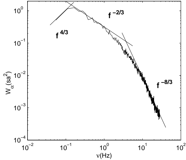
FIGURE 3.31 – Densité spectrale expérimentale des fluctuations d’AA. La fréquence de coupure f_c = 3.5Hz correspond à V = 20cm/s .
