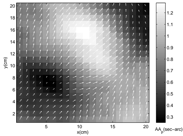
FIGURE 4.5 – Exemple d’un écran d’AA (en haut) et l’écran d’AA avec le filtrage de la pupille (en bas) de diamètre D = 10cm pour r_0 = 10cm , \lambda = 0.5\mu m et \mathcal{L}_0 = 20m
