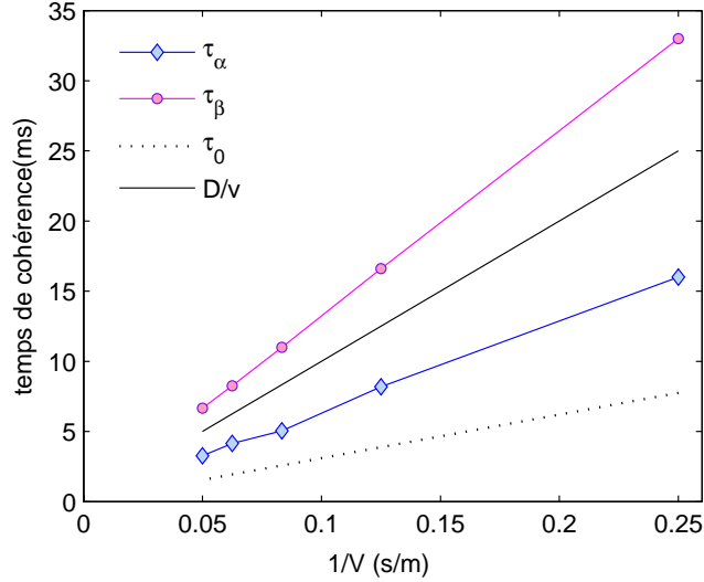
FIGURE 4.9 – \tau_\alpha dans les deux directions vs 1/V pour r_0 = D = 10\text{cm} , L_0 = 25\text{m} pour un coefficient de chute K = e , comparaison avec \tau_0 (Roddier) et D/V
