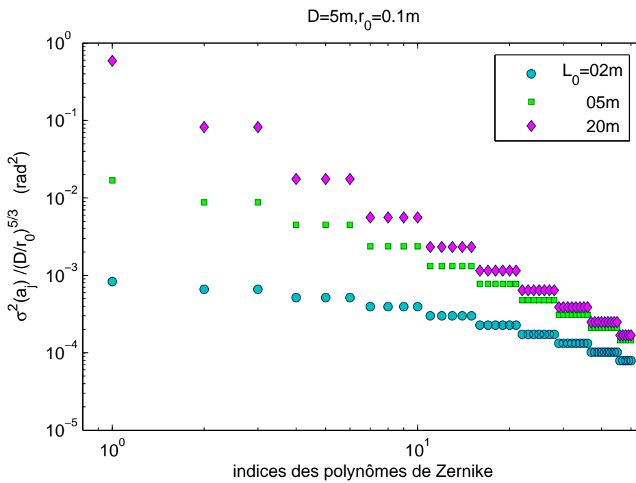
FIGURE 2.7 – Variance des coefficients des polynômes de Zernike normalisées par l'énergie de turbulence (D/r_0)^{5/3} pour D = 5m et pour un ordre croissant de valeurs d'échelle externe.
