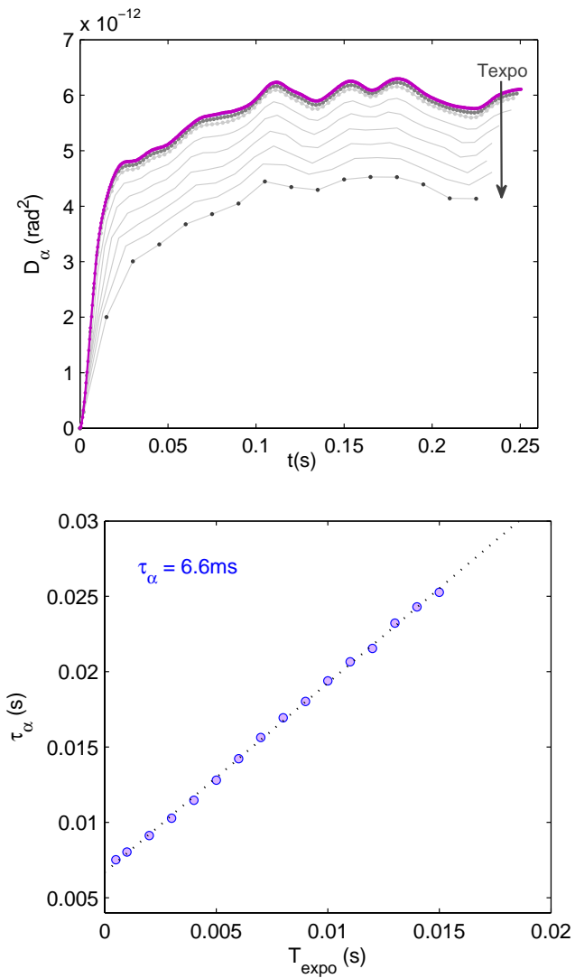
FIGURE 4.11 – Chute de la variance donnée par la hauteur de la fonction de structure à mesure que le temps de pose ( T_{\text{expo}} ) augmente (en haut). Détermination de \tau_\alpha = 6.6 \text{ms} par extrapolation de la droite à l'origine pour r_o = D = 10 \text{cm} , L_o = 25 \text{m} et V = 10 \text{m}
