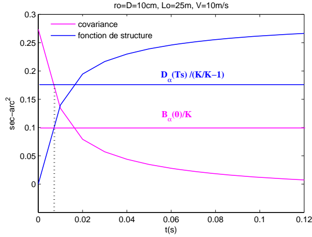
FIGURE 4.7 – La définition du \tau_\alpha à partir de la fonction de structure ou la covariance des fluctuations d'AA
