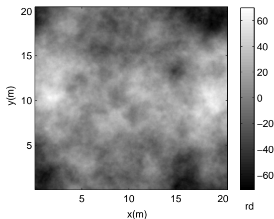
FIGURE 4.1 – Exemple d’un écran de phase obtenu par simulation numérique pour r_0 = 10cm et \mathcal{L}_0 = 20m .
