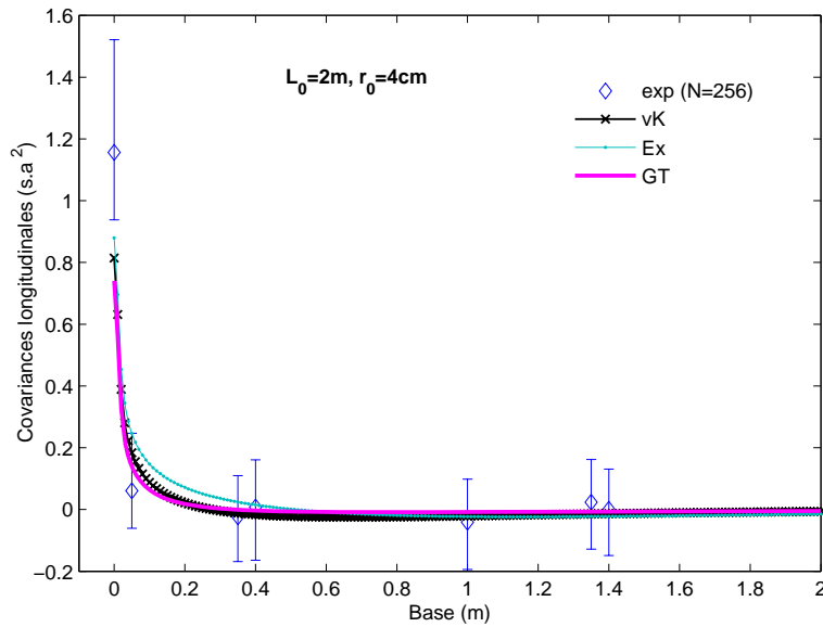
FIGURE 3.28 – La covariance expérimentale moyennée sur 256 mesures et l'ajustement par les covariances théoriques avec \mathcal{L}_0 = 2m et r_0 = 4cm .
