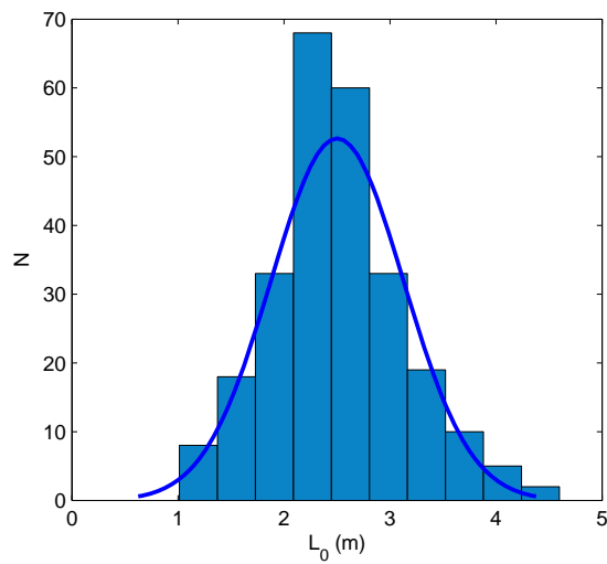
FIGURE 3.29 – Mesure de \mathcal{L}_0 par l'expérience LOTUCE au laboratoire mesurées toutes les 9 secondes en bleu et les valeurs moyennées toutes les minutes en noir (en haut). L'histogramme correspondant (en bas) pour les séries de mesures du 22 nov.2010 (forte turbulence). La valeur moyenne est \mathcal{L}_0 = 2,4m et \Delta\mathcal{L}_0 = 1,3m
