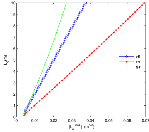
FIGURE 3.25 – Variation de la covariance normalisée intégrée sur toutes les bases L_{alpha}(D, \mathcal{L}_0) en fonction de \mathcal{L}_0 pour les différents modèles.
