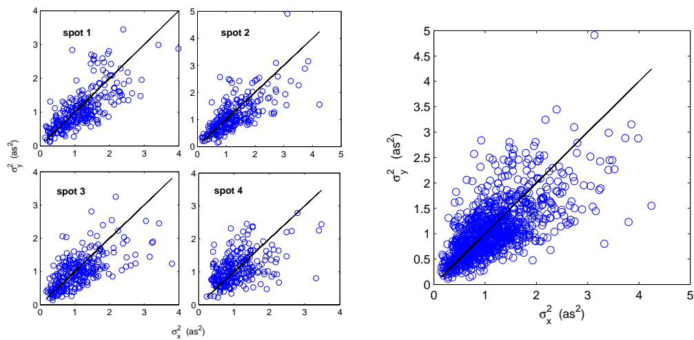
FIGURE 3.20 – Comparaison des variances dans les deux directions x et y pour les quatre voies (à gauche) avec coefficients de corrélation r > 0.72 et les mesures totales (à droite) pour les séries de mesures du 22 Nov. 2010 (forte turbulence)
