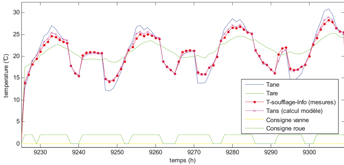
Figure 46. La validation du modèle de l'échangeur rotatif
