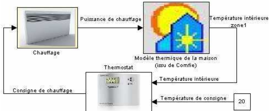
Figure 91. Schéma global de la simulation dans Simulink
