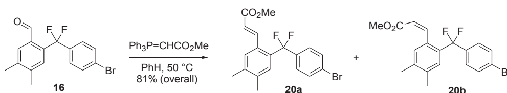
Schéma 17. Réaction de Wittig à partir de l'aldéhyde 16 .
