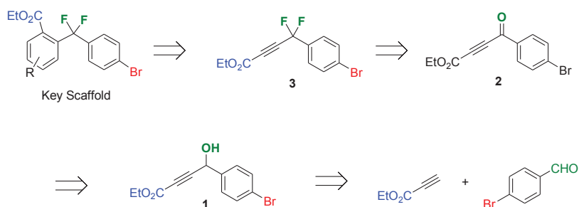
Schéma 4. Rétrosynthèse pour l'obtention du scaffold clé.
