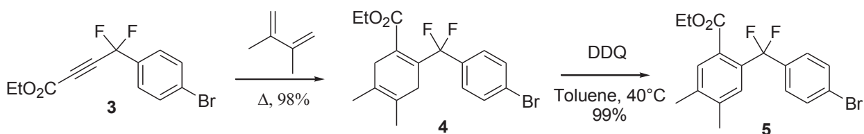
Schéma 6. Synthèse d'un exemple représentatif de scaffold clé, le composé 5 .
