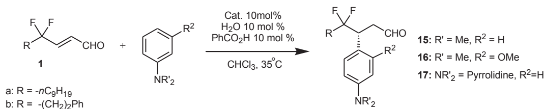
Schéma 20. Addition de différentes anilines aux énal 1.
