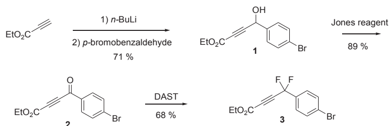
Schéma 5. Synthèse de l'intermédiaire 3 .
