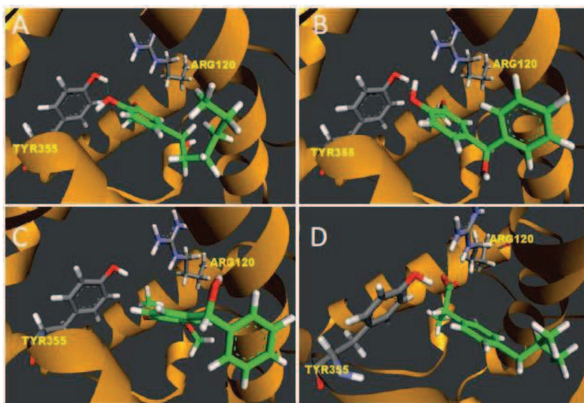
Figure 7B. Résultats de modélisation moléculaire sur les principales molécules étudiées.
