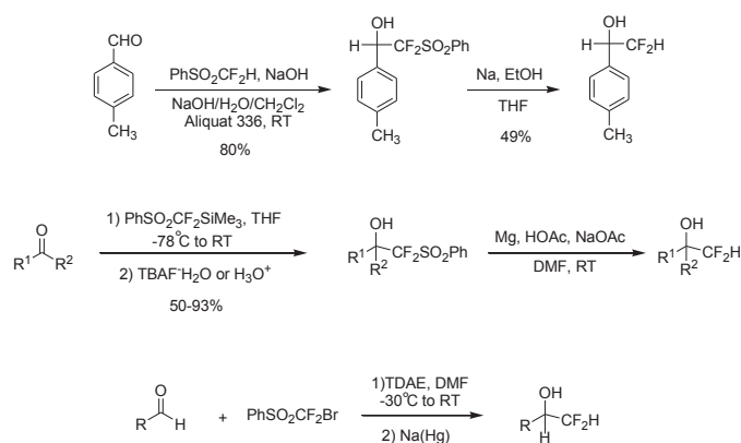
Schéma 16. Exemples représentatifs d'utilisation de \text{PhSO}_2\text{CF}_2\text{H} , \text{PhSO}_2\text{CF}_2\text{SiMe}_3 et \text{PhSO}_2\text{CF}_2\text{Br} .
