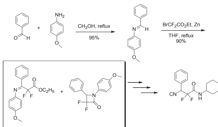
Schéma 13. Synthèse du N -cyclohexyl-2,2-difluoro-3-phenylpropanamide.
