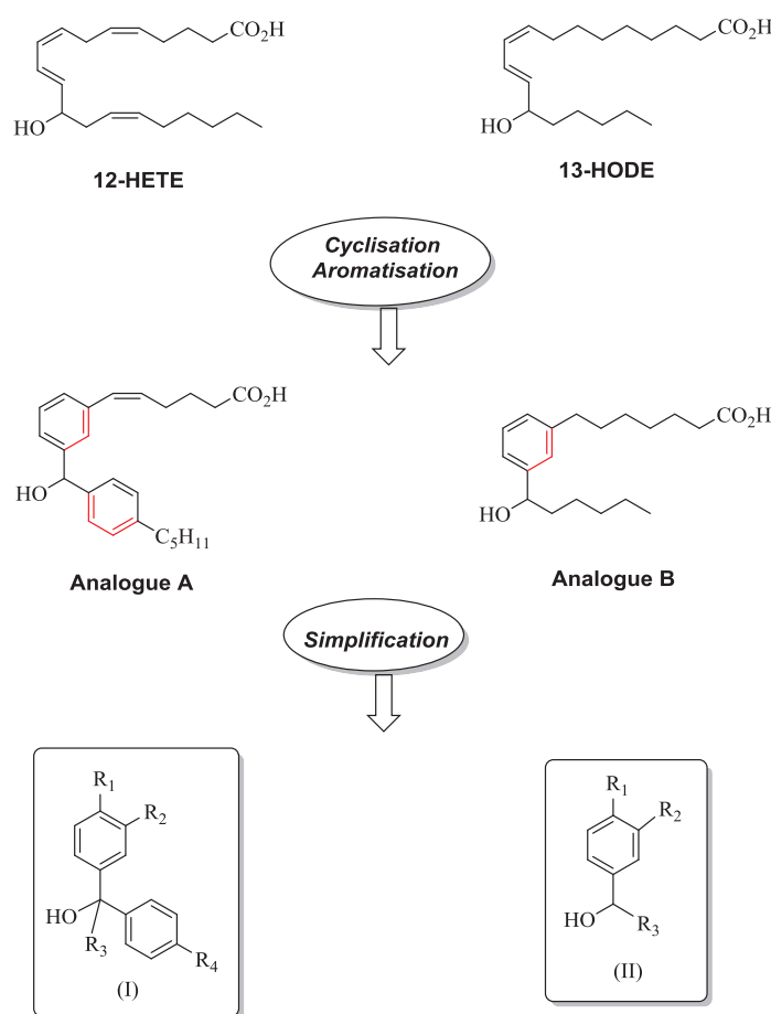
Schéma 1: Analogues simplifiés du 12-HETE et du 13-HODE
