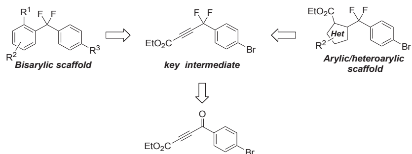
Schéma 3. Une nouvelle stratégie pour la synthèse de composés gem -difluorés bisaryliques et de dérivés mixtes aryl/hétéroaryliques.
