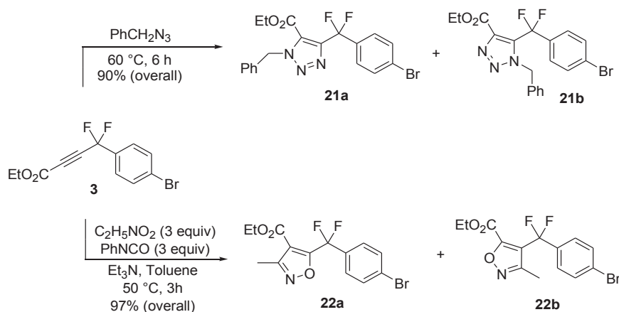
Schéma 18. Synthèse de dérivés mixtes aromatique-hétéroaromatique gem -difluorés 21 et 22 .
