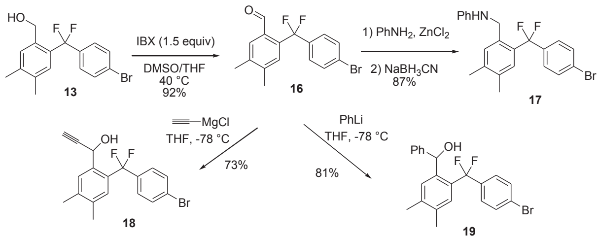
Schéma 14. Oxydation en aldéhyde puis utilisations de 16
