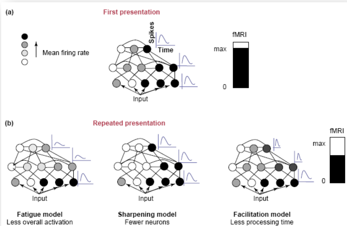
Figure 2.2 : Modèles explicatifs reliés à l'effet de RS. En haut à gauche : Décharge d'un neurone du cortex temporal du singe macaque en réponse à la présentation visuelle d'objets (décharges neuronales lors de la première présentation d'un objet, d'un nouveau stimulus et lors de la présentation répétée de l'objet). En haut à droite et en bas : Comparaison des trois modèles de l'effet de RS concernant les modifications de décharge neuronale et d'amplitude du signal BOLD après répétition d'un stimulus. Dans le modèle de fatigue, la réponse de l'ensemble de la population neuronale sensible au stimulus présentée diminue. Dans le modèle d'aiguisement, l'activité des neurones codant des traits non pertinents pour la reconnaissance du stimulus cesse, seuls les neurones pertinents maintiennent leur réponse. Dans le modèle de facilitation, la même population continue à décharger mais le temps de traitement (latence ou durée de la décharge) diminue (Figures empruntées à Grill-Spector, Henson et Martin, 2006).
