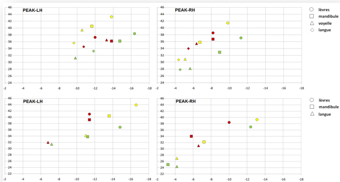
Figure D.3 : Projections des coordonnées Y et Z des pics d'activation maximale des articulateurs supralaryngés et vocaliques (en haut, étude 1.1, en bas, étude 2.1; les deux colonnes correspondent aux deux hémisphères). Une organisation somatotopique est observée, impliquant une position plus postérieure des lèvres par rapport à la langue dans la dimension rostro-caudale (Y) et une position plus dorsale des lèvres par rapport à la langue et la vocalisation ainsi que pour la mandibule par rapport à la langue dans l'axe dorso-ventral (Z).
