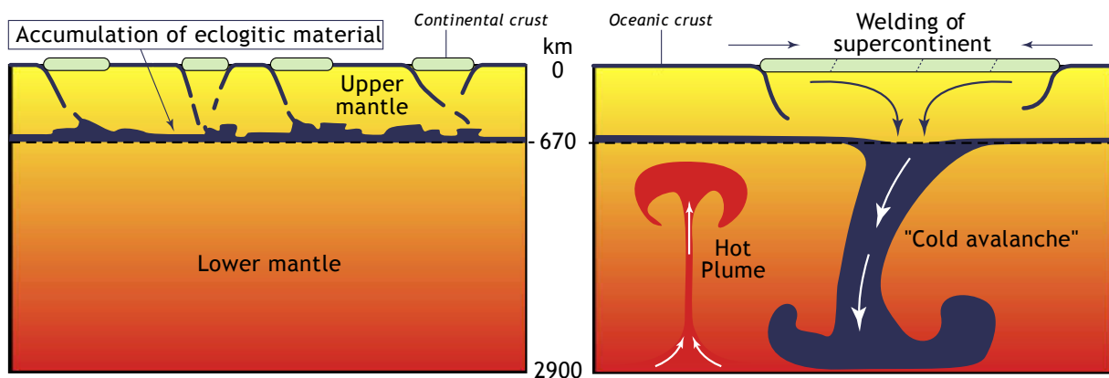
FIGURE 1.20 : Le modèle d'« avalanche froide » : pendant la première phase (à gauche), du matériel éclogitique dense ( d > 3.3 ) est subduit et s'accumule à la transition de phase de 670 km (base du manteau supérieur). Passé un certain seuil, ce matériel « coule » dans le manteau inférieur au cours de la seconde phase (à droite), provoquant l'assemblage d'un supercontinent en surface et, en profondeur, une instabilité qui génère la remontée de panaches mantelliques chauds. D'après les modèles de Stein & Hofmann (1994), Davies (1995), Condie (1998) et Yale & Carpenter (1998).
