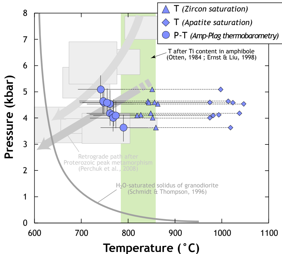
FIGURE 4.8 : Diagramme P–T dans lequel ont été reportées les conditions de cristallisation calculées à partir de différents thermomètres et thermobaromètres pour 10 échantillons du pluton de Bulai. Les champs et les flèches en grisé représentent des estimations P–T obtenues sur la base de l'étude des granulites de la Zone Centrale (voir Figure 3.27).
