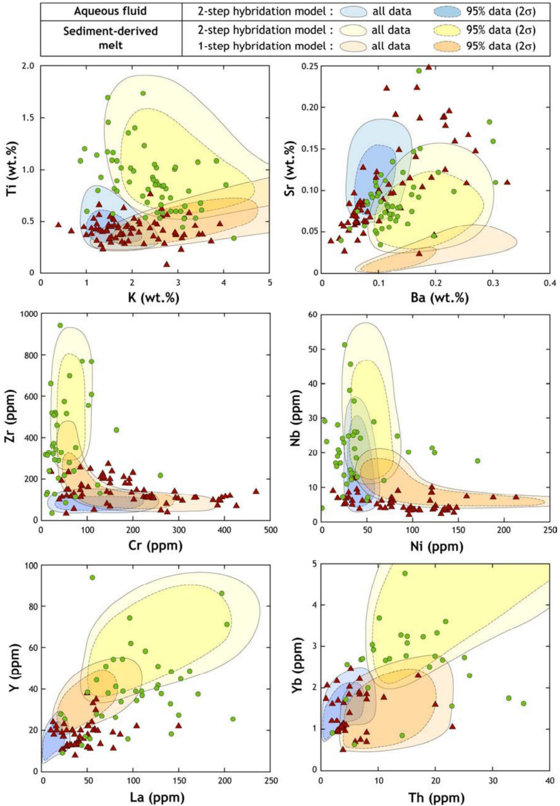
FIGURE 4.12 : Diagrammes binaires identiques à ceux de la Figure 4.10, où la composition des liquides virtuels correspond à une modélisation en utilisant des agents métasomatiques différents des TTT : un fluide aqueux (bleu) et un liquide issu de la fusion de sédiments (orange, jaune). Les symboles sont identiques à ceux de la Figure 4.10.
