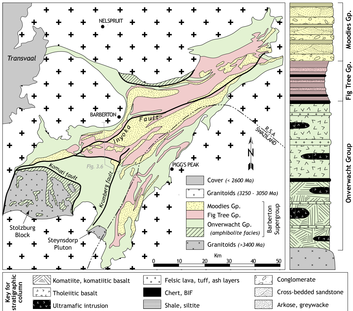
FIGURE 3.5 : Carte géologique et log stratigraphique schématique de la ceinture de roches vertes de Barberton (d'après Brandl et al., 2006). La ligne en grisé correspond à la position de la coupe de la Figure 3.6.
