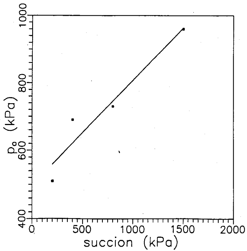
Figure VIII-6 : Relation entre p_0 et la suction
