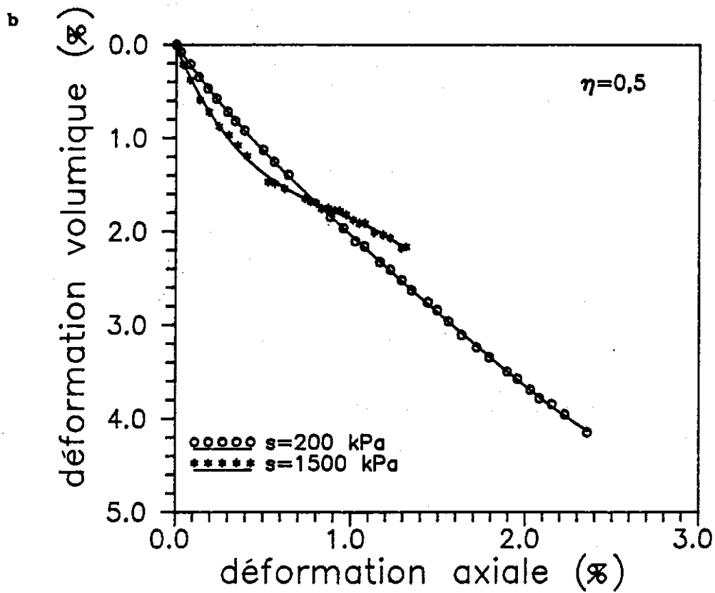
Figure VI-28 : Courbes des essais à \eta = 0,5
