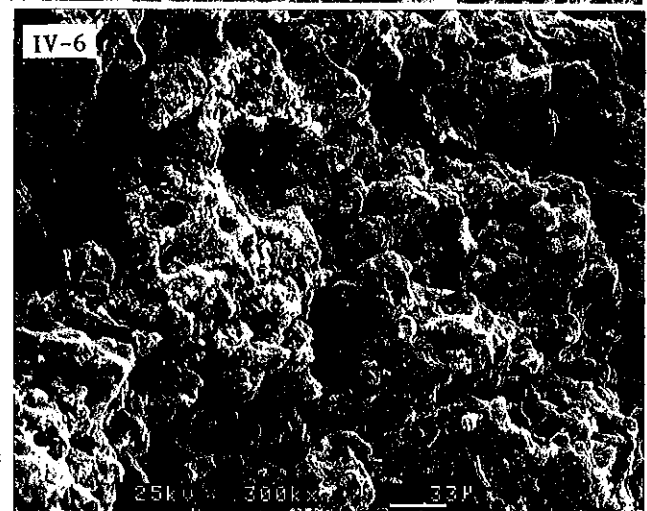
Photos en microscopie électronique à balayage du limon compacté IV-1, IV-2 et IV-3 : côté sec (Psec) IV-4 et IV-5 : côté humide (Hum) IV-6 et IV-7 : Optimum (Nat)
