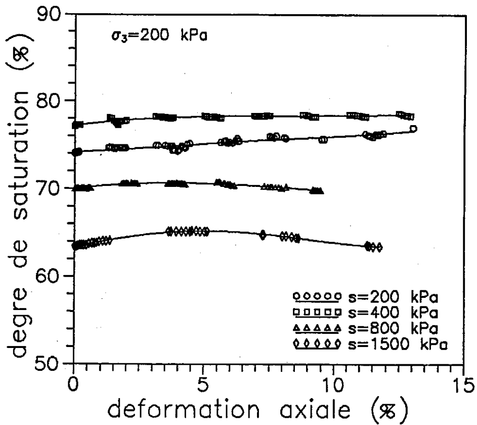
Figure 1-3 : Variations d'échange d'eau et de degré de saturation lors du cisaillement sous \sigma_3 = 200 \text{ kPa}
