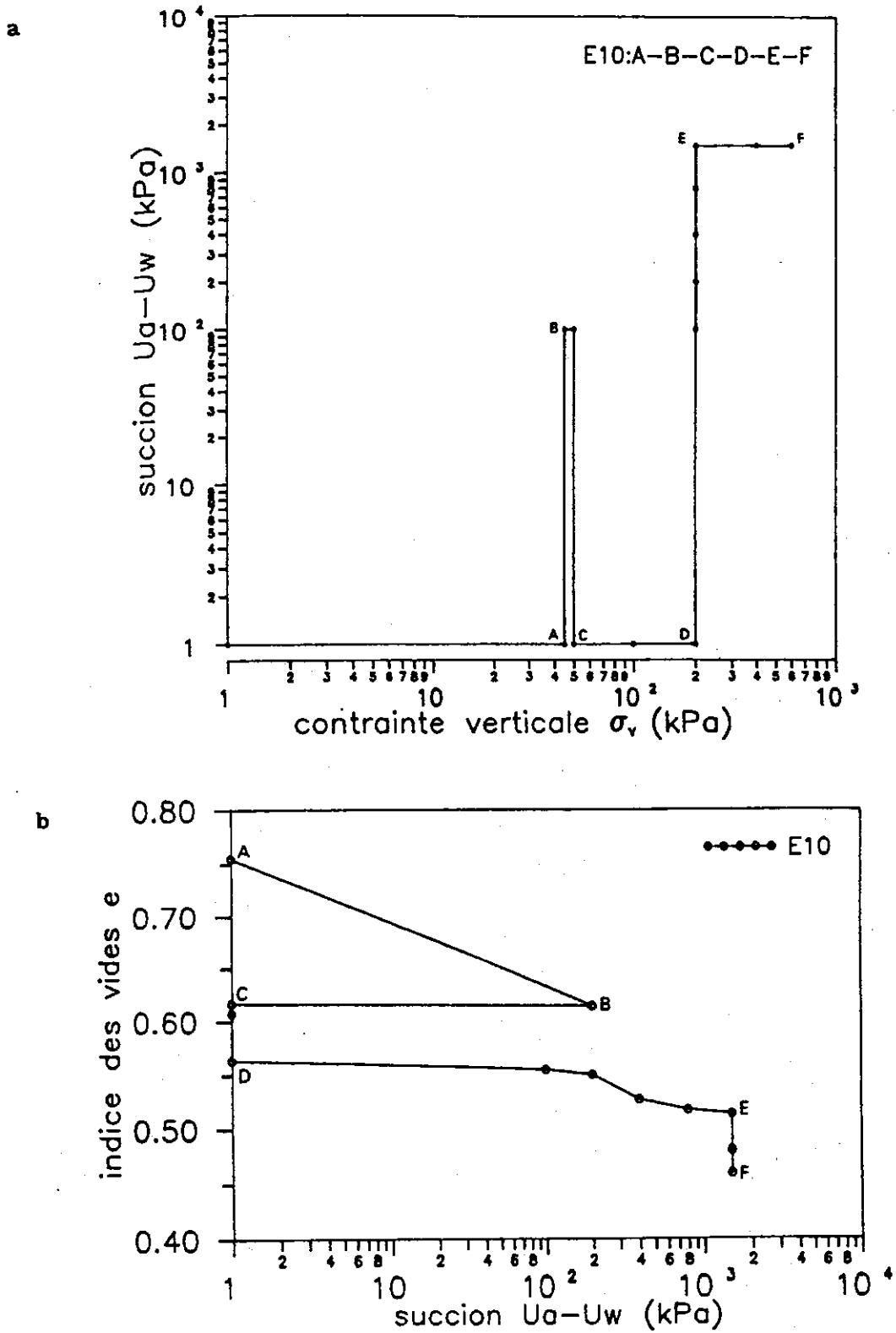
Figure IV-7 : Variation de volume en fonction de la succion a) chemin de contraintes b) réponse en volume (Vicol 1990)
