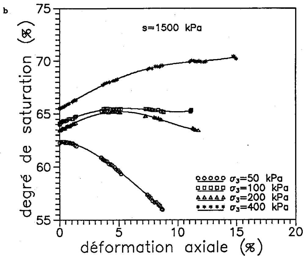
Figure VI-23 : Evolutions de l'échange d'eau et du degré de saturation lors des essais de cisaillement à s = 1500 kPa
