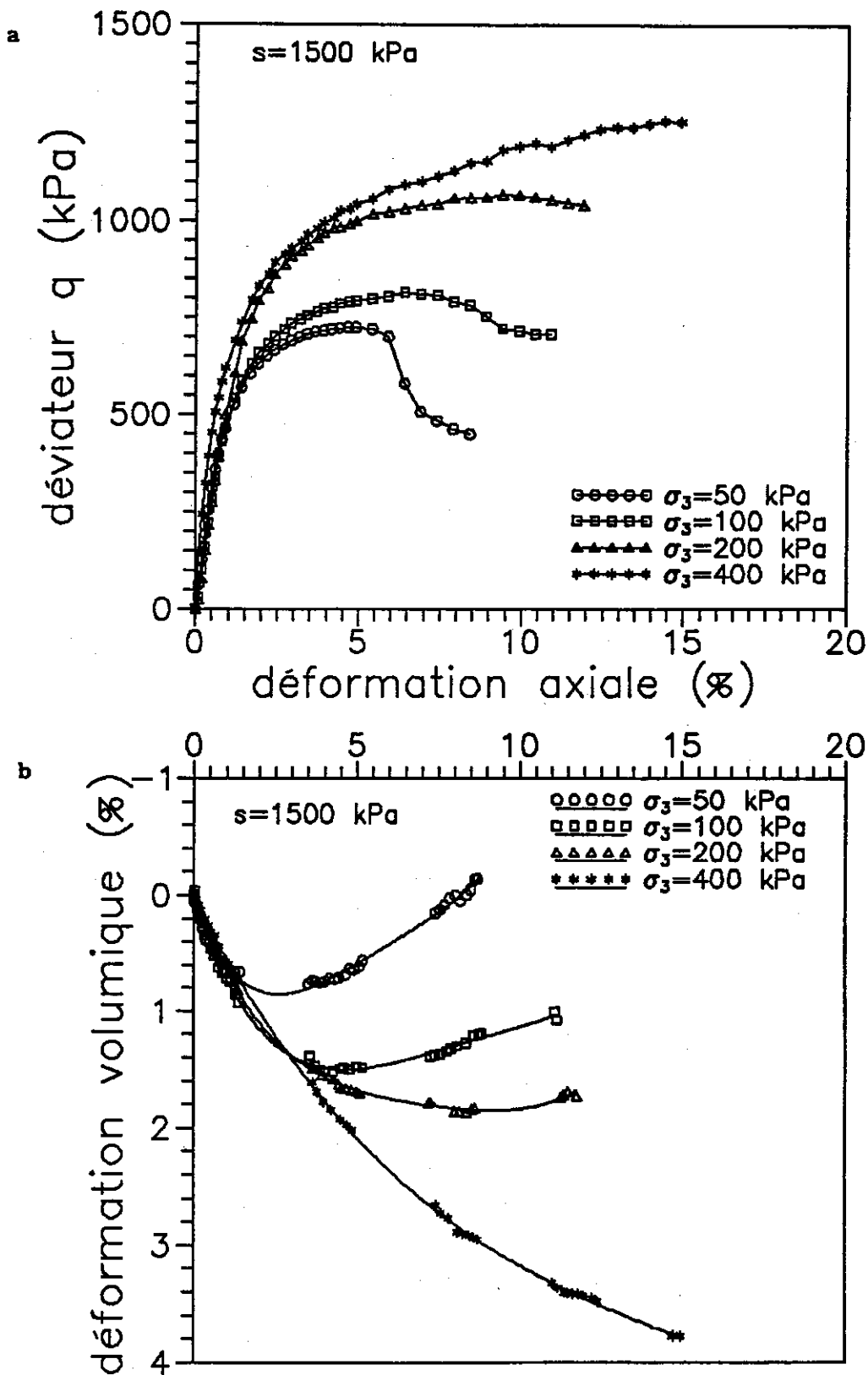
Figure VI-18 : Courbes de cisaillement à s = 1500 kPa
