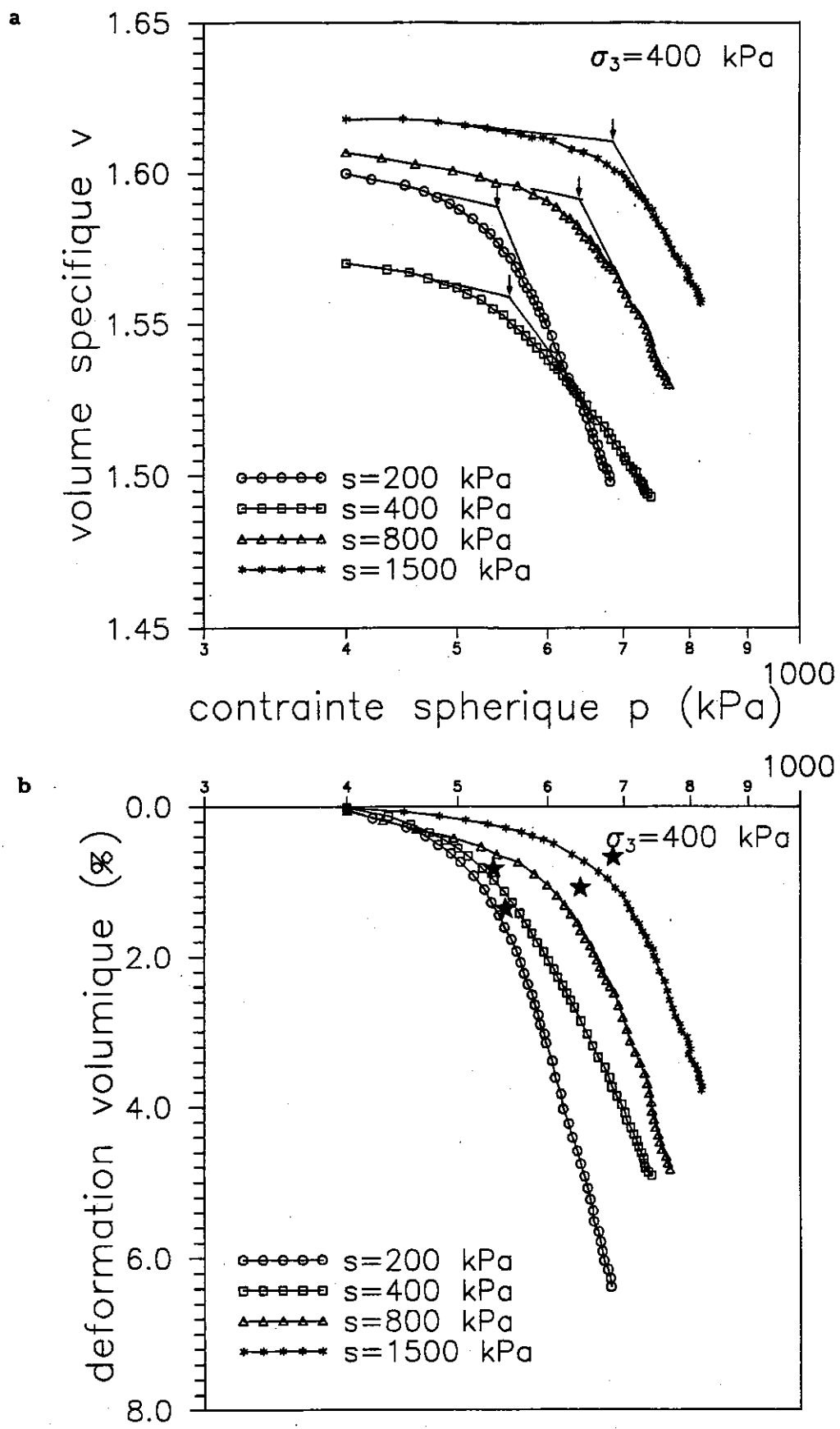
Figure VII-5 : Variations volumiques lors des essais de cisaillement à \sigma_3 = 400 \text{ kPa} a) dans le plan v -log p b) dans le plan d\varepsilon_v -log p
