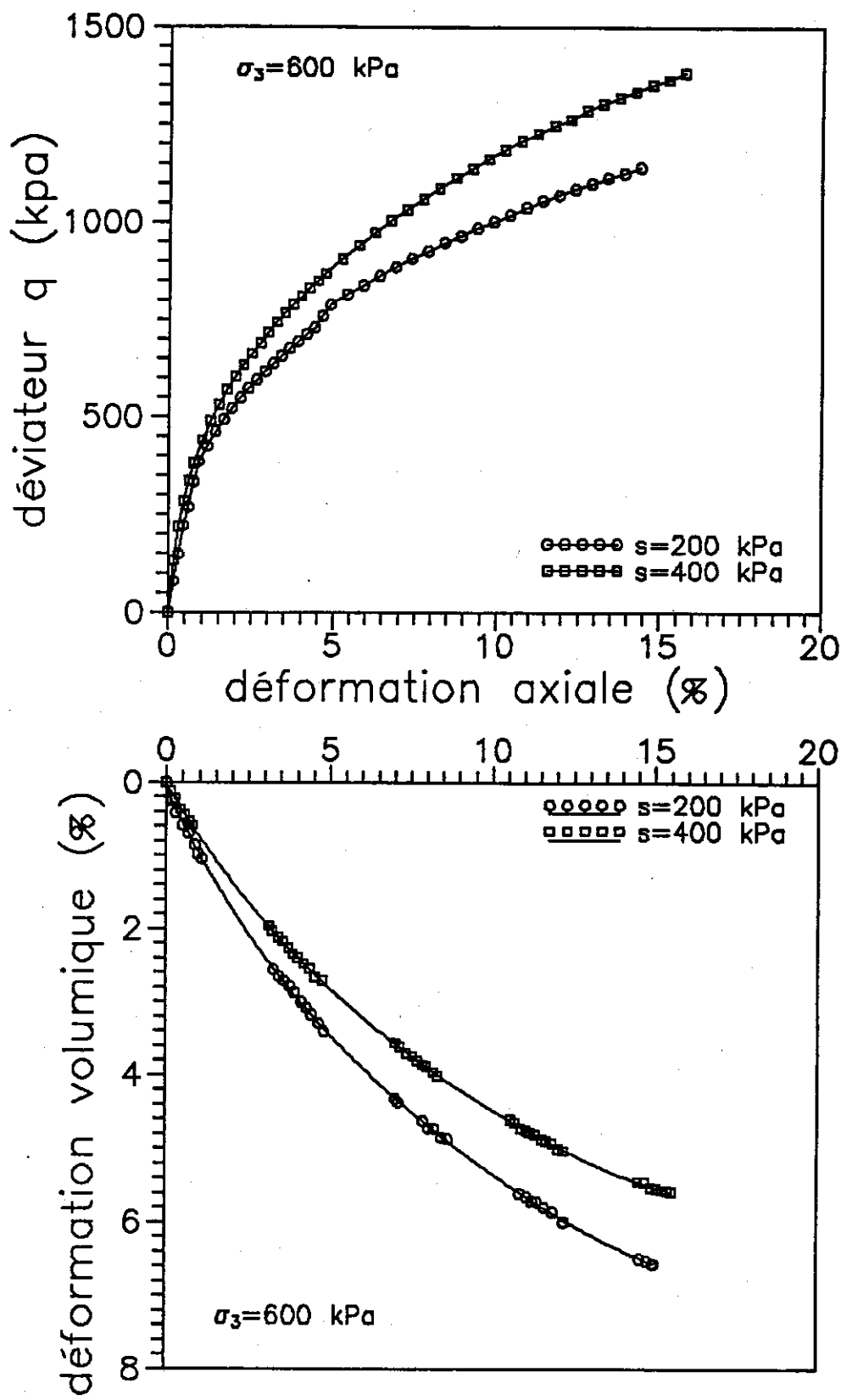
Figure VI-16 : Courbes de cisaillement à \sigma_3 = 600 \text{ kPa} a) effort-déformation b) variations volumiques
