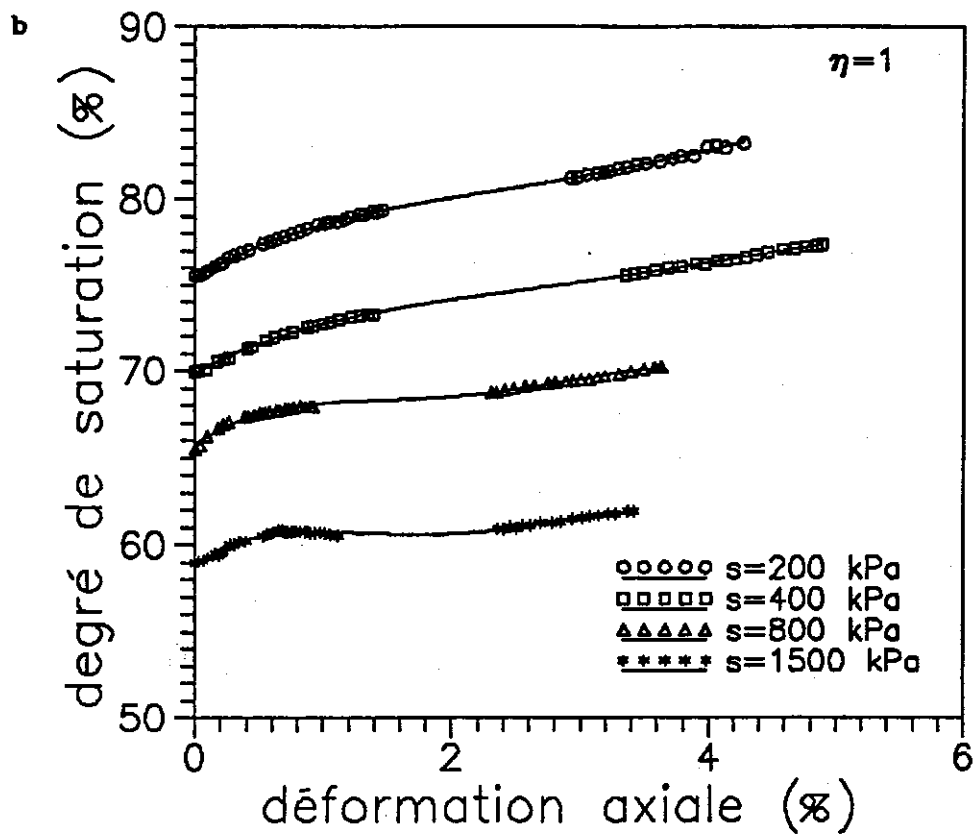
Figure VI-31 : Evolutions de l'échange d'eau et du degré de saturation lors des essais à \eta = 1
