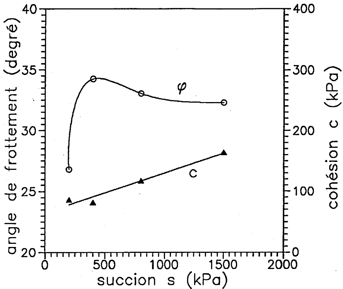
Figure VI-27 : Variations de l'angle de frottement et de la cohésion en fonction de la suction
