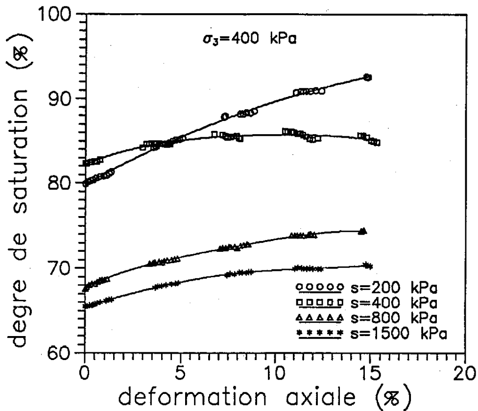
Figure 1-4 : Variations d'échange d'eau et de degré de saturation lors du cisaillement sous \sigma_3 = 400 kPa
