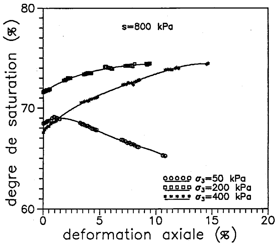
Figure 1-7 : Variations d'échange d'eau et de degré de saturation lors du cisaillement à s = 800 kPa
