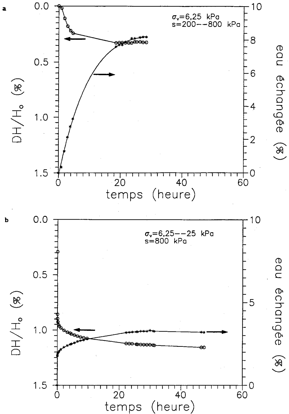
Figure VI-4 : Evolutions de la déformation axiale et de l'échange d'eau a) lors de l'augmentation de suction de 200 à 800 kPa b) lors du chargement de 6,25 à 25 kPa
