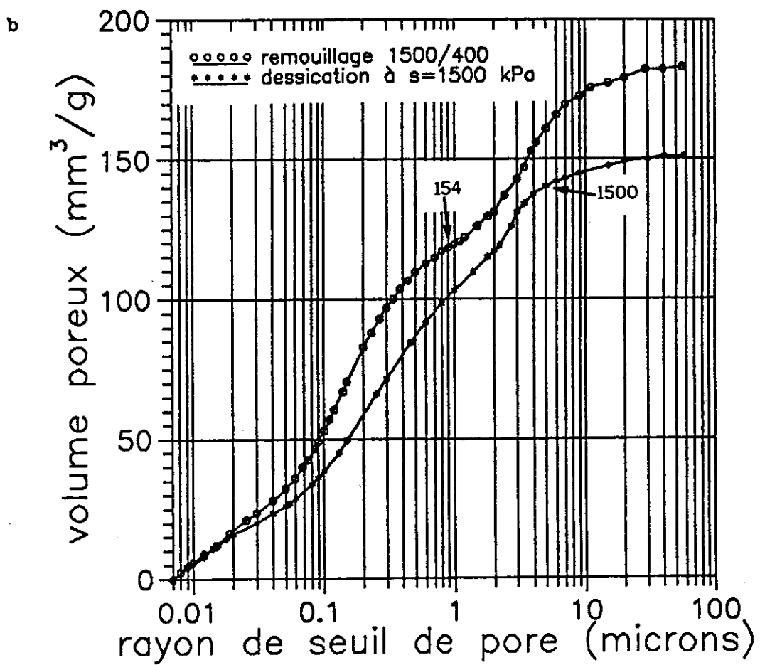
Figure IV-8 : Courbes porosimétriques
