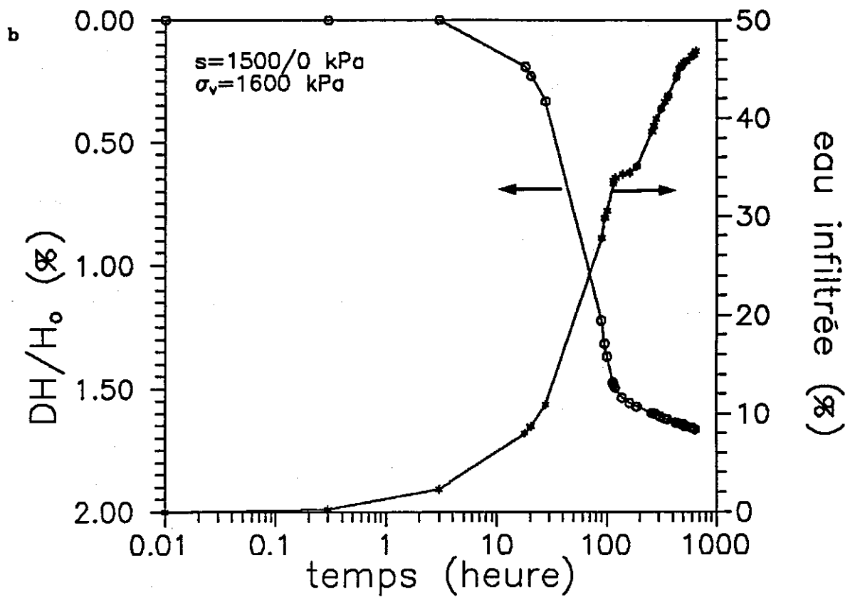
Figure VI-9 : Evolutions de la déformation axiale et de l'eau infiltrée lors des essais de remouillage a) succion initiale égale à 800 kPa b) succion initiale égale à 1500 kPa
