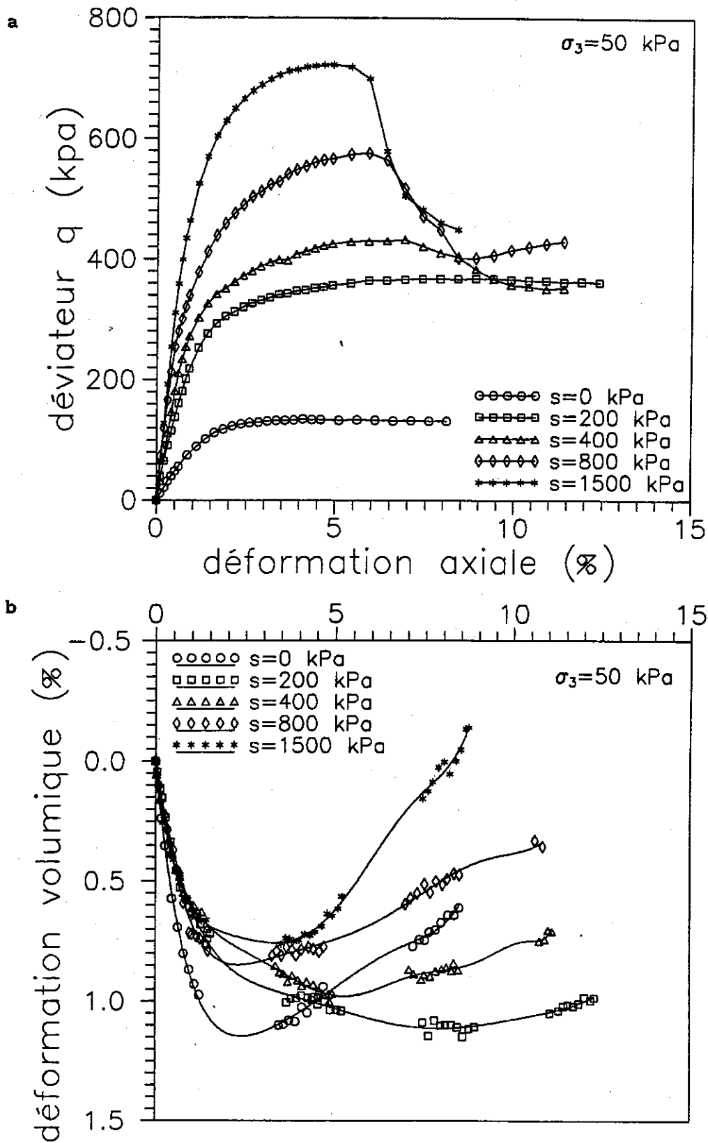
Figure VI-12 : Courbes de cisaillement à \sigma_3 = 50 \text{ kPa}
