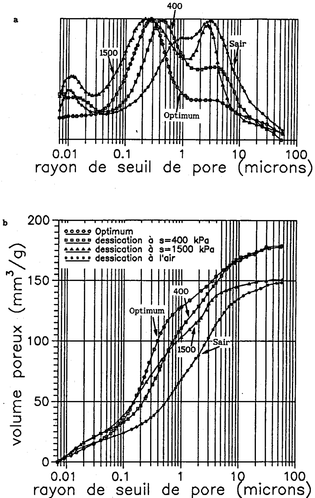
Figure IV-5 : Effet de la dessiccation sur les courbes porisimétriques a) courbes dérivées b) courbes cumulées
