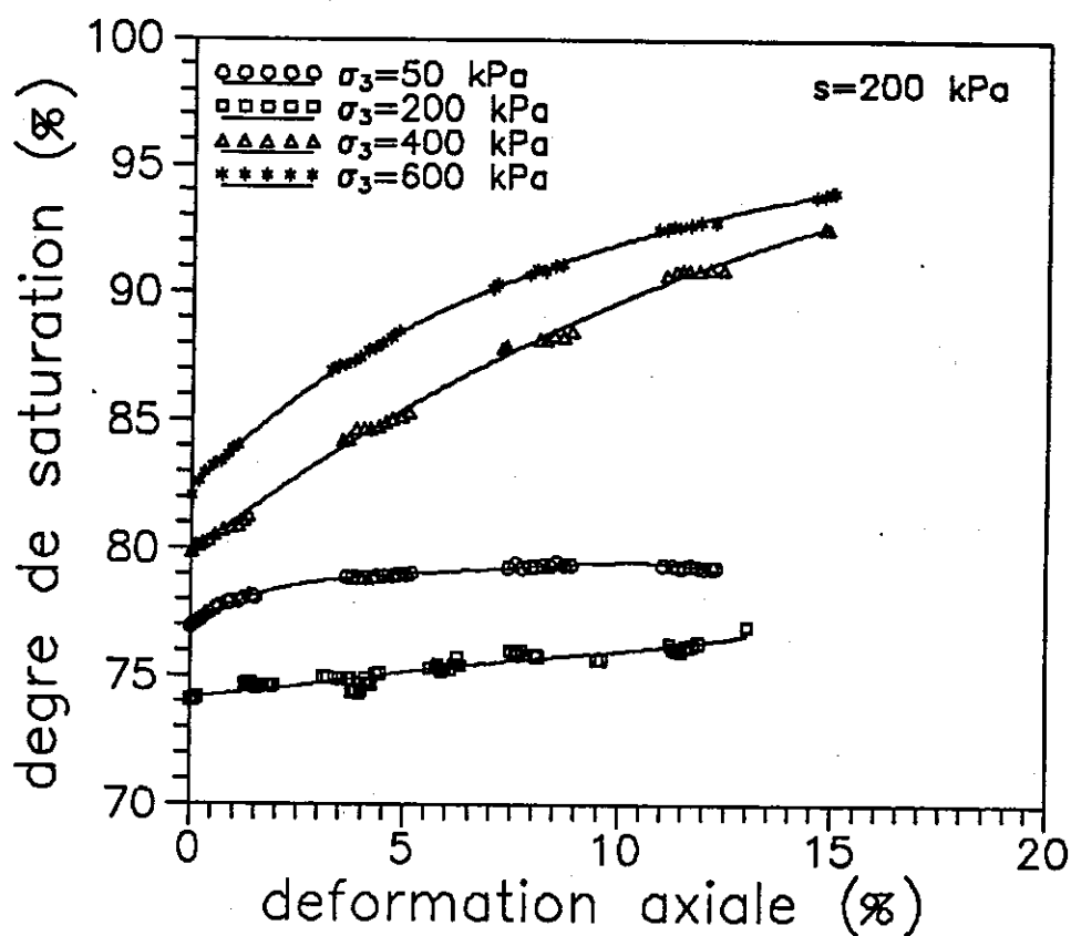
Figure 1-5 : Variations d'échange d'eau et de degré de saturation lors du cisaillement à s = 200 \text{ kPa}
