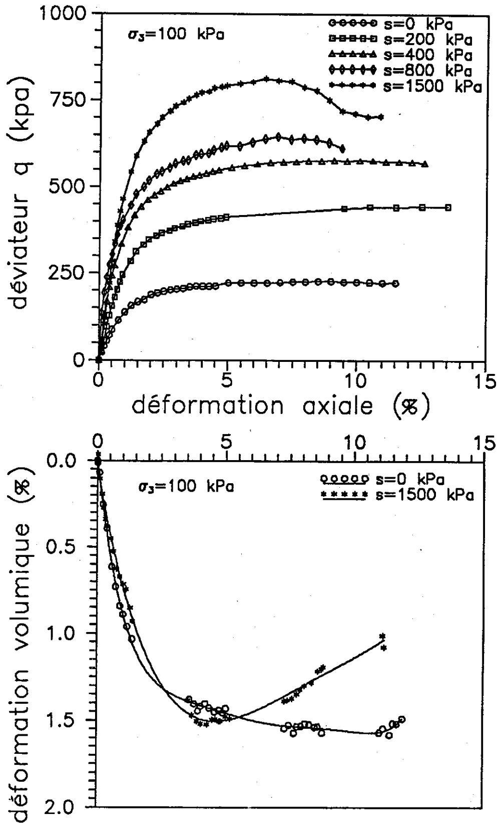
Figure VI-13 : Courbes de cisaillement à \sigma_3 = 100 \text{ kPa} a) effort-déformation b) variations volumiques
