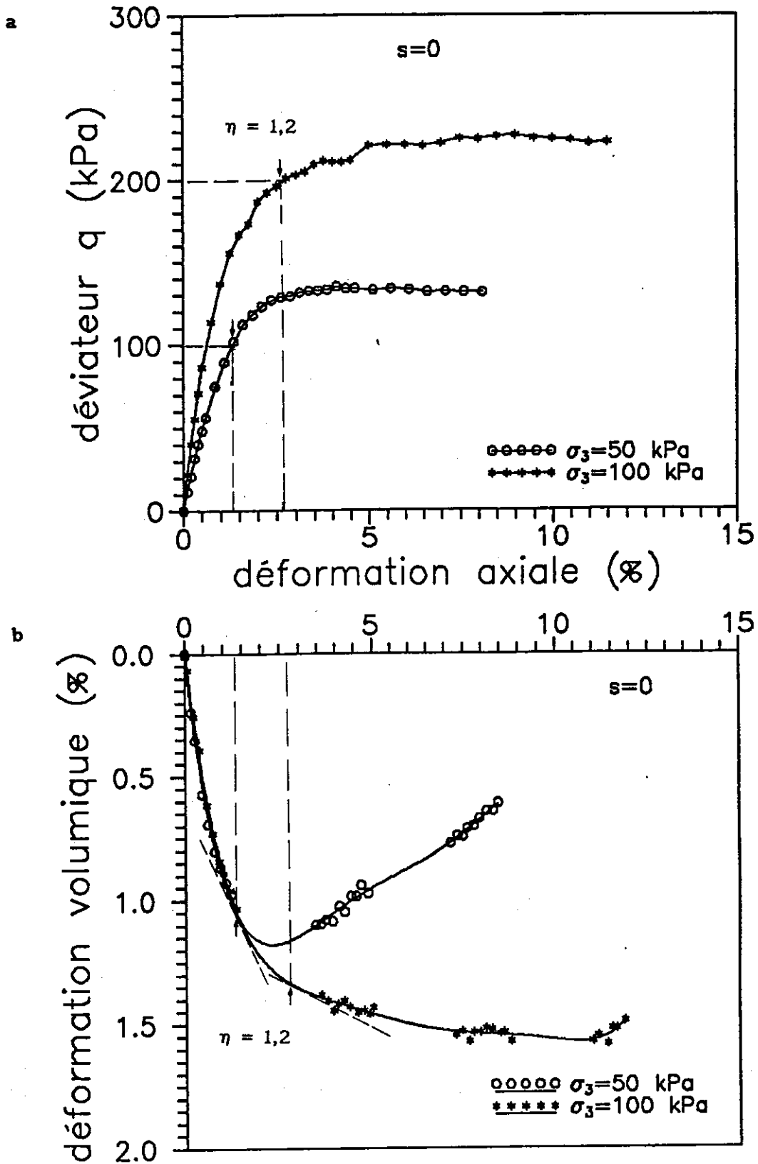
Figure VII-21 : Courbes de cisaillement à succion nulle a) effort-déformation b) variations volumiques
