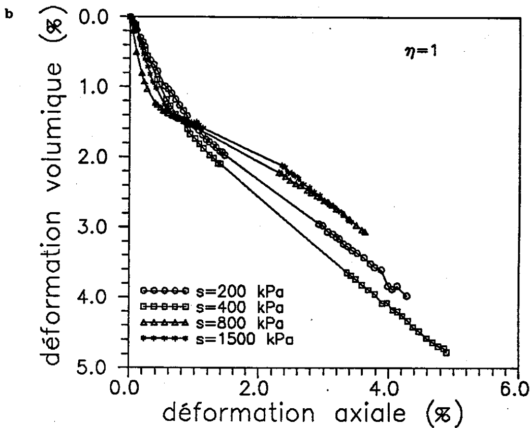
Figure VI-29 : Courbes des essais à \eta = 1
