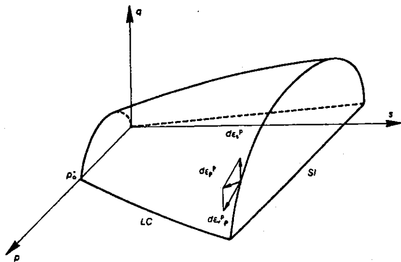
Figure VIII-4 : Surfaces de charge dans l'espace p-q-s (Alonso et al. 1990)
