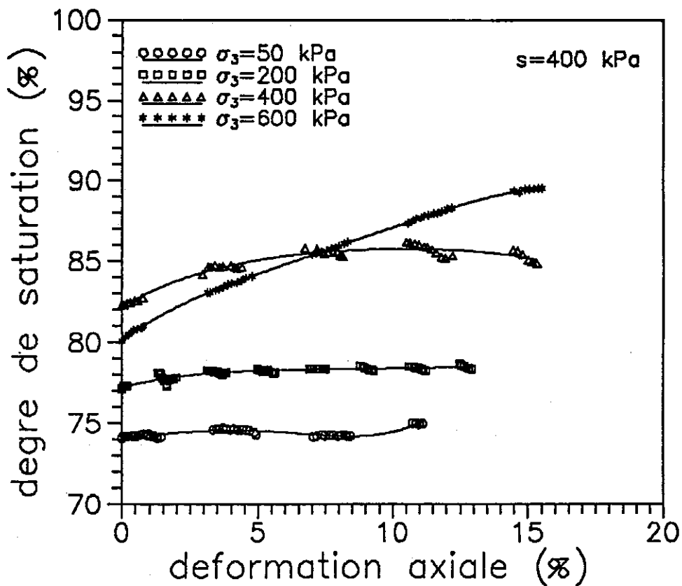
Figure 1-6 : Variations d'échange d'eau et de degré de saturation lors du cisaillement à s = 400 kPa
