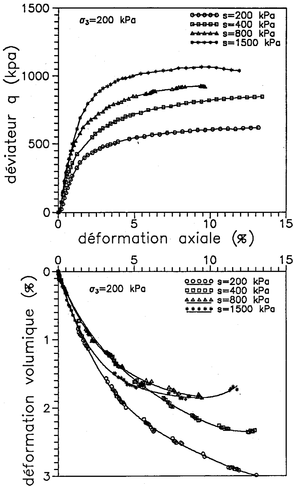
Figure VI-14 : Courbes de cisaillement à \sigma_3 = 200 kPa a) effort-déformation b) variations volumiques
