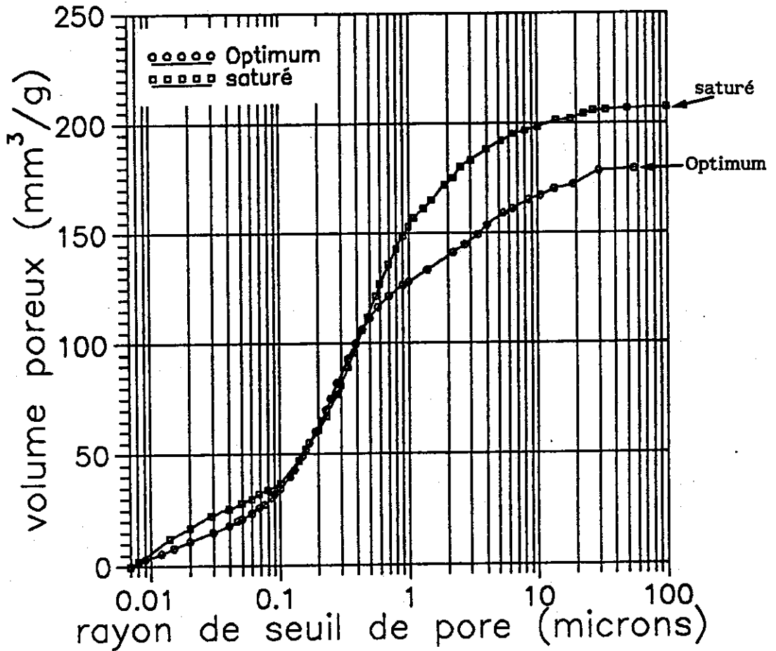
Figure IV-2 : Courbes porosimétriques
