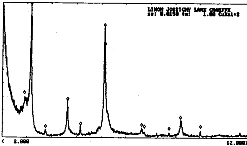
Spectres diffractométriques des trois lames du limon de Jossigny (Lapeyre 1992)
