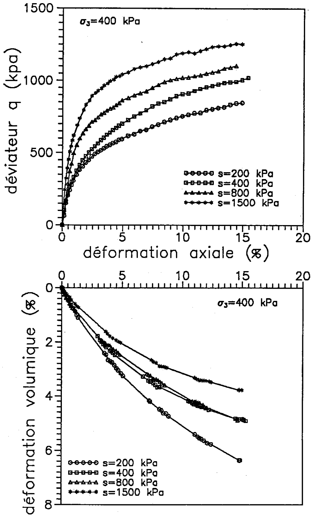
Figure VI-15 : Courbes de cisaillement à \sigma_3 = 400 \text{ kPa} a) effort-déformation b) variations volumiques
