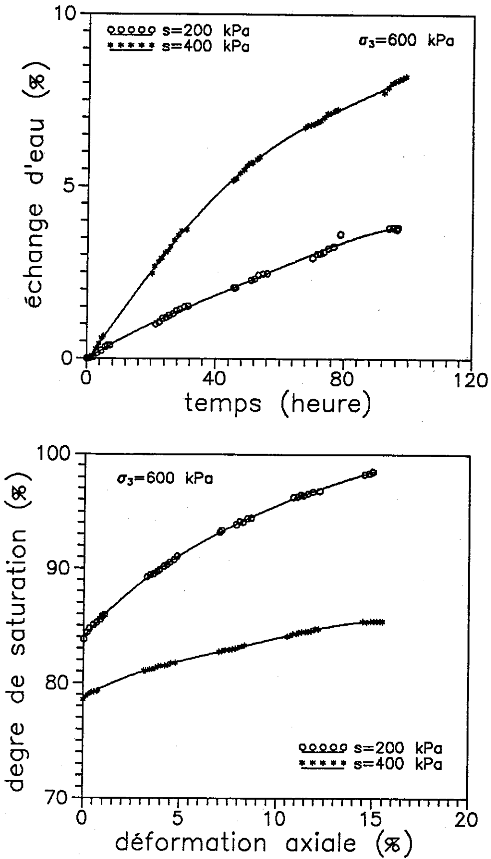
Figure VI-22 : Evolutions de l'échange d'eau et du degré de saturation lors des essais de cisaillement à \sigma_3 = 600 \text{ kPa}
