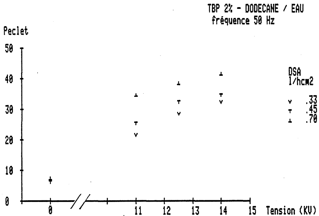
Figure VI-14 : Nombre de Peclet à divers débits en fonction de la tension
