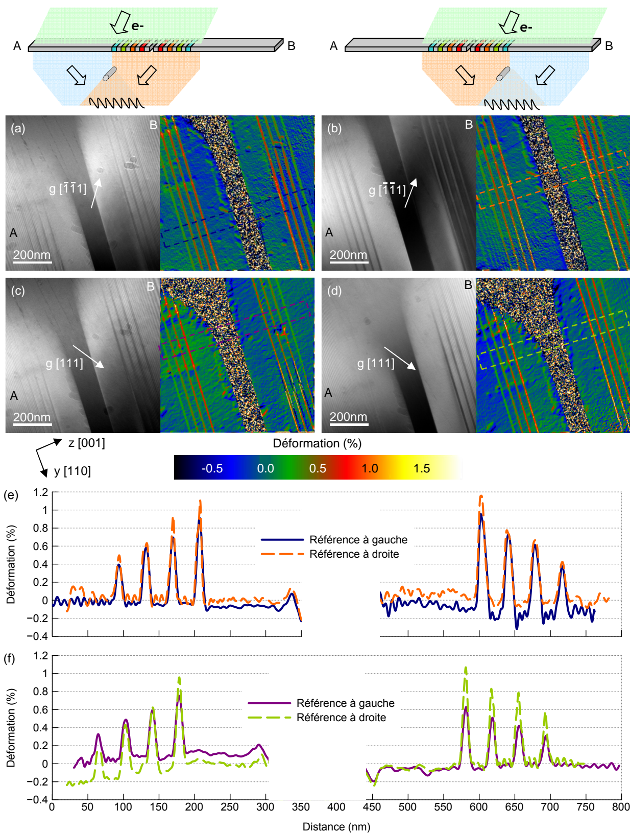
FIGURE IV.13 – Expérience réalisée sur un échantillon préparé par polissage en sandwich et possédant 4 couches de SiGe avec des concentrations de 45%, 38%, 31% et 20% de Ge. (a-d) Hologrammes en champ sombre et cartes de déformation obtenus à partir des réflexions (\bar{1}\bar{1}1) pour les cas (a,b) et (111) pour les cas (c,d). L'interférence est créée avec le substrat de gauche dans les cas (a,c) et le substrat de droite dans les cas (b,d). Les cartes représentent la déformation calculée dans la direction définie par le vecteur \vec{g} dessiné sur l'hologramme. (e,f) Profils de déformation extraits des cartes (a,b) et (c,d) respectivement, comme indiqué par des cadres pointillés. Les profils ont été moyennés sur 80 nm dans la direction y [110] .
