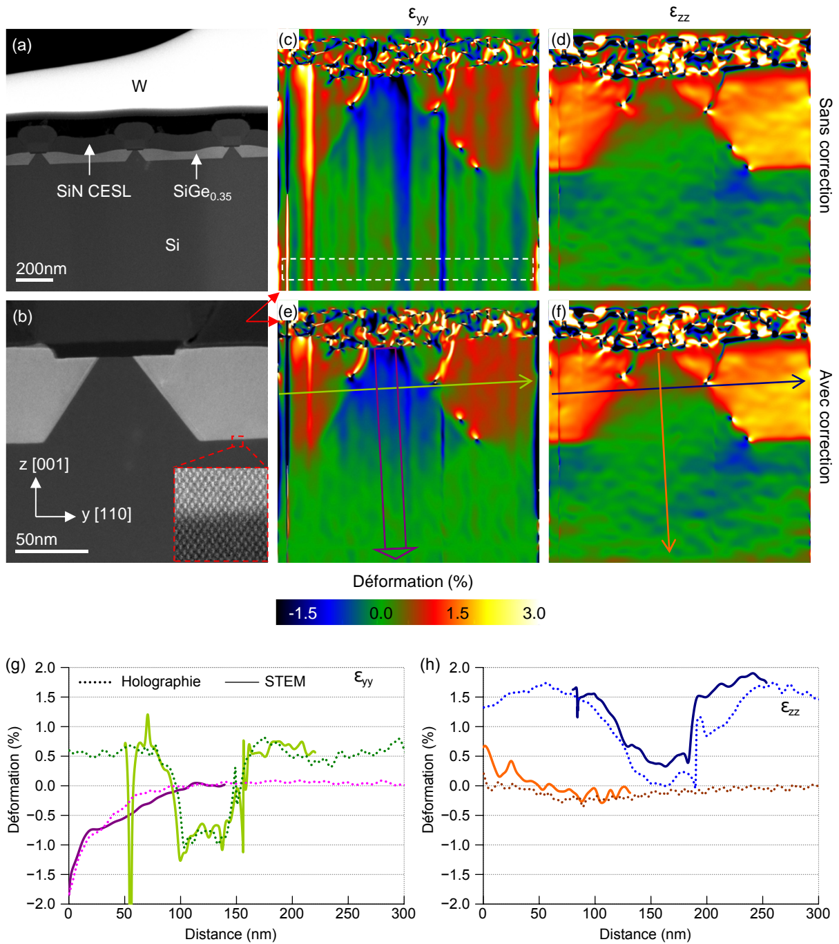
FIGURE VI.5 – (a) Image STEM-HAADF à faible grandissement de l'échantillon non siliciuré possédant un film stresser de SiN, ainsi que des sources/drains de Si 0,65 Ge 0,35 :B. (b) Image STEM-HAADF haute résolution d'un des dispositifs. La direction de scan est la direction z [001]. (c,d) Cartes de déformation \epsilon_{yy} et \epsilon_{zz} reconstruites par analyse des phases géométriques. Un masque gaussien de rayon 3\sigma = 0,17 \text{ nm}^{-1} a été utilisé dans l'espace de Fourier. Deux réflexions de type {111} ont été sélectionnées de façon à reconstruire le tenseur 2D des déformations. (e,f) Cartes de déformation obtenues en effectuant une correction supplémentaire consistant à soustraire le profil de phase du substrat (dans la région encadrée par un trait blanc pointillé) à l'ensemble de l'image. (g,h) Profils de déformation extraits des cartes (e,f) suivant les flèches. Les profils de déformation obtenus par holographie sont également reportés en pointillés.
