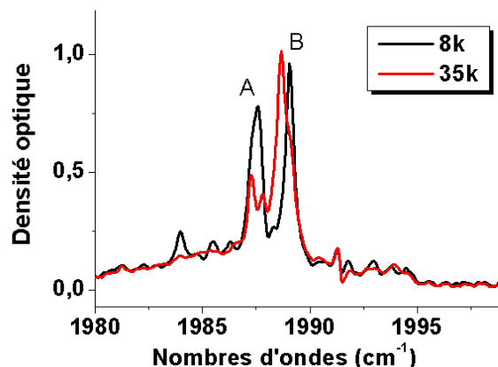
FIGURE 4.31 – Spectres d'absorption de W(CO)_6 en matrice de CF_4 à 8 et 35 K. - Le spectre est constitué de deux bandes A ( 1987,5 \text{ cm}^{-1} ) et B ( 1988,7 \text{ cm}^{-1} ) larges de \approx 1 \text{ cm}^{-1} reposant sur un piédestal large de \approx 7 \text{ cm}^{-1} .
