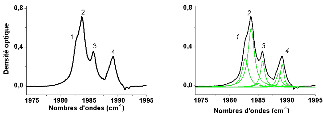
FIGURE 4.3 – Spectre d'absorption infrarouge de W(CO)_6 en matrice d'azote à 20 K. - A droite : ajustement des bandes 1 et 2 par des Lorentziennes ; ajustement des bandes 3 et 4 par trois Lorentziennes.
