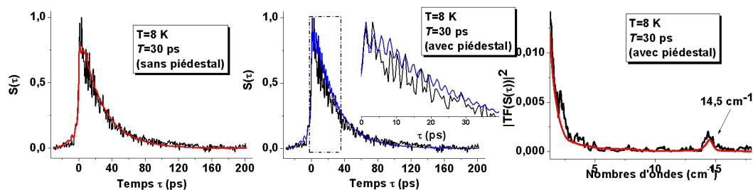
FIGURE 4.21 – Signal d'écho de photons stimulé de W(CO)_6/CH_4 à 8 K. - Pour ce signal, T=30 ps. Le signal expérimental est en noir, le modèle est en rouge. A gauche, le signal est modélisé (en rouge) sans considérer le piédestal. Au milieu, nous avons rajouté la contribution du piédestal (en bleu). A droite : module au carré de la transformée de Fourier du signal d'écho et modèle avec piédestal. Voir le texte pour les paramètres du modèle.
