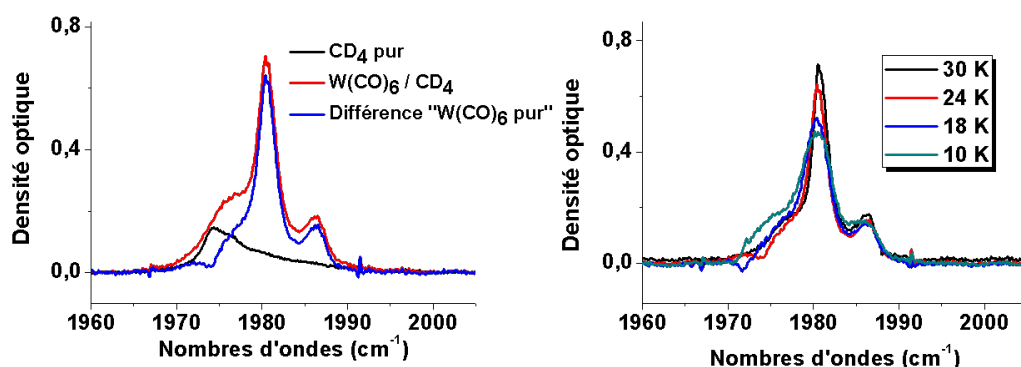
FIGURE 4.28 – Spectres d'absorption de \text{W}(\text{CO})_6 en matrice de \text{CD}_4 dans la région des élongations CO à 24 K. - A gauche, on a superposé un spectre d'absorption de \text{CD}_4 pur ; la différence entre les deux spectres est également représentée. A droite, évolution des spectres de différence pour quatre températures entre 10 et 30 K.
