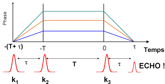
FIGURE 2.3 – Illustration de la dispersion de la phase des différents dipôles puis de la remise en phase générant l'écho de photons. - Durant le temps d'attente T , la phase est imprimée dans le système, elle n'évolue pas. Seules les populations peuvent relaxer.
