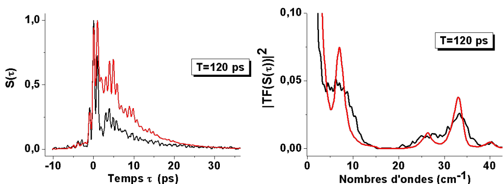
FIGURE 5.12 – Signal d'  cho de photons stimul  s de \text{Fe}(\text{CO})_5/\text{N}_2    20 K. - A droite, module au carr   de la transform  e de Fourier du signal d'  cho. Le temps T=120 ps. Le signal exp  rimental est en noir, le mod  le est en rouge. Voir texte pour les param  tres du mod  le.
