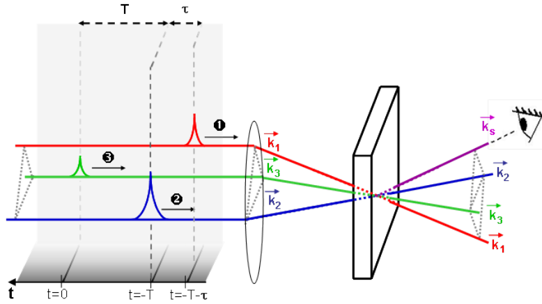
FIGURE 2.1 – Représentation schématique de la séquence d'impulsions arrivant sur l'échantillon. - Les impulsions 1 (en rouge) et 2 (en bleu) sont décalées du temps \tau . Les impulsions 2 et 3 (en vert) sont décalées de T . On définit t=0 le temps où la troisième impulsion arrive sur l'échantillon. Les trois faisceaux sont focalisés en un même point sur l'échantillon et le signal d'écho (en violet) est produit dans une direction dictée par les conditions d'accord de phase.
