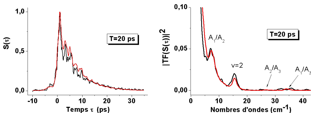
FIGURE 5.11 – Signal d'  cho de photons stimul  s de \text{Fe}(\text{CO})_5/\text{N}_2    20 K. - A droite, module au carr   de la transform  e de Fourier du signal d'  cho. Le temps T=20 ps. Le signal exp  rimental est en noir, le mod  le est en rouge. Voir texte pour les param  tres du mod  le.
