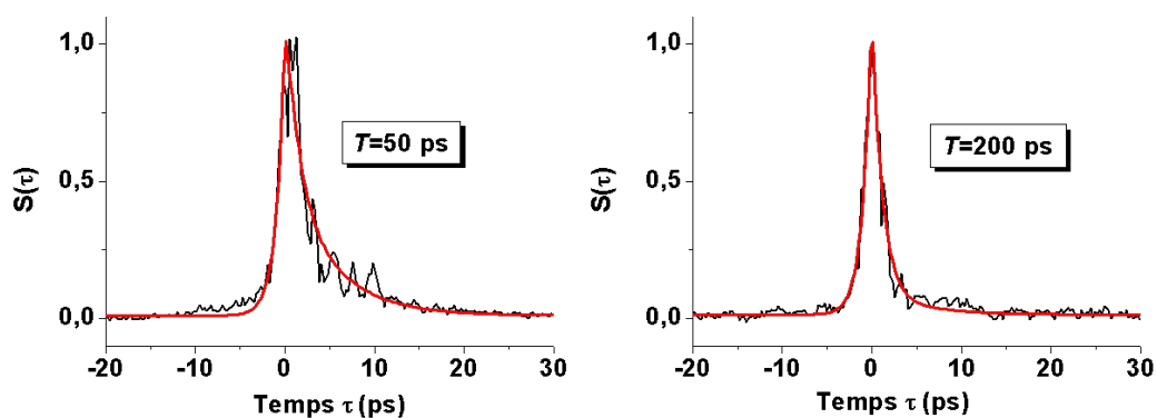
FIGURE 4.13 – Signaux d'échos de photons en présence de diffusion spectrale. - les signaux expérimentaux (en noir) sont modélisés (en rouge) par l'expression 2.49. A gauche, T=50 ps. A droite, T=200 ps.
