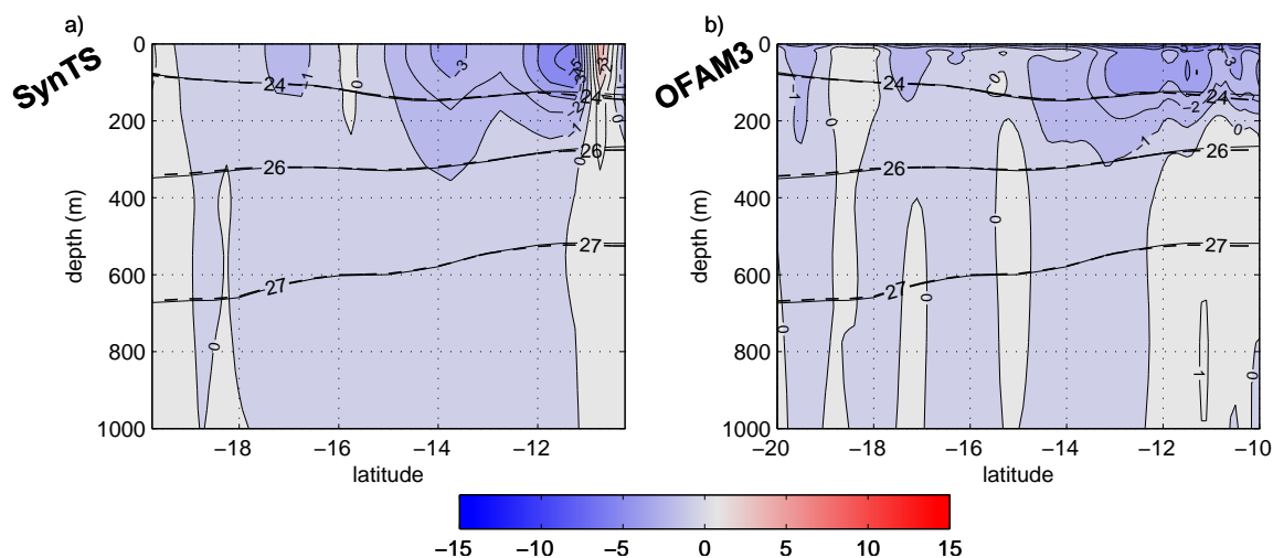
Figure V.12: Anomalies de vitesses (en \text{cm.s}^{-1} ) lors des épisodes El Niño le long de la radiale 161°E; a) méthode SynTS, b) modèle OFAM3; les isopycnes 24, 26 et 27 sont indiquées en trait plein noir (positions moyennes en trait tireté).
