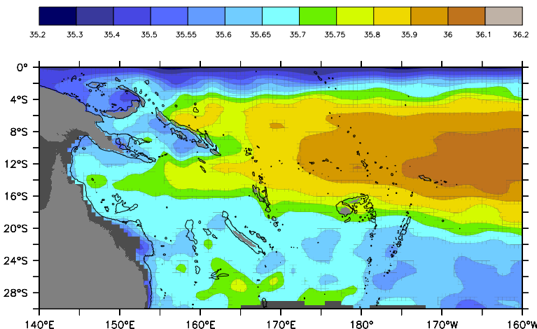
Figure I.18: Salinité au niveau de l'isopycne \sigma=25 \text{ kg}\cdot\text{m}^{-3} représentant les eaux de thermocline tropicales, (Climatologie CARS, Ridgway & Dunn, 2003)
