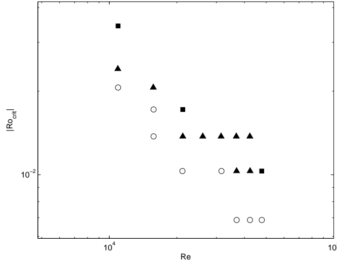
Figure 6.3: Diagramme de stabilité pour un écoulement de base de cisaillement. Expériences stables (○). Expériences instables (▲) visualisées avec des particules de Kalliroscope. Expériences instables (■) avec visualisation par PIV de modes libres ayant des nombres d'onde azimutaux m_1 = 4 et m_2 = 5 . Le rapport de fréquence et le rapport d'aspect valent \omega = 1.20 et h = 3 .
