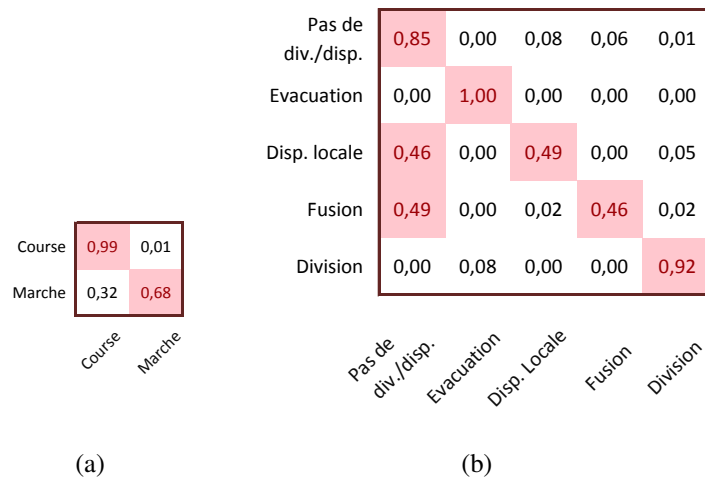
FIGURE 5.14 – Les matrices de confusion obtenues en utilisant le classificateur 'Forêt aléatoire', (a) les évènements marche et course, (b) Les évènements fusion, division, dispersion locale et évacuation
