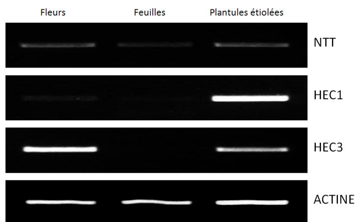
Figure 33 : Expression des gènes codant pour les facteurs de transcription NTT et HECATE dans les plantules étiolées 3 jours.
