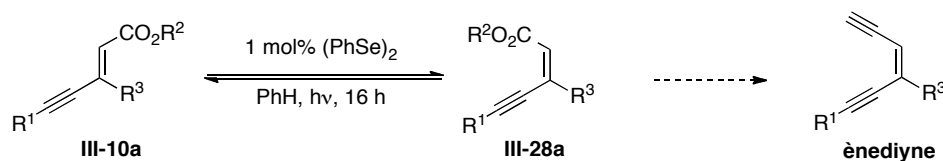
Schéma 94 : Isomérisation de l'ényne par action de (PhSe) 2
