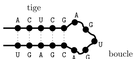
FIG. 1.12 – Exemple de formation d'une tige-boucle.
