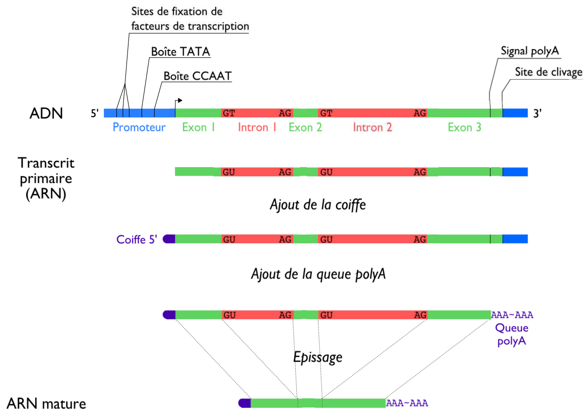
FIG. 1.6 – Processus de maturation des transcrits primaires.
