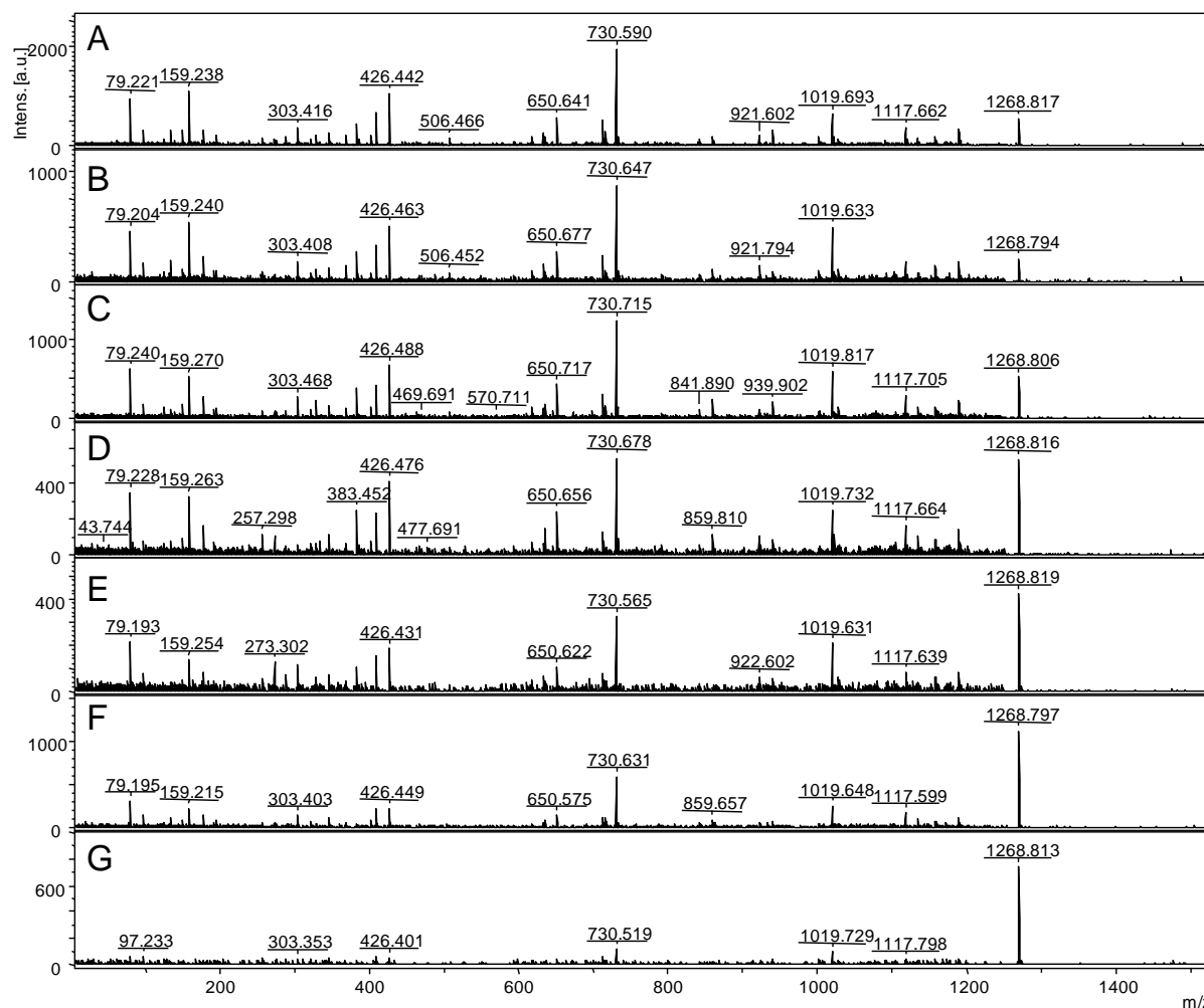
Figure 1.6: Spectres CID, par MALDI-TOF/TOF, en mode négatif, de l'ion parent [M-H]^- m/z 1268,808 de la chimère GCT A obtenus avec une fluence de : (A) 100% ; (B) 90% ; (C) 80% ; (D) 70% ; (E) 64% ; (F) 60% et (G) 50%. La base A , soulignée et en gras, est un ribonucléotide possédant un groupement 3'- PO_4H_2 .
