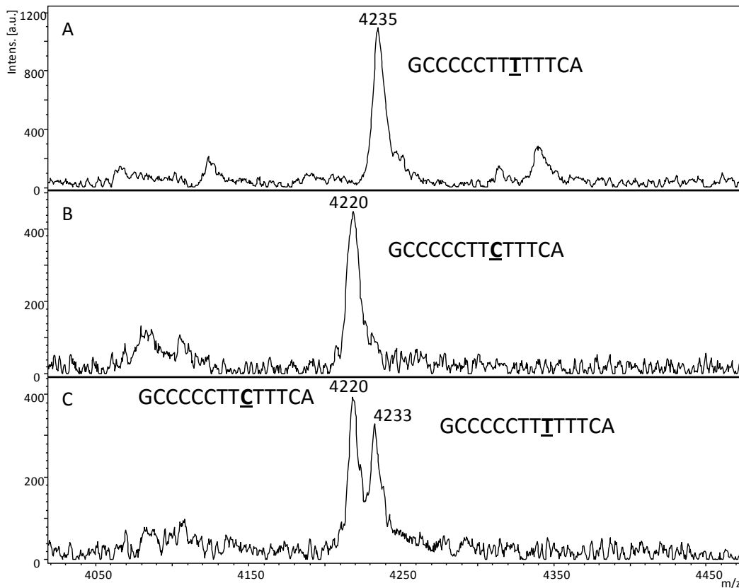
Figure 4.2 : Spectres de masse MALDI-TOF de la région des 14-mer de la ribo-PCR ATP des fragments anti-sens [M-H]^- du locus NOS1 rs3741476 d' : (A) un homozygote A; (B) un homozygote G et (C) un hétérozygote R. L'ion [M-H]^- GCCCCCTTCTTTCA représente l'allèle G et l'ion [M-H]^- GCCCCCTTTTTTCA représente l'allèle A.
