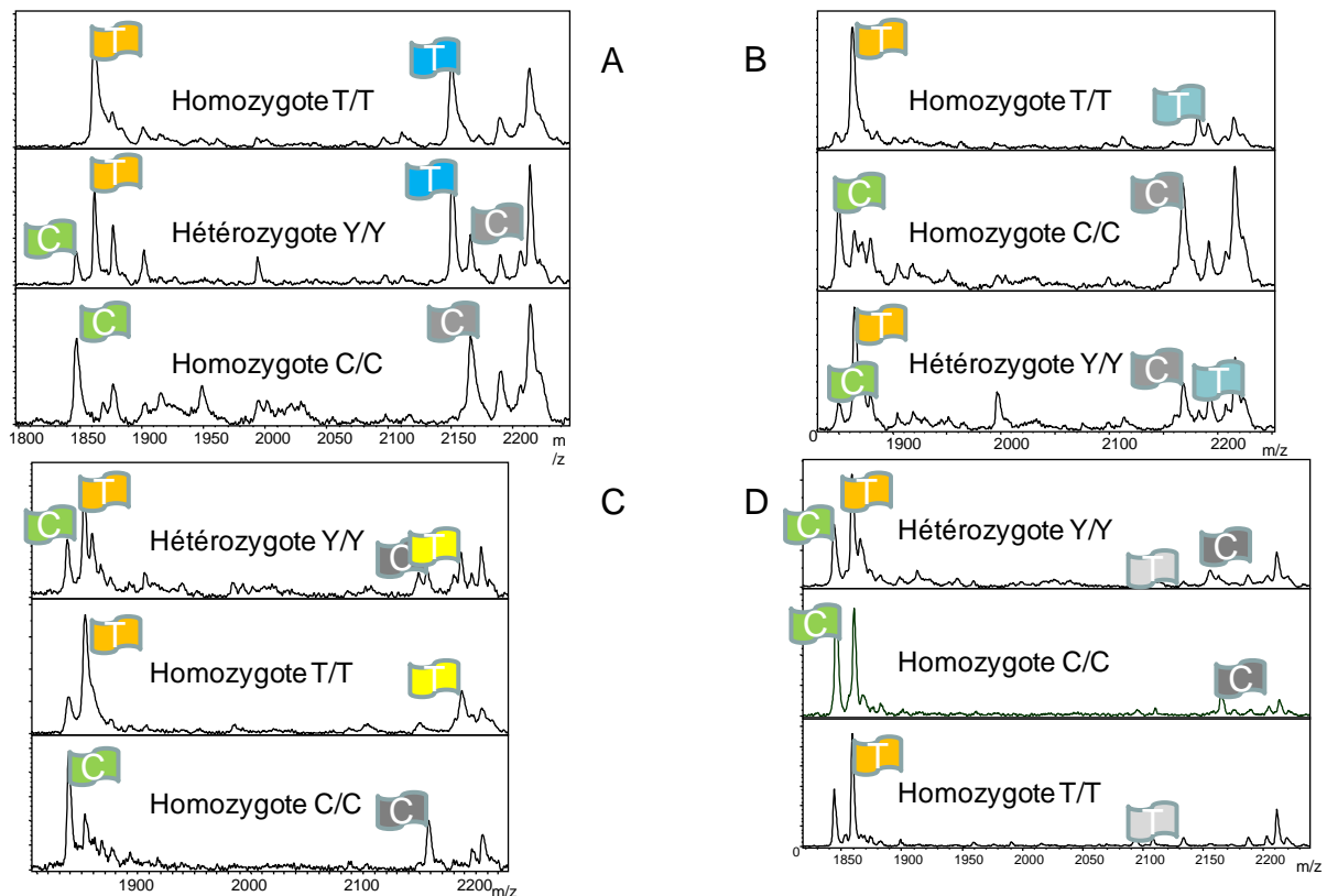
Figure 5.7 : Spectres de masse MALDI-TOF de la région des 6 à 7-mer du duplex de la riboPAP-PCR GTP des flags [M-H]^- des locus SLCO1B1 rs4363657 et rs4149056. Le flag orange CTCTAG correspond à l'allèle T et le flag vert CTCCAG correspond à l'allèle C du SNP rs4363657 tandis que le flag gris TCTCTAG correspond à l'allèle C du SNP rs4149056. Les flags suivants correspondent à l'allèle T du SNP rs4149056 (A) bleu TCCTCAG; (B) bleu clair TTTCTAG; (C) jaune TTTTTAG et (D) gris clair CCTCCAG. Les fragments proviennent du re-séquençage de la riboPAP-PCR du locus rs4149056.
