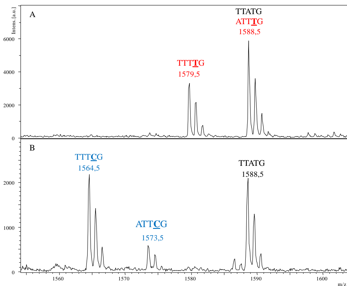
Figure 3.5 : Spectres de masse MALDI-TOF en mode réflecteur de la région des 5-mer de l'élongation linéaire GTP des ions [M-H] des fragments de clivage du locus CDKN2A- msp1 d'un ADN: (A) 0% méthylé et (B) 100% méthylé. Les ions [M-H] ATTTG , TTTCG , en rouge, représentent les CpGs 0% méthylé alors que les ions [M-H] ATTCG , TTTCG , en bleu, représentent les CpGs 100% méthylé. L'ion [M-H] TTATG est un fragment de clivage du re-séquençage du locus.
