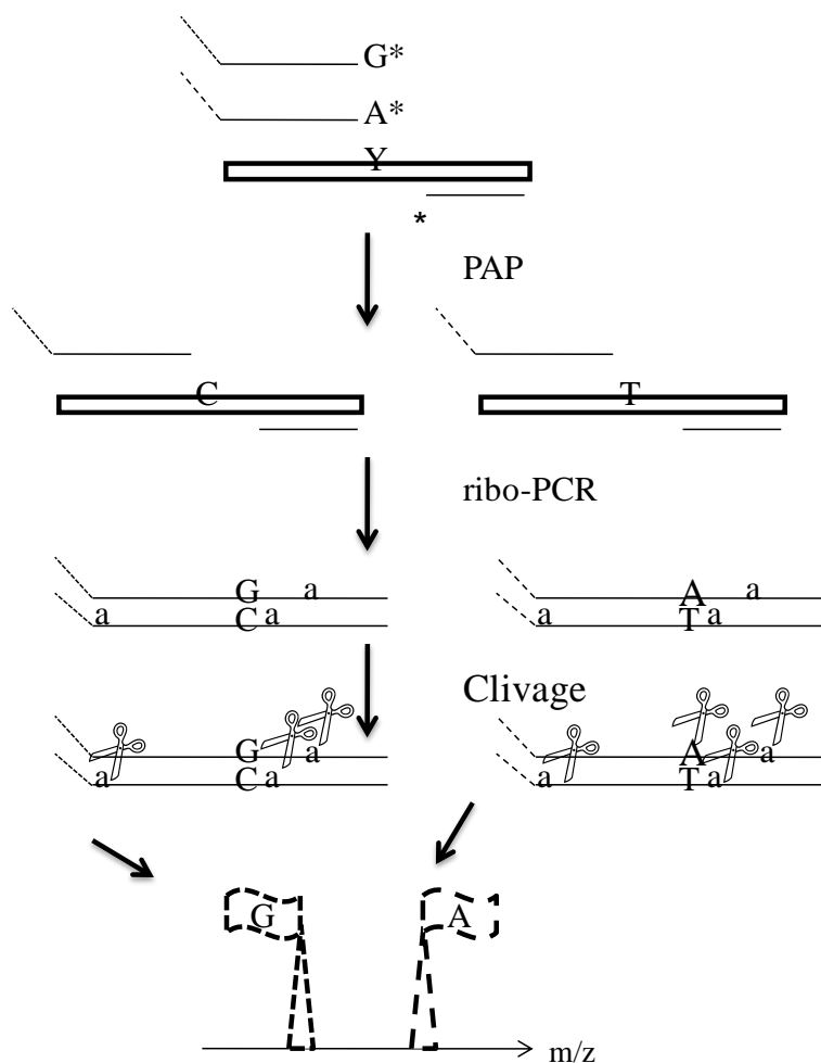
Figure 5.1 : Principe de la riboPAP-PCR avec ATP pour l'étude d'un SNP Y. Tout d'abord, une réaction de pyrophosphorolyse, PAP, a lieu lors de l'accroche des amorces allèles-spécifiques contenant les tags sur l'ADN. La dernière base qui contient la modification * 2' PO 4 est enlevée. Puis, la réaction de ribo-PCR ATP a lieu en incorporant de nouveau la dernière base des amorces. Elle est ensuite clivée afin d'analyser les séquences allèles-spécifiques flag par MALDI-TOF MS.
