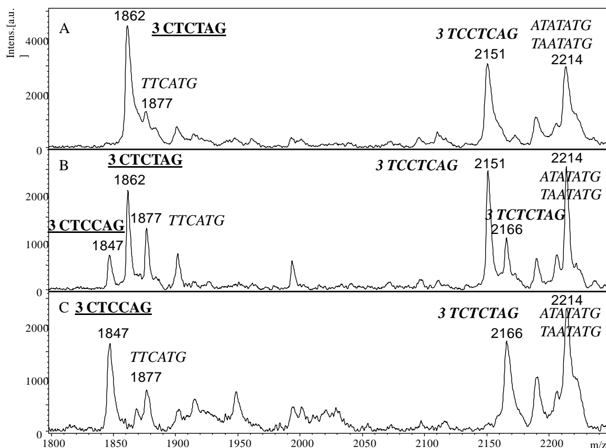
Figure 5.4: Spectres de masse MALDI-TOF de la région des 6 à 7-mer du duplex de la riboPAP-PCR GTP des flags [M-H]^- des loci SLCO1B1 rs4363657 et rs4149056 d' : (A) un homozygote TT-IT; (B) un hétérozygote TC-TC et (C) un homozygote CC-CC. Les flags du SNP rs4363657 sont en gras et soulignés tandis que les flags du SNP rs4149056 sont en gras et en italique. Les autres fragments proviennent du re-séquençage de la riboPAP-PCR du locus rs4149056. L'ion [M-H]^- CTCTAG représente l'allèle C et l'ion [M-H]^- CTCCAG représente l'allèle T du SNP rs4363657. L'ion [M-H]^- TCCTCAG représente l'allèle T et l'ion [M-H]^- TCTCTAG représente l'allèle C du SNP rs4149056.
