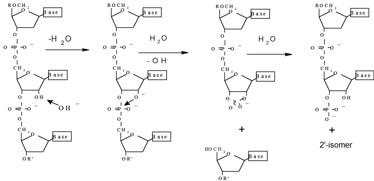
Figure 15 : Réaction de clivage de la chaîne nucléotidique située après un ribonucléotide, en milieu basique au niveau de la liaison P-O du phosphodiester: substitution nucléophile au niveau de l'atome de phosphore suivant le ribonucléotide (Shabarova & Bogdanov 1994).
