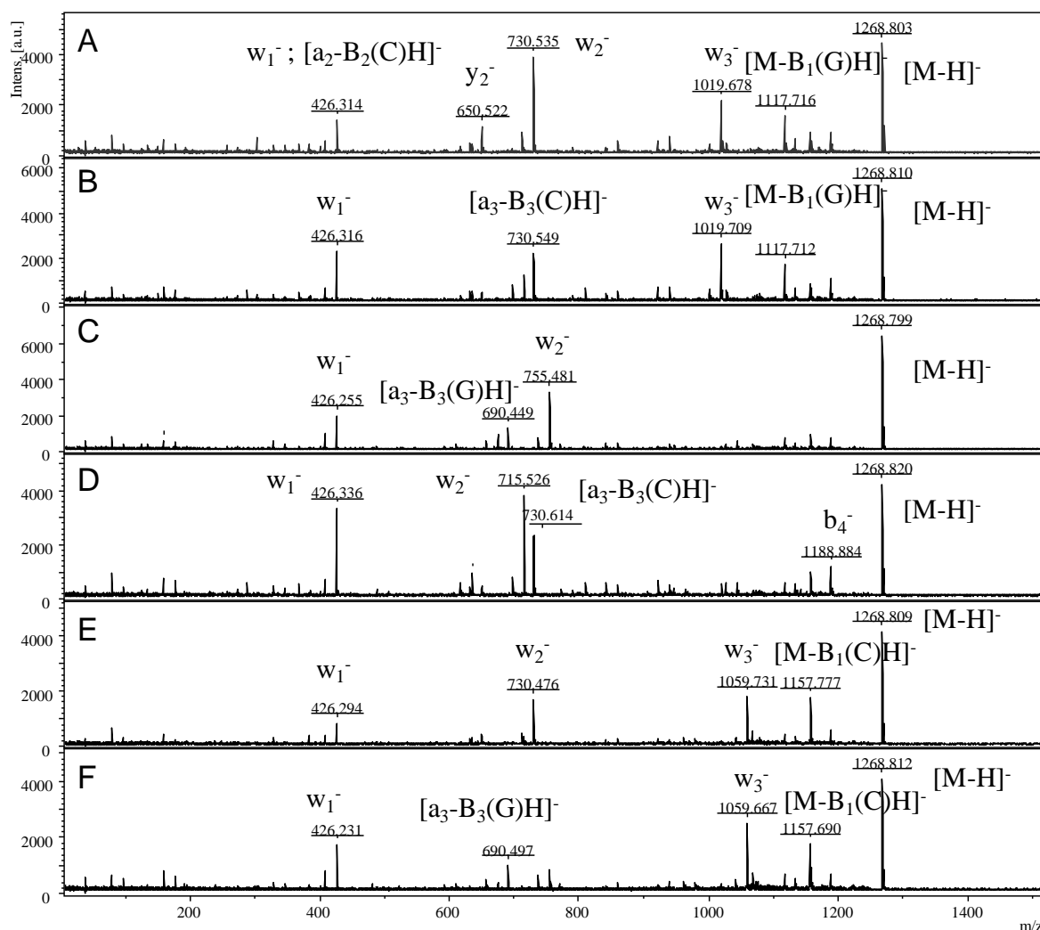
Figure 1.2: Spectres CID, par MALDI-TOF/TOF, en mode négatif, de l'ion parent [M-H]^- m/z 1268,808 des isomères : (A) GCTA ; (B) GTCA ; (C) TCGA ; (D) TGCA ; (E) CGTA et (F) CTGA . La base A , soulignée et en gras, est un ribonucléotide possédant un groupement 3'-PO 4 H 2 .
