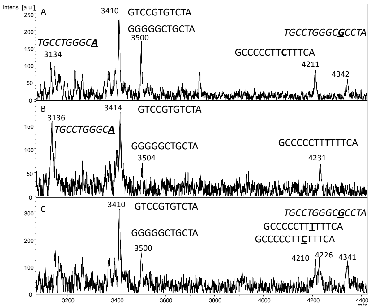
Figure 4.5 : Spectres de masse MALDI-TOF de la région des 10 à 14-mer du duplex de la ribo-PCR ATP des fragments anti-sens [M-H] des loci NOS1 rs3741476 et H19 rs2839698 d': (A) un homozygote G et un hétérozygote Y; (B) un homozygote A et un homozygote T et (C) un hétérozygote R et un homozygote C. L'ion [M-H] TGCCTGGGCA représente l'allèle T et l'ion [M-H] TGCCTGGGC CCTA représente l'allèle C du locus H19 . Ils sont en italique. L'ion [M-H]
