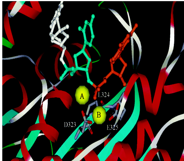
Figure 14 : Représentation du site des ADN polymérase permettant l'incorporation des NTPs.
