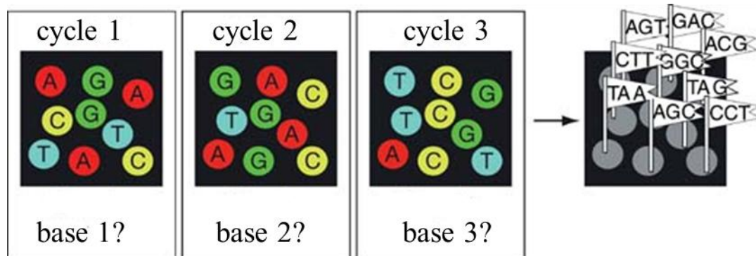
Figure 3 : Schéma de principe du séquençage cyclique sur puce, reproduit et modifié du site internet à l'adresse suivante : http://www.currentprotocols.com/protocol/mb0701 .
