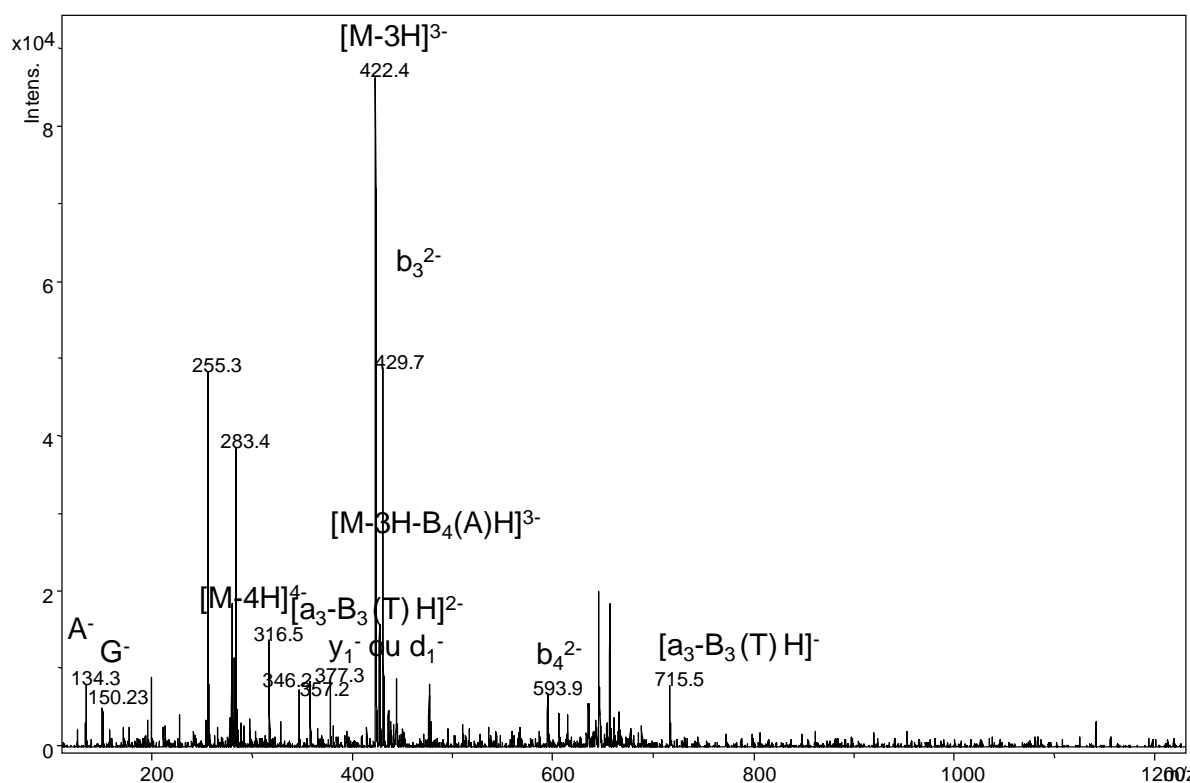
Figure 1.8: Spectre de masse, par ESI-ITMS, en mode négatif, de la chimère GCTA ( M=1269,816 Da). La base A , soulignée et en gras, est un ribonucléotide possédant un groupement 3'-PO_4H_2 .
