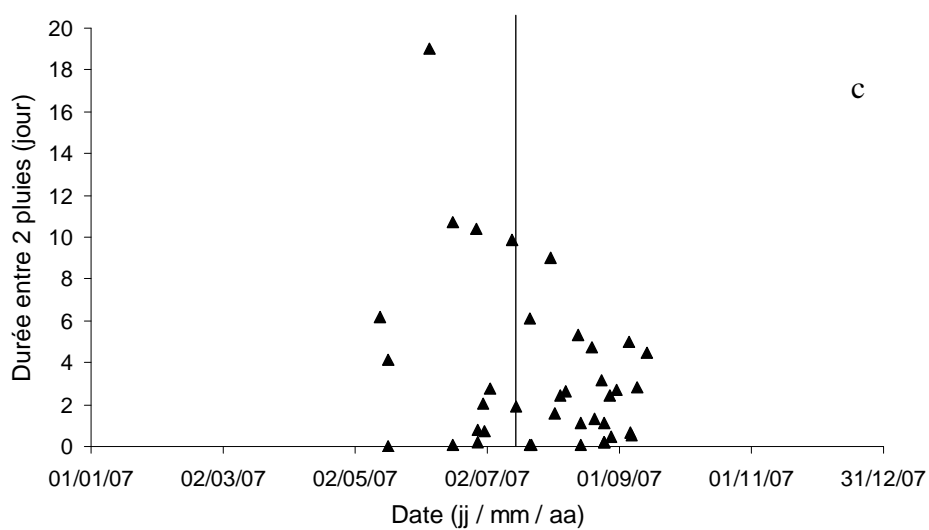
Figure 2.20 : Caractéristiques de l'érosion éolienne durant l'année 2007 : a) durée des événements érosifs, b) vitesse maximale des vents au cours de ces événements, c) durée entre deux pluies successives.
