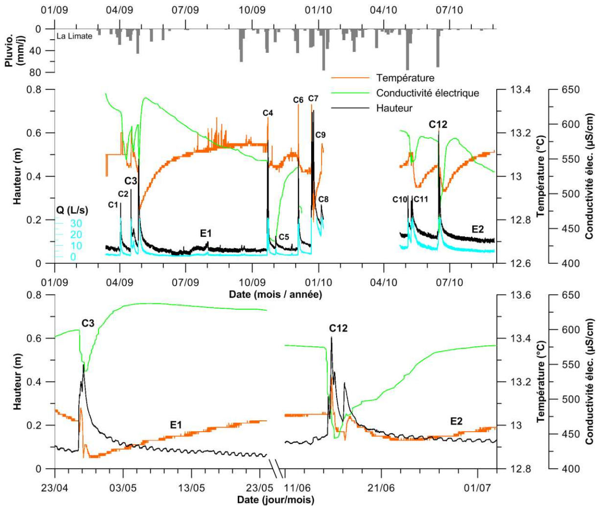
Figure 3.3 : Enregistrement CTD de la source de la Font d'Ouvin, associé aux précipitations journalières sur la même période. Les périodes d'étiage sont notées « E » et les crues « C ». Deux crues, C3 et C12, sont exposées à titre d'exemple.
