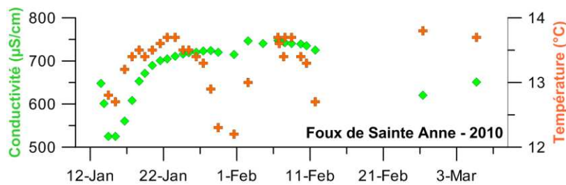
Figure 3.4 : Enregistrement manuel de la conductivité électrique et de la température, à l'aide d'un multimètre WTW 340i, au cours de l'hiver 2010 à la Foux de Sainte Anne d'Evenos.
