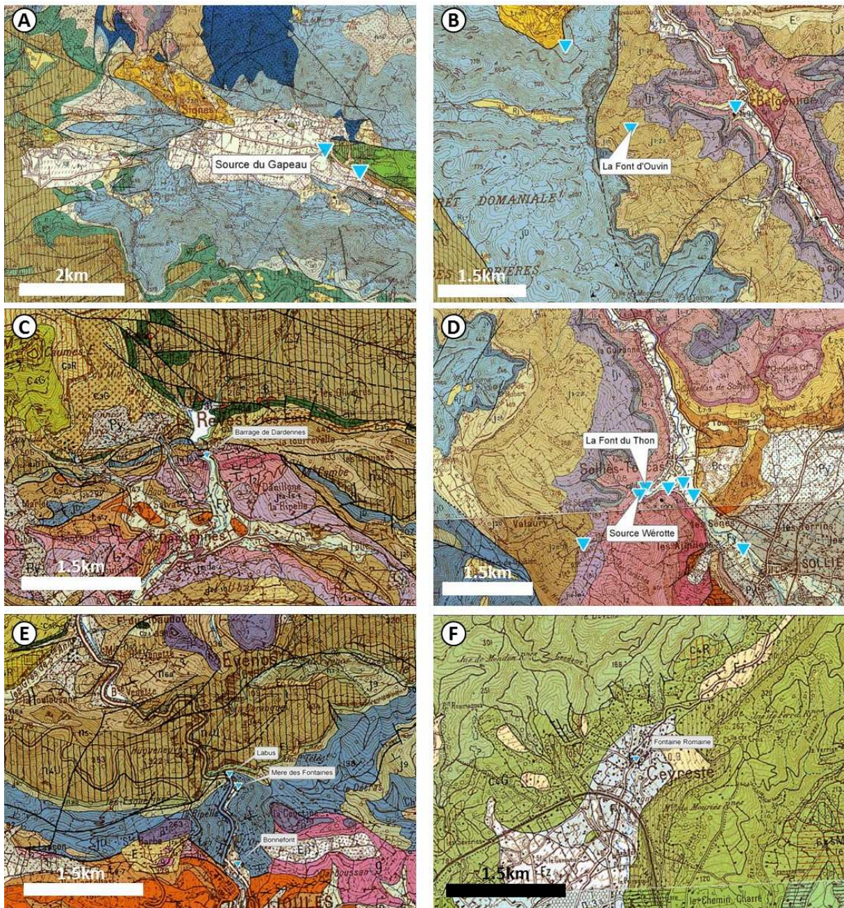
Figure 2.3 : Localisation des sources équipées sur les cartes géologiques au 1/50000 du BRGM. (A) Source du Gapeau à Signes à la charnière de l'Unité du Beusset et du Massif d'Agnis. (B) Source de la Font d'Ouvvin à Belgentier située sur les contreforts du Massif des Morières. (C) Conduite des fuites latérales du Barrage de Dardennes en contrebas de la retenue. (D) Sources de la Font du Thon et de Werotte dans le vallon de Valaury, affluent du Gapeau, à Solliès-Toucas. (E) Sources des Gorges d'Ollioules : Labus, source captée de Maire, ou Mère, des Fontaines et source de Bonnefont. (F) Source-puits de la Fontaine Romaine à Ceyreste.
