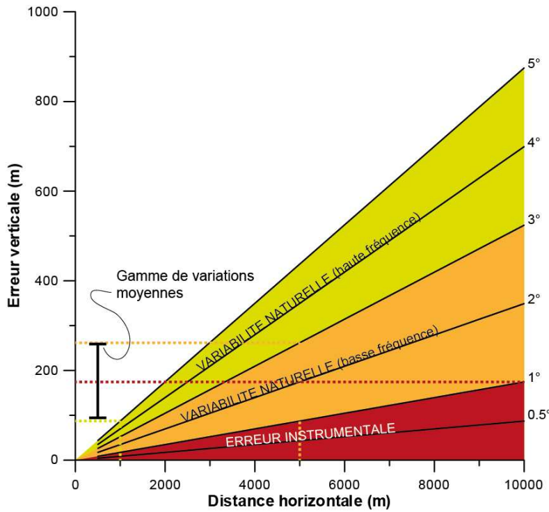
Figure 5.5 : Variations de l'erreur verticale en fonction de la distance entre le point de mesure du pendage et la charnière de pli, et selon l'angle de l'erreur sur le pendage. La gamme des variations moyennes est choisie selon la distance maximale observée pour chacun des trois types d'erreur.
