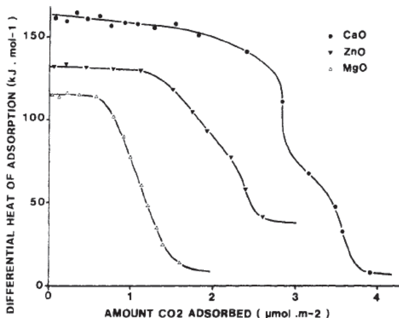
Figure 22 : Energie d'adsorption de CO 2 sur différents oxydes prétraités à 673 K d'après [28]
