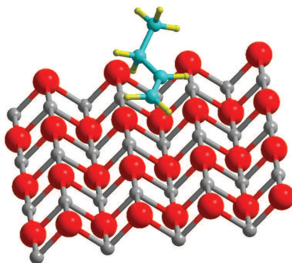
Figure 28 : adsorption du but-1-ène sur le plan (110)
