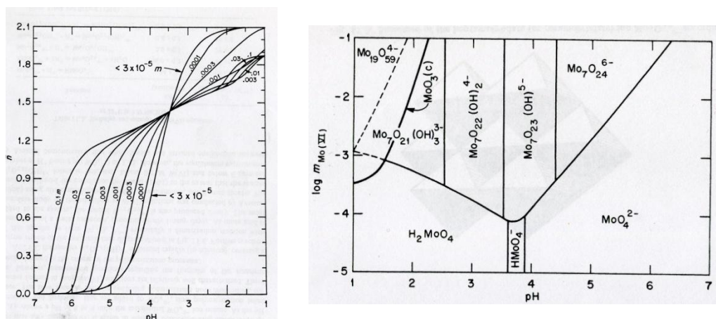
Figure I. 8 : Titrage protométrique d'une solution de MoO 4 2- à différentes concentrations. n représente le nombre de protons consommés par atome de Mo (gauche) Diagramme de prédominance des ions de Mo(VI) à 25°C et de force ionique I = 3M (droite)
