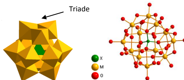
Figure I. 11 : Structure de l'HPA de Keggin, isomère α en modèle polyèdre (gauche) et modèle boule (droite)
