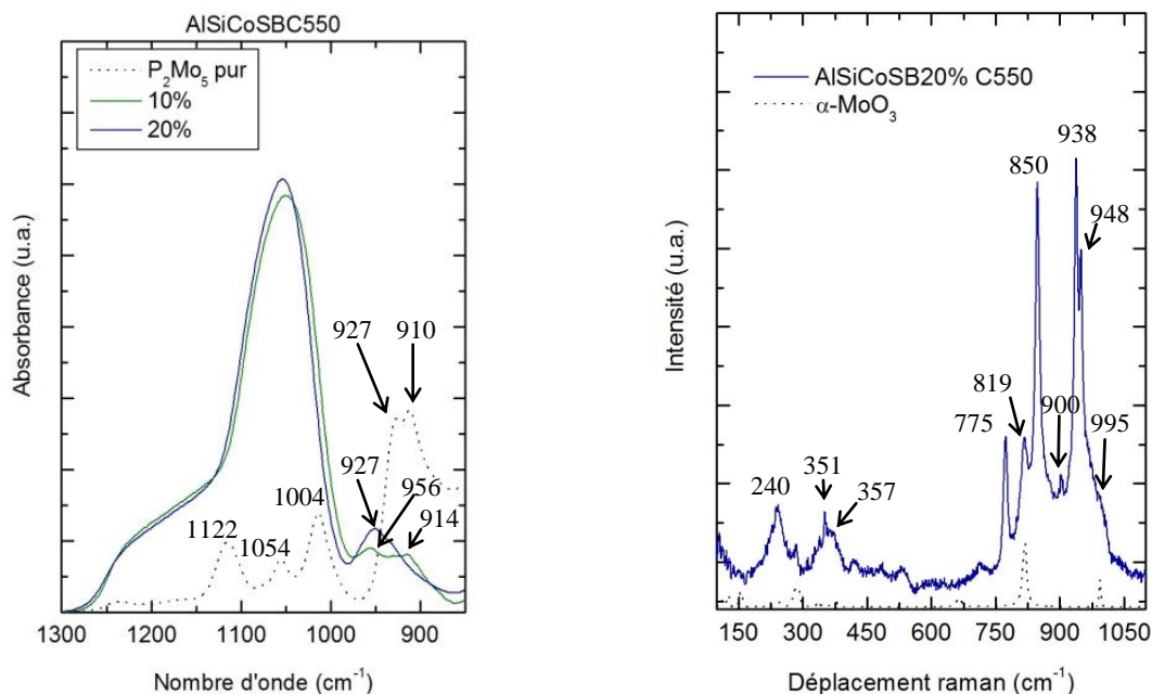
Figure III. 5 : Spectres IRTF (gauche) et Raman (droite) des matériaux AISiCoSB550 à 10% et 20 % de MoO 3 , les matériaux sont calcinés à 550°C
