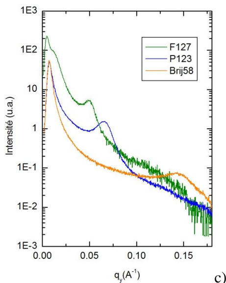
Figure II. 5 : Isothermes d'adsorption d'azote (a) distributions de la taille des pores calculées par la méthode BJH (b) et diagrammes SAXS (c) des matériaux SiKeg10%-Brij, P123 et F127
