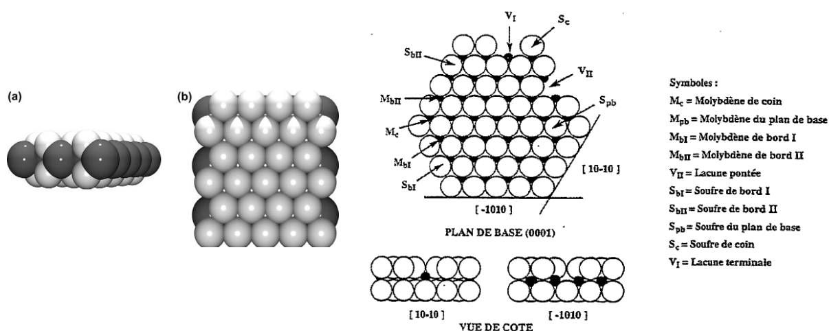
Figure I. 15 : Représentation d'un feuillet de MoS 2 (gauche) Enumération des différents sites de surface du MoS 2 (droite) selon 26
