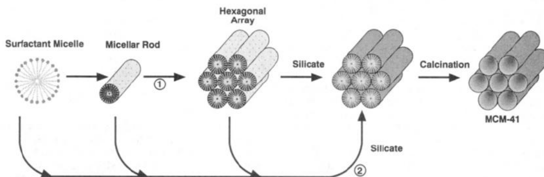
Figure I. 5 : Mécanismes proposés de formation de silice MCM-41 5
