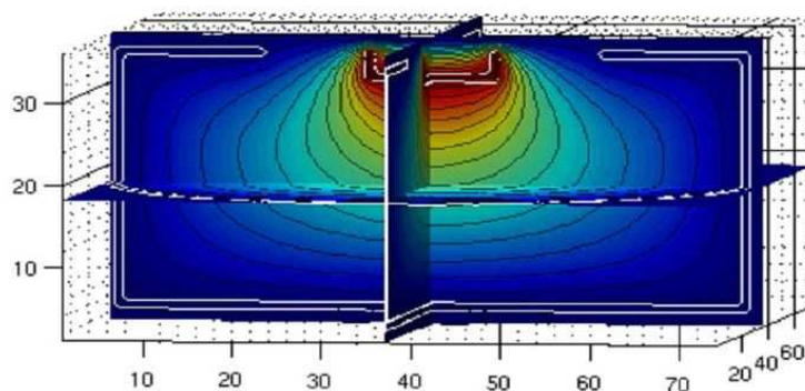
FIGURE 2.4.3: Lignes de champs électriques dans un cristal de Germanium Hyper Pur de type BeGe
