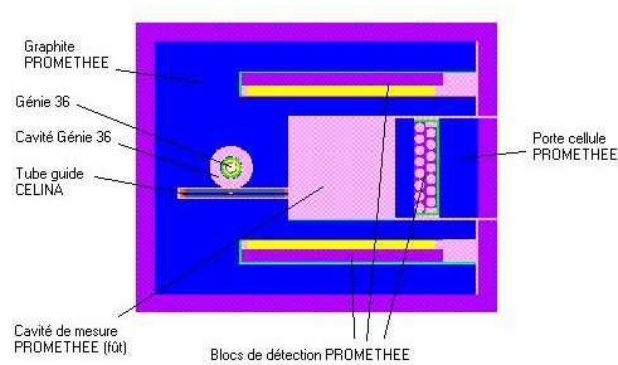
FIGURE 2.1.9: Vue de dessus du dispositif CELINA intégré dans PROMETHEE
