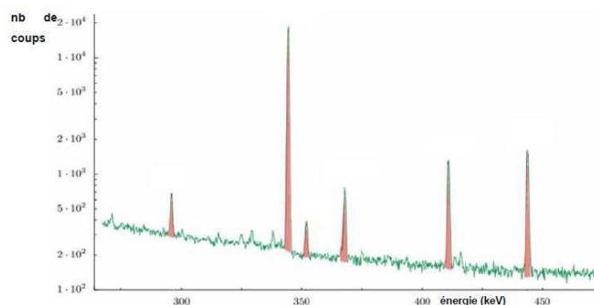
FIGURE 2.4.14: Spectre gamma d'une source étalon d'euporium152 entre 250 et 450 keV
