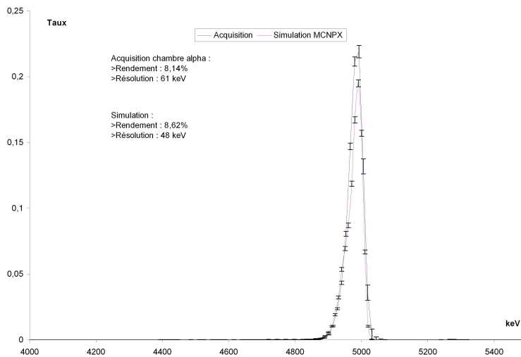
FIGURE 2.5.6: Spectres obtenus par modélisation et expérimentation avec un capteur PIPS dans la configuration de mesure de la figure 2.5.5
