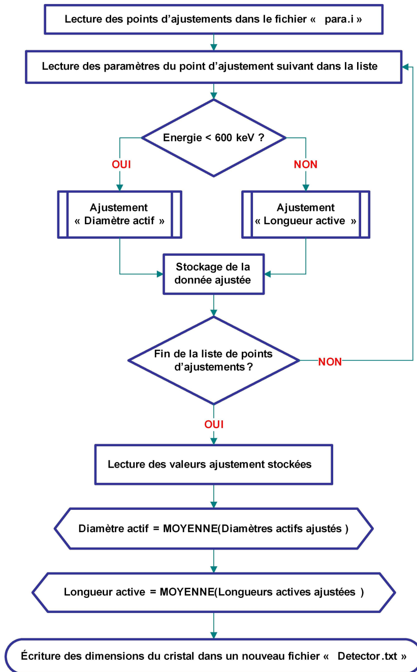
FIGURE 2.4.13: Diagramme de l'ajustement de l'épaisseur du modèle numérique du détecteur GeHP
