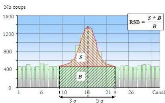
FIGURE 2.4.21: Illustration du rapport signal sur bruit d'un pic. Le RSB est défini par \frac{(S+B)}{B} où B est le fond sous le pic (calculé sur l'intervalle \pm 3\sigma ) et S+B est la somme du contenu des canaux sur l'intervalle \pm 3\sigma
