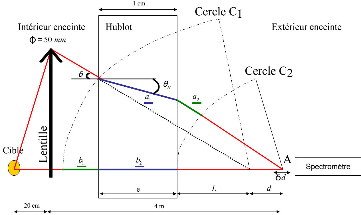
FIGURE 2.17 – Lors de la traversé d'un hublot, les rayons de la sonde ne parcourent pas la même distance dans le diélectrique, le phase acquise le long de la propagation va dépendre de l'angle d'incidence. Sur le schéma, \theta = \theta_{Max}
