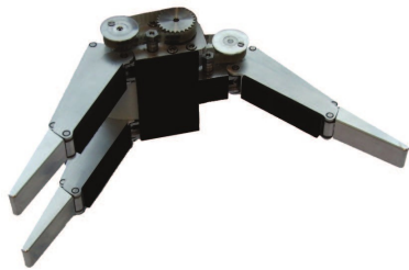
Delft Hand 2 (Meijneke, Kragten, and Wisse 2011)
