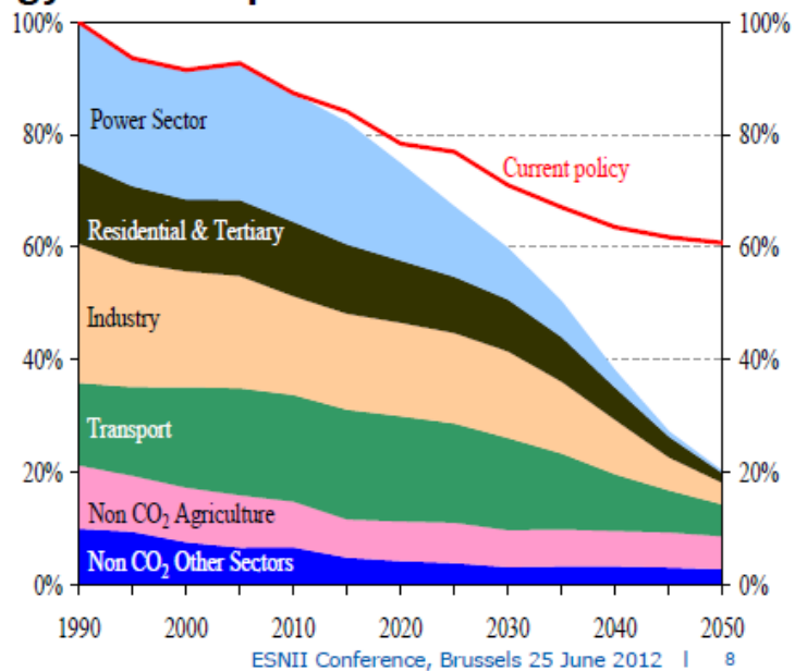
FIGURE I.5.2 – Objectif de réduction des gaz à effets de serre par poste de consommation d'énergie.
