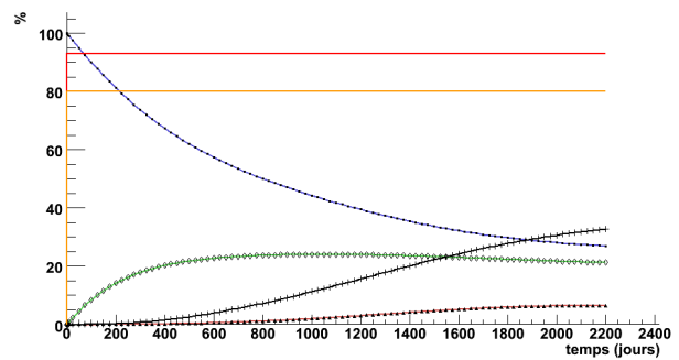
FIGURE III.2.28 – Nombre de boulets à détourner pour récupérer une SQ et qualité du plutonium produit en fonction du burnup (répartition des % des différents isotopes)
