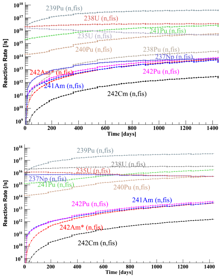
FIGURE III.3.13 – Contribution des fissiles et AM pour le cas proliférant d'origine (haut) et le cas de couvertures enrichies en 237 Np (bas)
