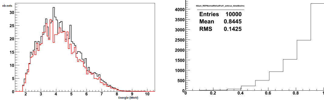
FIGURE II.4.4 – À gauche, les écarts entre le spectre 235 U (en noir), et 241 Pu (en rouge). À droite, le test de Kolmogorov-Smirnov indique une p-valeur moyenne de 0.84 entre les deux spectres, avec un écart en normalisation 12%.
