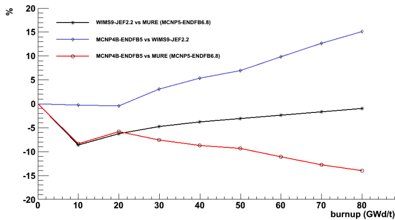
FIGURE III.2.7 – Comparaison des inventaires en 241 Pu entre notre simulation et les résultats des participants du benchmark
