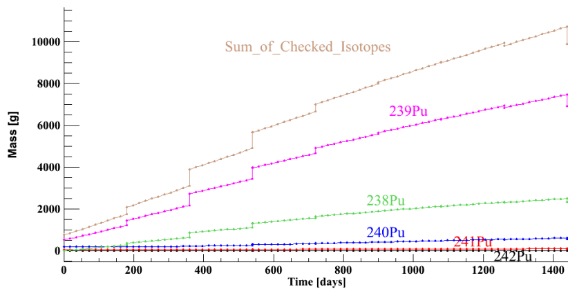
FIGURE III.3.14 – Transmutation des déchets et production de plutonium dans un huitième de couche radiale (cas du combustible utilisé de CANDU enrichi en 237 Np).
