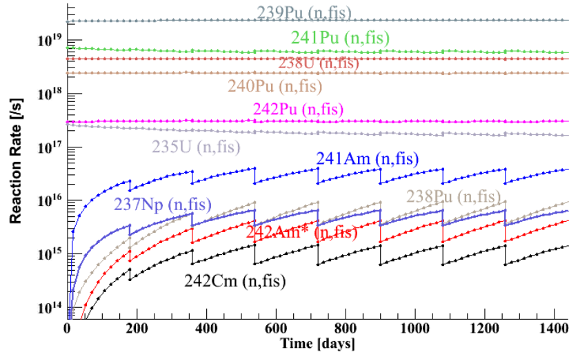
FIGURE III.3.4 – Contribution des différents noyaux à la production de puissance dans le cas proliférant.
