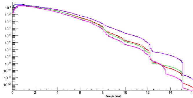
FIGURE I.6.5 – Flux des \bar{\nu}_e par fission de noyau fissile
