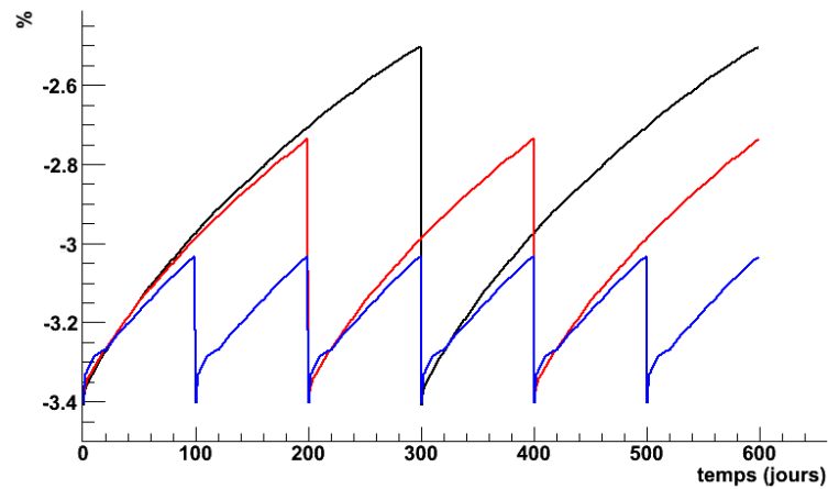
FIGURE III.1.12 – Évolution sur 600 jours de l'écart entre les figures III.1.10 et III.1.11
