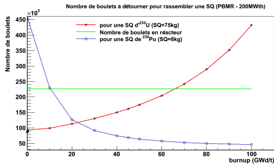
FIGURE III.2.28 – Nombre de boulets à détourner pour récupérer une SQ et qualité du plutonium produit en fonction du burnup (répartition des % des différents isotopes)
