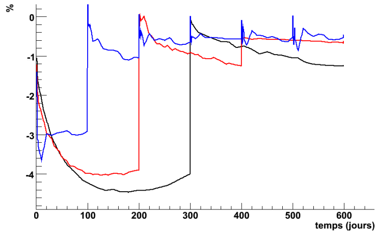
FIGURE III.1.22 – Écarts obtenus entre les calculs présentés en fig. III.1.18 et III.1.21.
