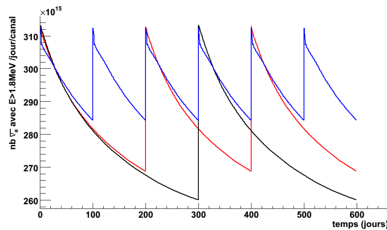
FIGURE III.1.14 – Méthode utilisée : produit des taux de fission par nos spectres d' \bar{\nu}_e émis par fission construits par Huber [5].
