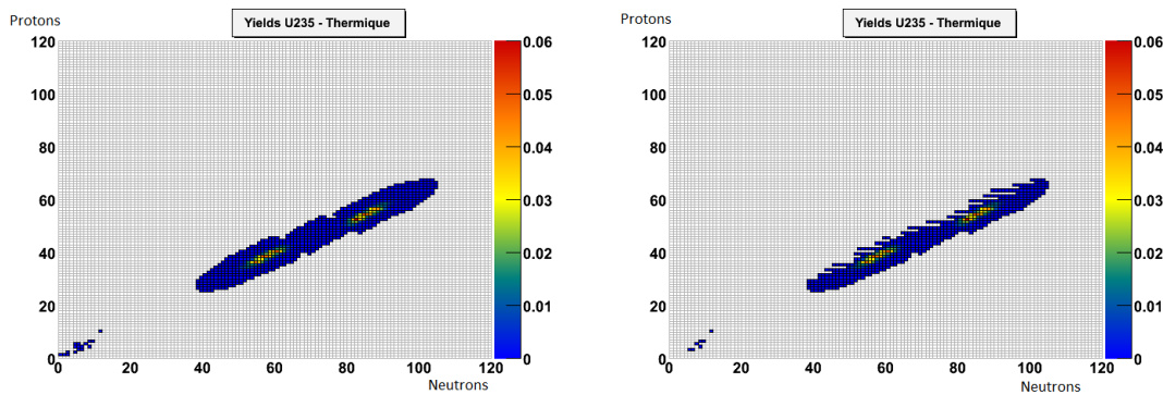
FIGURE I.1.3 – À gauche, distribution des produits de fissions de ^{235}\text{U} , à droite, ceux pouvant émettre des \bar{\nu}_e d'énergie > 1.8\text{ MeV}
