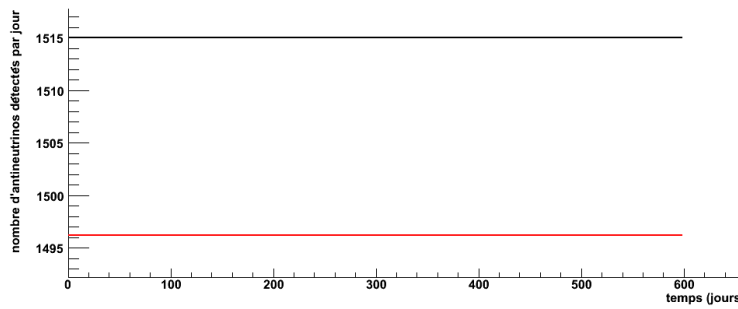
FIGURE III.1.23 – Écarts entre comportement légitime (en rouge) et proliférant (en noir) avec nos spectres à 12h.
