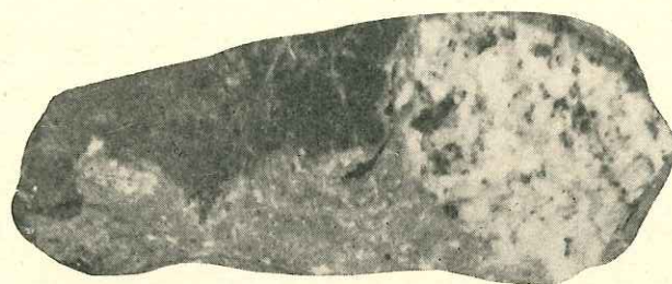
Fig. 11. Intrusion diabasique dans l'arkose (les Lanches). L'arkose (roche gris-clair, en bas), englobe un élément granitique (à droite). En haut, la diabase intrusive (roche foncée). Grandeur naturelle.
