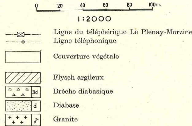
Fig. 17. Le Plenay. 1. Brèche diabasique à éléments sédimentaires et à ciment argileux.
