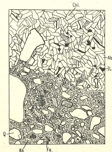
Fig. 21. Diabase albite-chloritique (en haut) transgressant sur arkose (en bas). (Les Pentes du Bouvier). 12×, lumière naturelle. Q: quartz; Ab: albite; Fa: feldspath alcalin très altéré (orthose?); Chl: chlorite; Il: ilménite.
