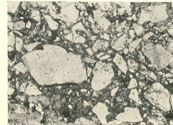
Fig. 31. Brèche de serpentine dans ciment calcitique. (Le Crêt). 24×, lumière naturelle.
