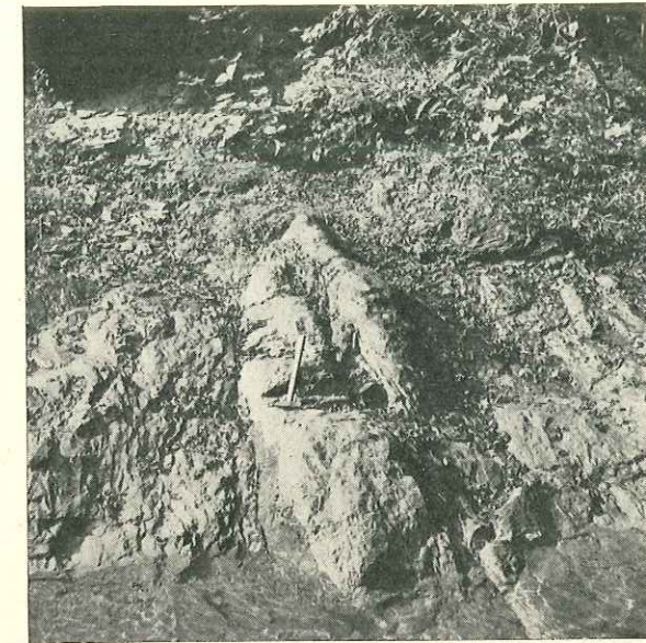
Fig. 8. Vers le Pré. Lentille inférieure d'ophisilice.
