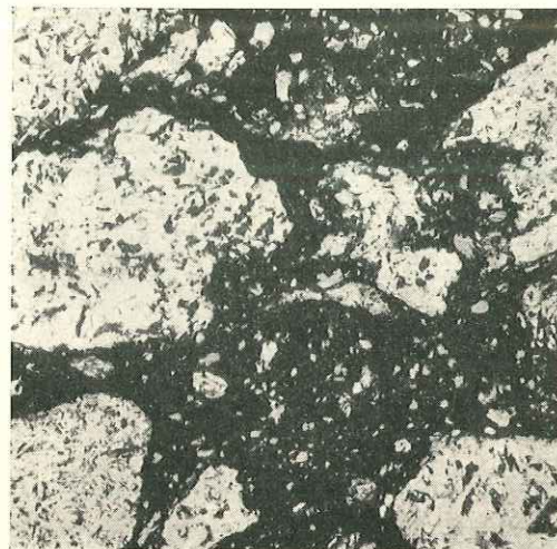
Fig. 29. Brèche d'éclatement. (Les Pentès du Bouvier). 24x, lumière naturelle. Débris de diabases albito-hématitiques dans une pâte hématitique.
