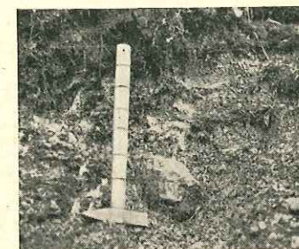
Fig. 33. Ophisphérite à moitié enfouie dans une serpentine très altérée (le Crêt).
