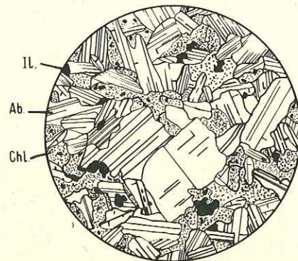
Fig. 23. Diabase intersertale grossière albito-chloritique. (Le Plenay). 12x, lumière naturelle. Ab: albite; Chl: chlorite; Il: ilménite. Le grand individu dans la partie inférieure du dessin est maclé suivant la loi acine-Ala.
