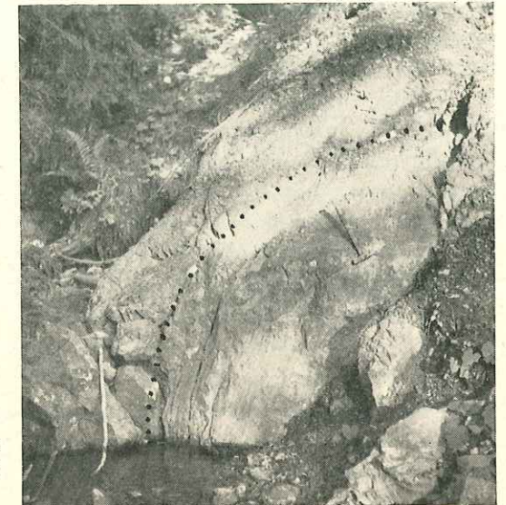
Fig. 6. Le Bartoli. Ophisphérite cyclopéenne. La ligne en pointillé sépare le centre de l'ophisphérite (à droite) du bord (à gauche).
