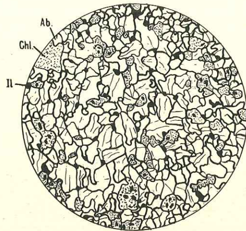
Fig. 24. Diabase hypidiomorphe albite-chloritique (élément de la brèche diabasique du Torrent des Bounaz). 12×, lumière naturelle. Ab: albite; Chl: chlorite; Il: ilménite.
