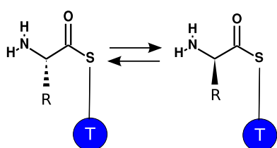
FIG. 1.11 – Réaction d'épimérisation sur l'acide aminé fixé sur le domaine de thiolation
