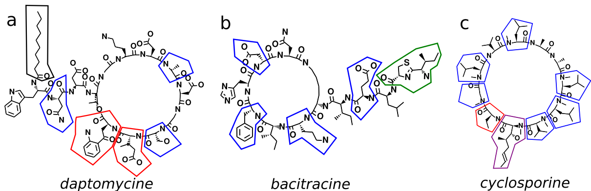
FIG. 1.24 – Structure de a) la daptomycine, b) la bacitracine A et c) la cyclosporine. Les acides aminés modifiés par des domaines secondaires sont encadrés en bleu, les acides aminés non-protéogéniques en rouge, l'hétérocycle (obtenu par un domaine secondaire) en vert, l'acide aminé non-protéogénique et modifié par un domaine secondaire en violet et l'acide gras en noir.
