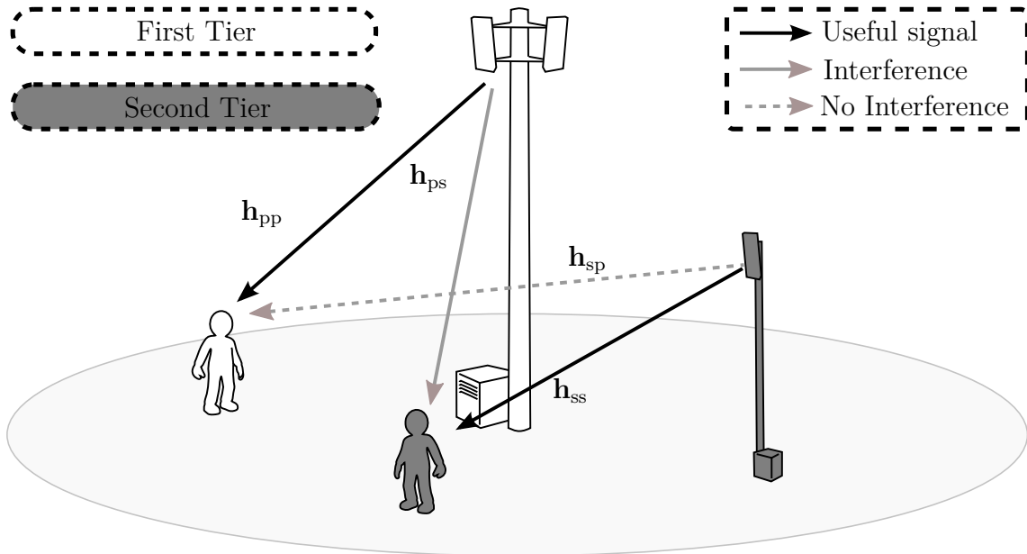
FIGURE 2 – Réseau à deux niveaux, une Small-cell.
