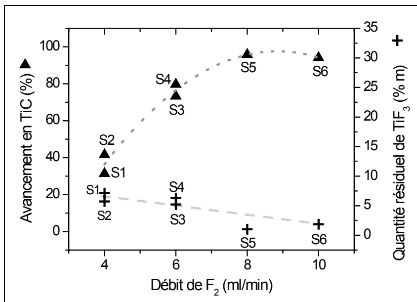
Figure 27 : Evolution de la transformation de TiC et TiF 3 en fonction du débit en F 2
