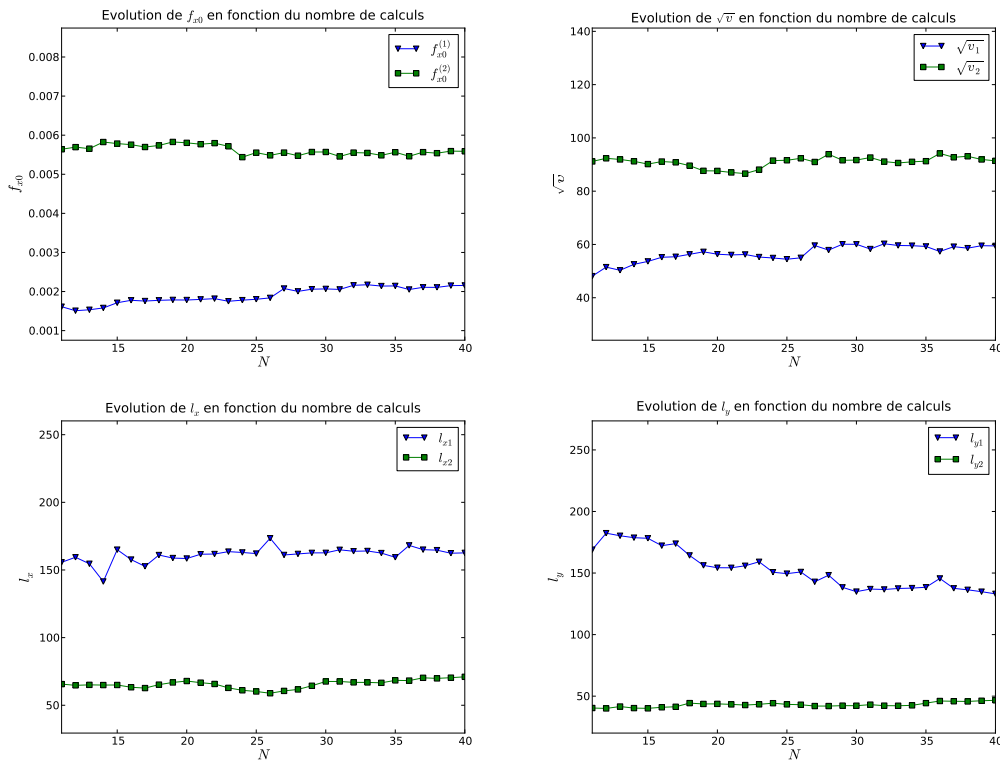
Figure 4.56 – Cas GF - Champ \sigma_I , E_{yy} = 3,5\% - Évolution des paramètres identifiés en fonction du nombre de réalisations du champ
