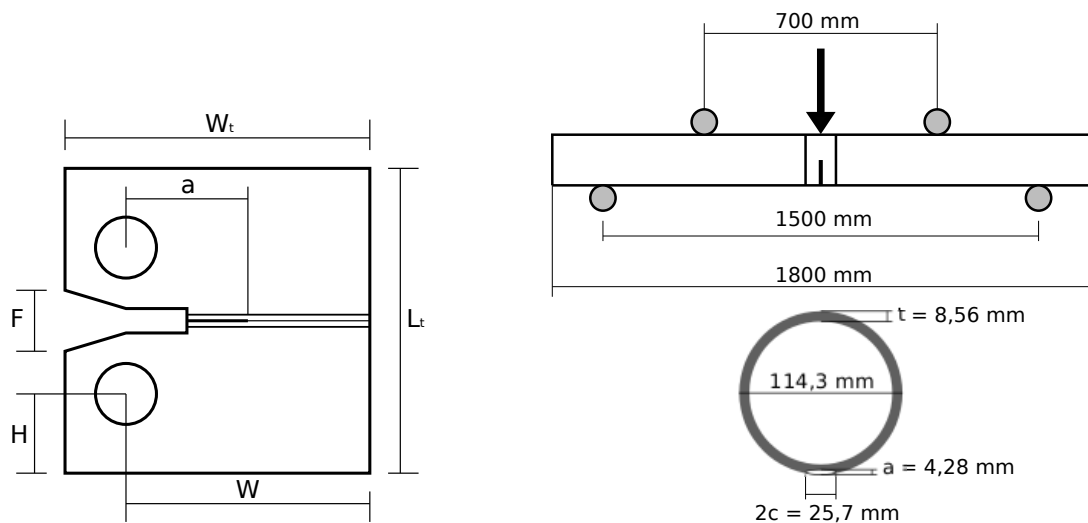
Figure 1.6 – Éprouvette CT ( B = 12,5 mm (épaisseur de l'éprouvette) ; W_t = 31,25 mm ; L_t = 30 mm ; W = 25 mm ; H = F = 8 mm ; a = 13,25 mm) à gauche et l'essai de flexion en quatre points à droite (Besson et al., 2004)
