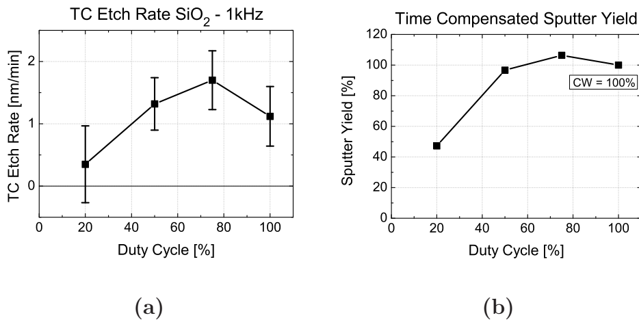
Figure A.8.: (a) Vitesse de la gravure en temps compensé de SiO 2 (matériau du masque) pour des rapports cycliques variés. (b) L'évolution approximée de la pulvérisation par rapport à un plasma continu (100%). Ce calcul est basé sur le flux d'ions de haute énergie et son énergie moyenne.
