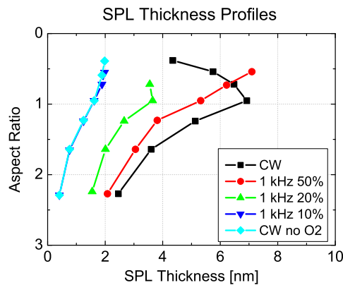
Figure A.10.: Epaisseur moyenne de la couche de passivation sur les flancs des motifs gravés dans un plasma pulsé de HBr/O_2 avec des rapports cycliques variés et en mode continue avec et sans O_2 .
