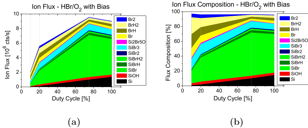
Figure A.3.: (a) Flux total d'ions d'un plasma HBr/O 2 AVEC polarisation du substrat et (b) sa composition relative.
