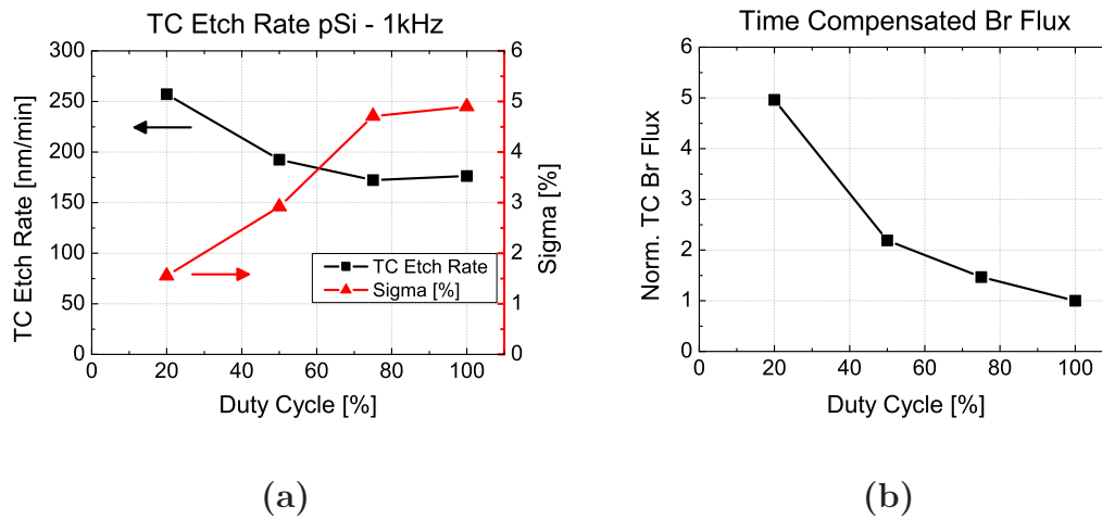
Figure A.7.: (a) Vitesse de la gravure en temps compensé de poly-silicium pour des rapports cycliques variés. (b) Flux de Br radicalaire en temps compensé.
