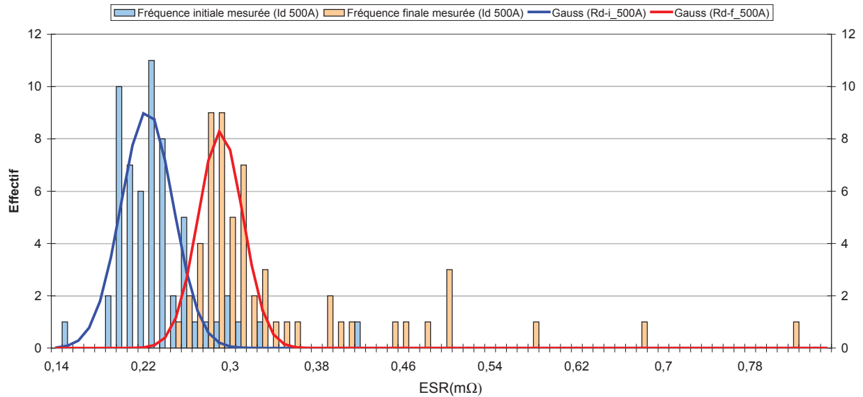
Figure 4. 25: Distributions initiale (Rd-i) et finale (Rd-f) des ESR obtenues par la méthode constructeur pour un cycle de charge décharge à 500A
