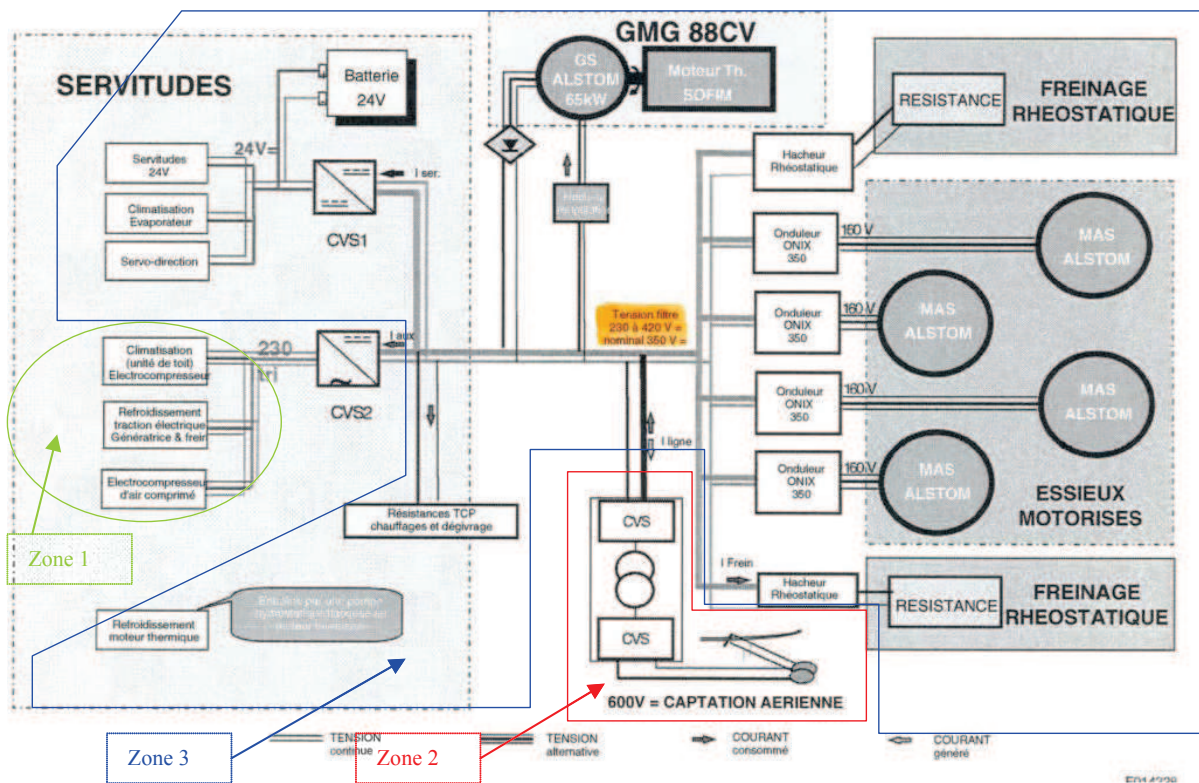
Figure 1. 2: Synoptique des lignes de puissance dans un trolleybus
