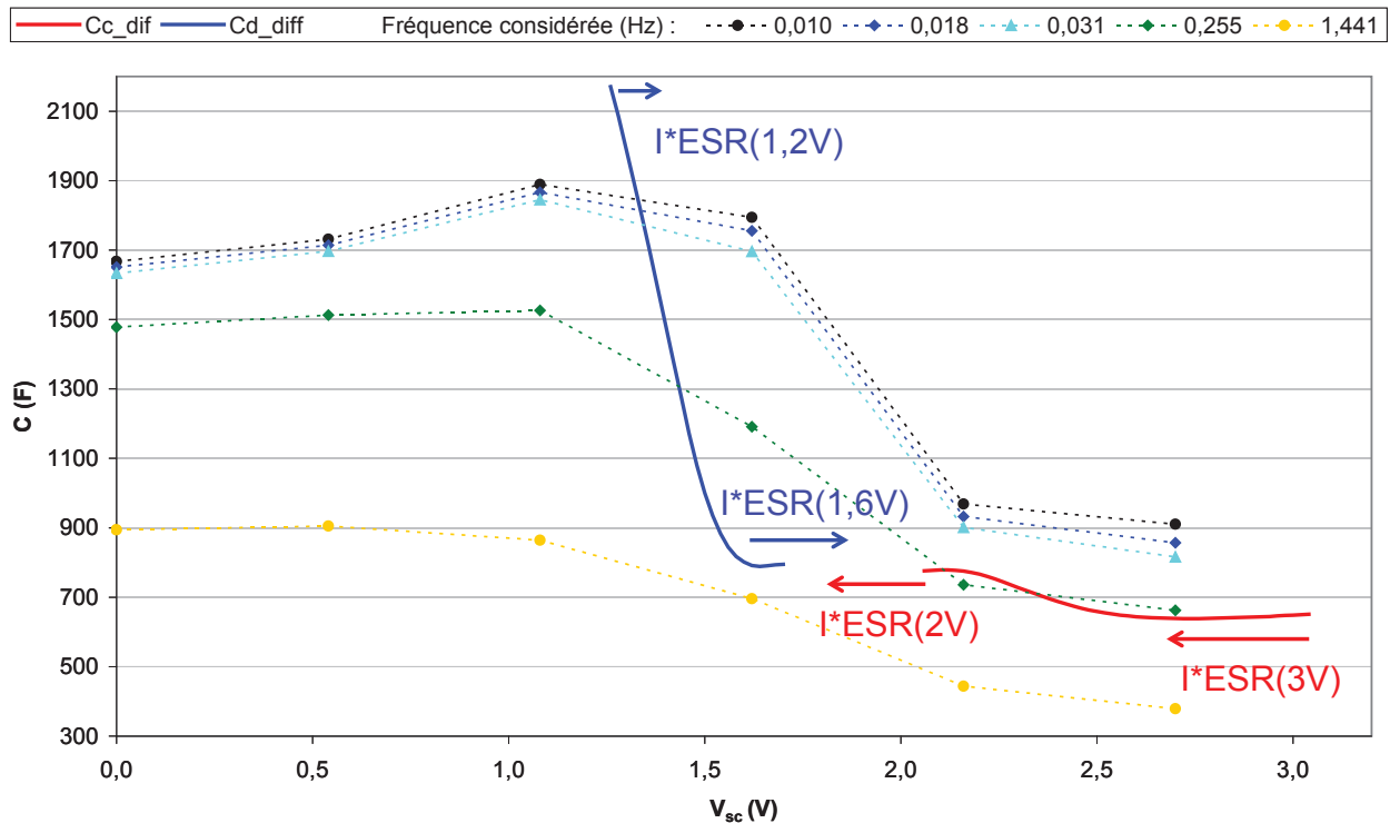
Figure 3. 35: C_{c\_diff}(V_{sc}) et C_{d\_diff}(V_{sc}) pour le dernier cycle (43000 ième ) et C(V_{sc}) capacité obtenue par spectroscopie complète 7h après l'arrêt du cyclage, et paramétré par la fréquence, le tout pour le composant P24
