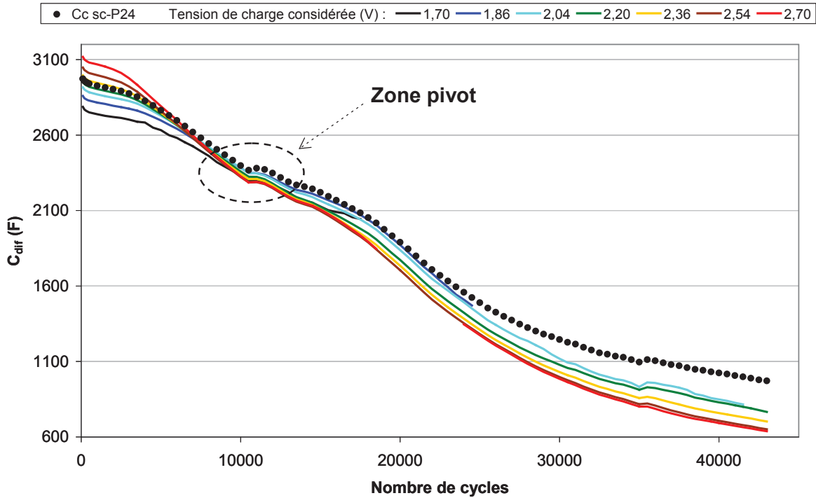
Figure 3. 30: C_{dif} charge et C_c du composant P24 ( I_{SC} de 300A) : Capacité différentielle obtenue pour certaines tensions de charge et capacité constructeur en fonction du nombre de cycles
