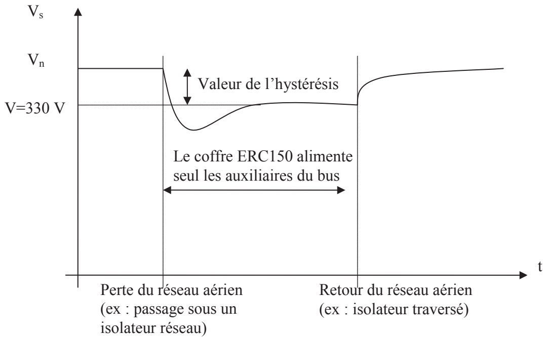
Figure 1. 4 : Tension du réseau de bord lors d'une micro-coupure
