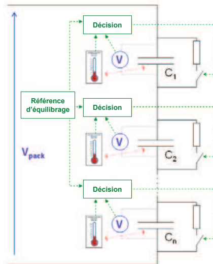
Figure 4. 28 : Système d'équilibrage retenu
