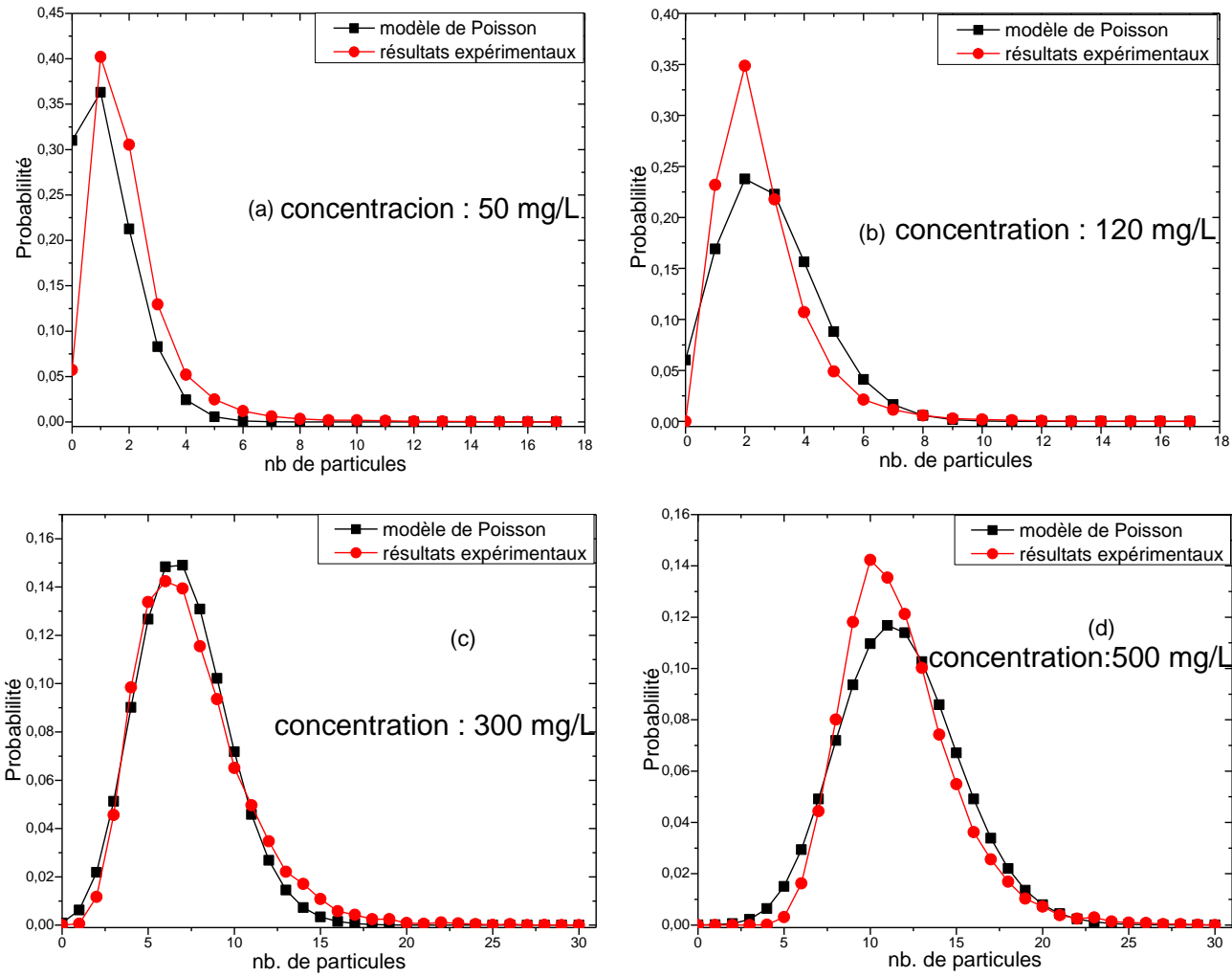
Figure III-1-11 : Comparaison des probabilités théoriques et la probabilité expérimentale du nombre de particules pour des suspensions de particules d' Al_2O_3 de diamètre nominal de 2 \mu m à différentes concentrations en Al total.
