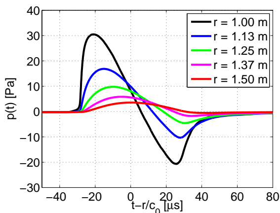
FIGURE 6.18: Formes d'onde de la solution analytique exprimée en somme de résidus, pour différentes distances curvilignes r depuis la source.
