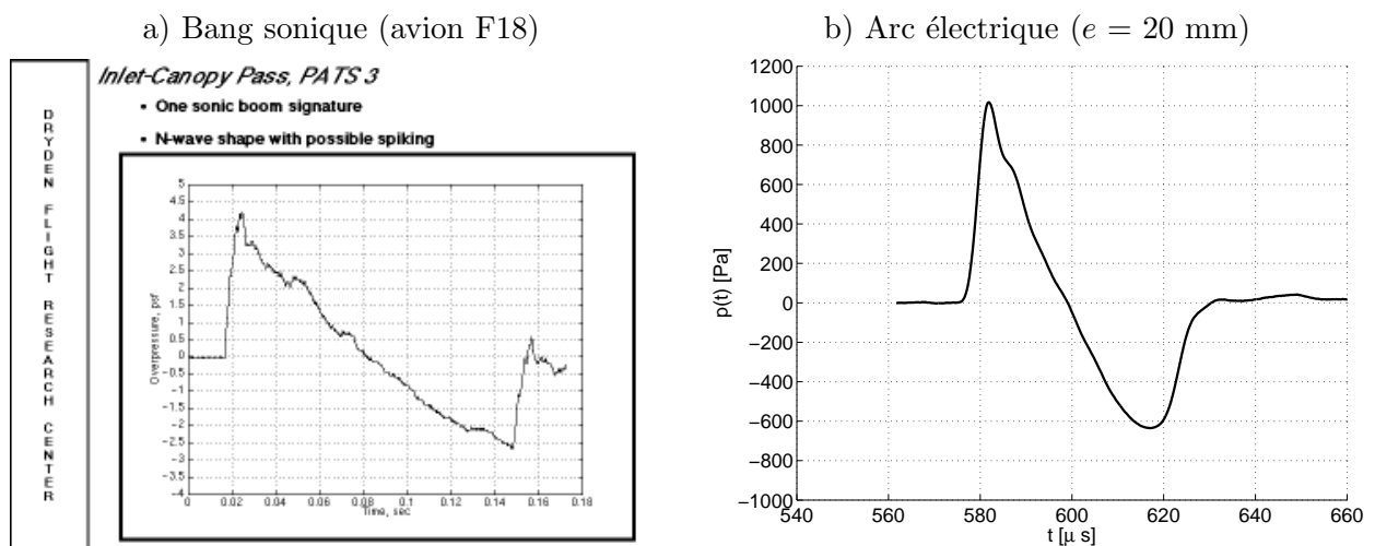
FIGURE 1.1: Formes d'ondes mesurées au sol : (a) lors du passage d'un avion supersonique F18 (d'après Hearing et al. (1995)) et (b) après claquage d'une source à arcs électriques, à 20 cm des électrodes.
