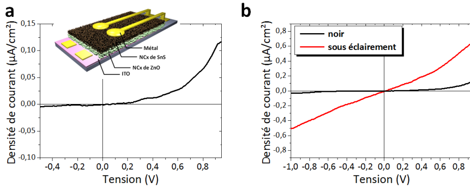
Fig. 5.15 – a) Mesure I/V de l'empilement ITO/ZnO/SnS/Au dans le noir ; b) Mesure du même dispositif sous éclairement.
