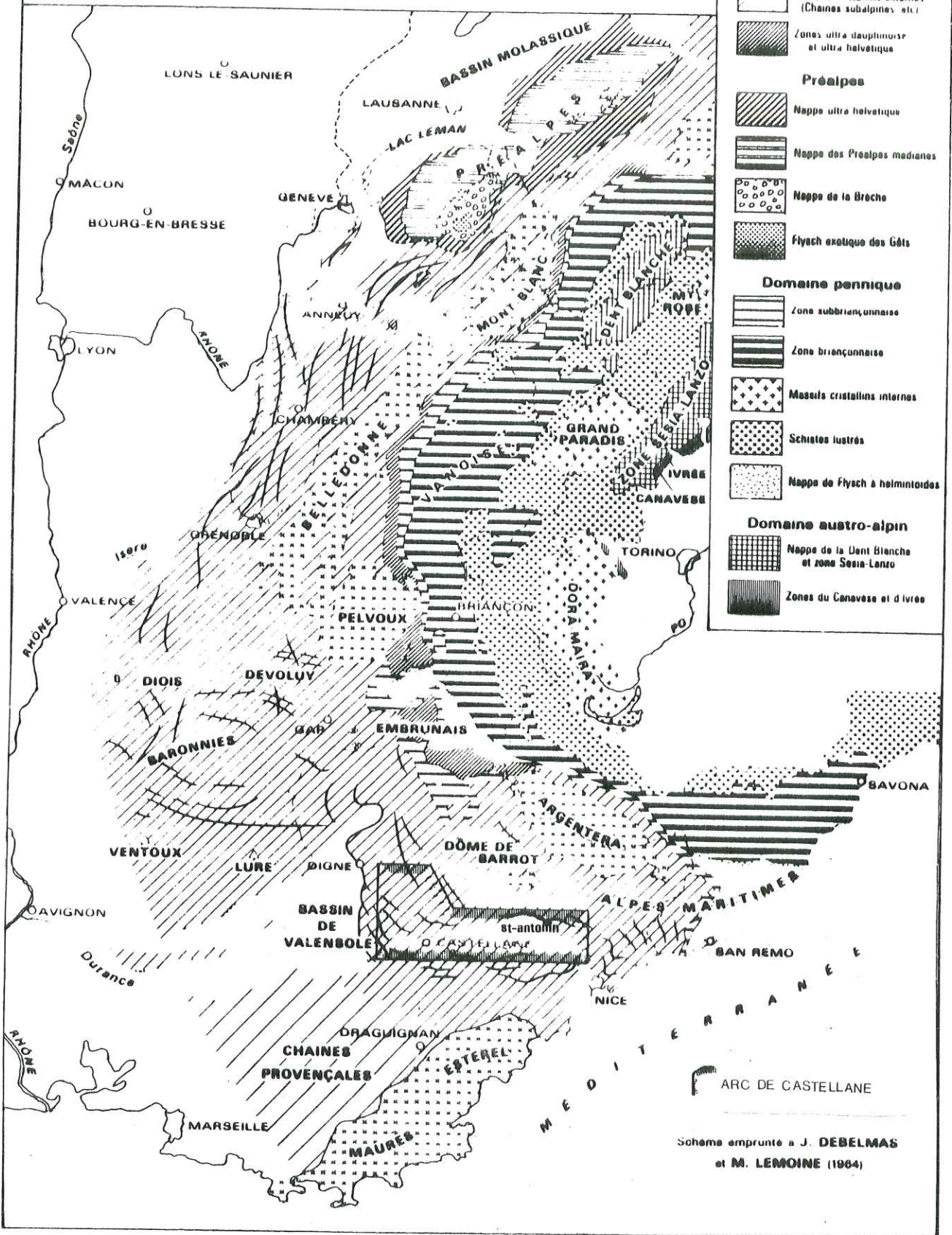
Fig.2 Délimitation de l'Arc de Castellane.
