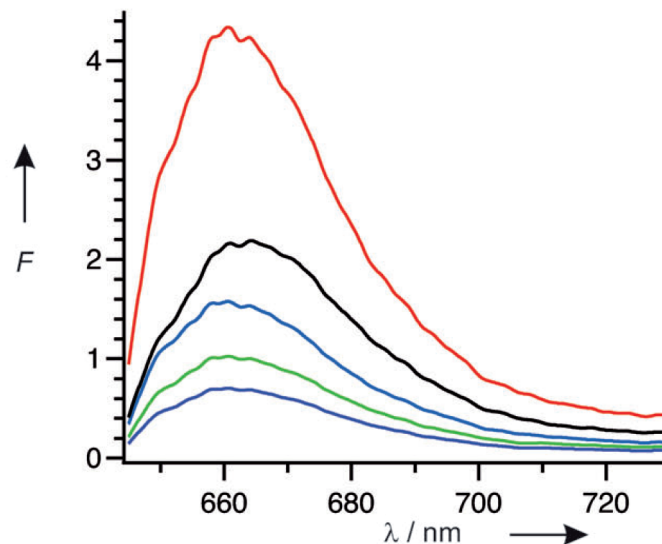
Figure 5.11 – Spectres d'émission de fluorescence normalisés par le nombre de molécules détectées dans le volume d'analyse en FCS. Les échantillons étudiés : ATTO647N (coube noire), mono50 (courbe verte), dim50 (courbe bleue), mono30 (courbe violette), dim30 (courbe rouge)
