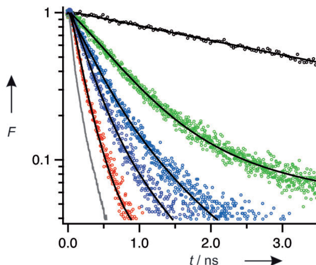
Figure 5.8 – Déclin du signal de fluorescence mesuré en TCSPC : ATTO647N (points noirs, \tau = 4.3 \pm 0.1\text{ns} ), mono50 (points verts, \tau = 615 \pm 20\text{ps} ), mono30 (points bleus, \tau = 135 \pm 15\text{ps} ), dim50 (points violets, \tau = 185 \pm 15\text{ps} ) et dim30 (points rouges, \tau = 65 \pm 10\text{ps} ), ajustés par une courbe mono-exponentielle convoluée avec la fonction de réponse d'appareil IRF (courbe grise) afin d'estimer \tau (courbes continues noires).
