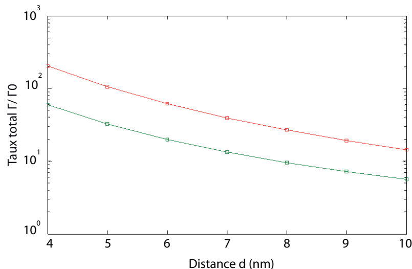
Figure 4.12 – Evolution du taux d'émission total pour un dipôle à proximité d'une NPAu de 36 nm de diamètre (ligne continue verte), ou au centre d'un dimère de NPAu (ligne continue rouge), pour \theta = \pi/4 , en fonction de la variation de la distance d , entre l'émetteur et la surface de la NPAu, Les calculs de la théorie de Mie sont représentés par les marqueurs.
