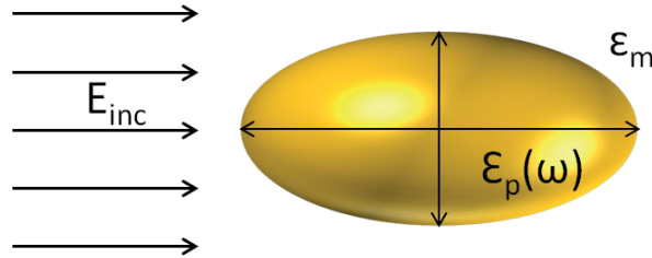
Figure 1.4 – particule elliptique longueur a pour le grand axe et b pour le petit axe, \epsilon_p , \epsilon_m sont respectivement les fonctions diélectriques de la particule et du milieu.
