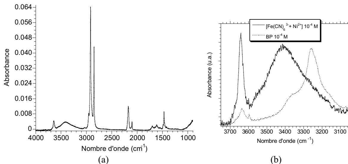
Fig. 4.6. (a) Spectre IR du film LB DODA / \text{FeCNNi} 10^{-4} M (20 couches sur \text{CaF}_2 + \text{AB} ). (b) Comparaison des bandes de vibration O-H avec celles du film LB \text{Rub}^{2+} / BP 10^{-4} M (chapitre 2).
