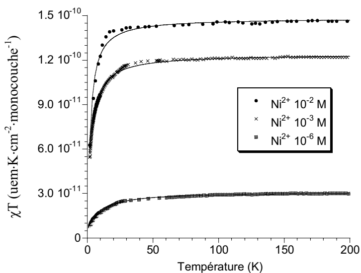
Fig. 5.26. Courbes de \chi T vs. T mesurées sous 10000 G pour les films LB RubCN / \text{Ni}(\text{ClO}_4)_2 formés à partir de différentes concentrations des sels métalliques en sous-phase. Les lignes continues correspondent aux meilleurs ajustements pour le modèle décrit dans le texte.
