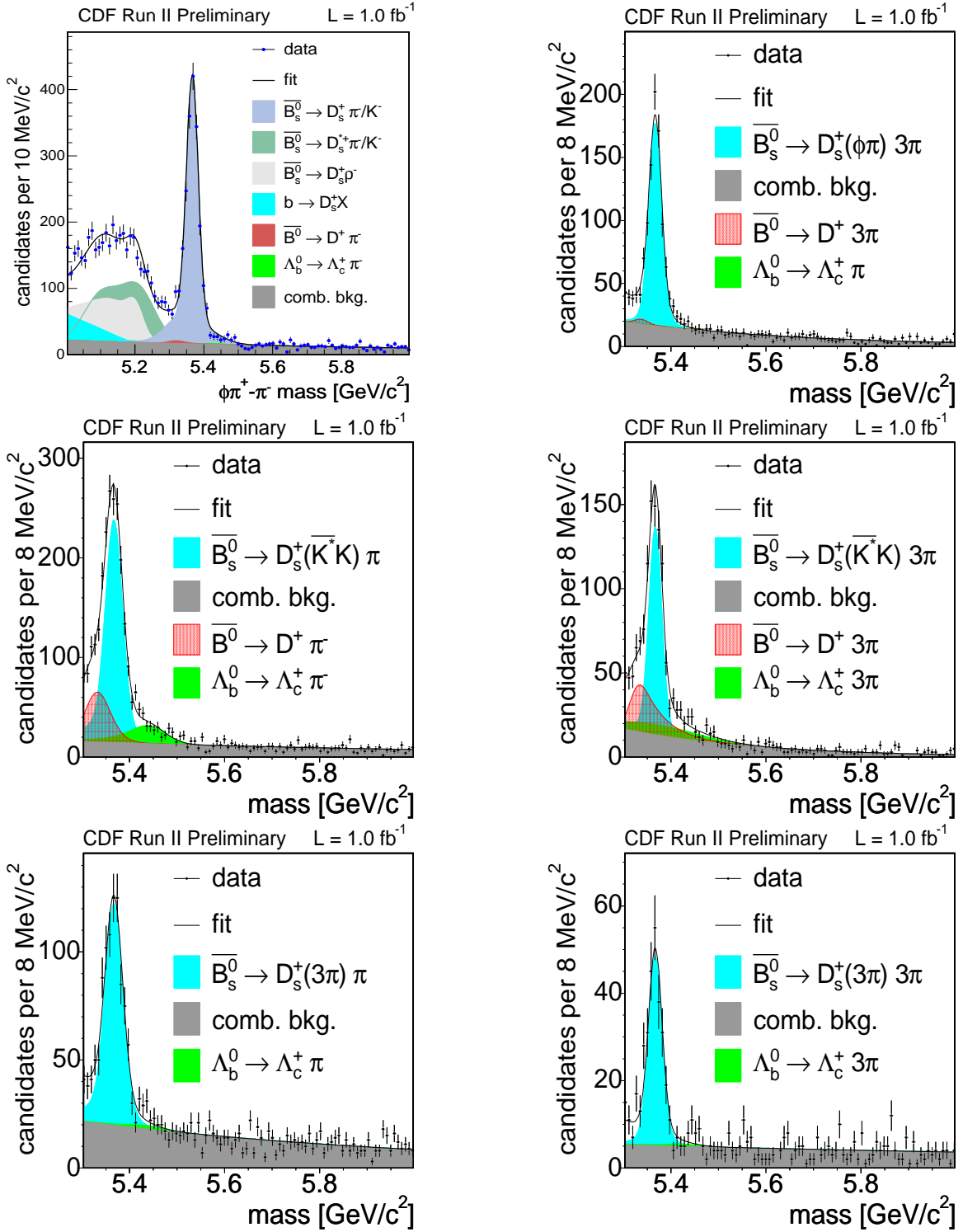
FIGURE B.3: Spectres de masse hadronique, qui montrent tous les composants des échantillons. Dans la colonne à gauche les désintégrations B_s^- \rightarrow D_s^- \pi^+ \pi^- , dans la colonne à droite les désintégrations B_s^- \rightarrow D_s^- \pi^- \pi^+ \pi^- . De haut au bas les désintégrations D_s^- \rightarrow \phi \pi^- , D_s^- \rightarrow K^{*0} K^- , D_s^- \rightarrow \pi^+ \pi^- \pi^- .
