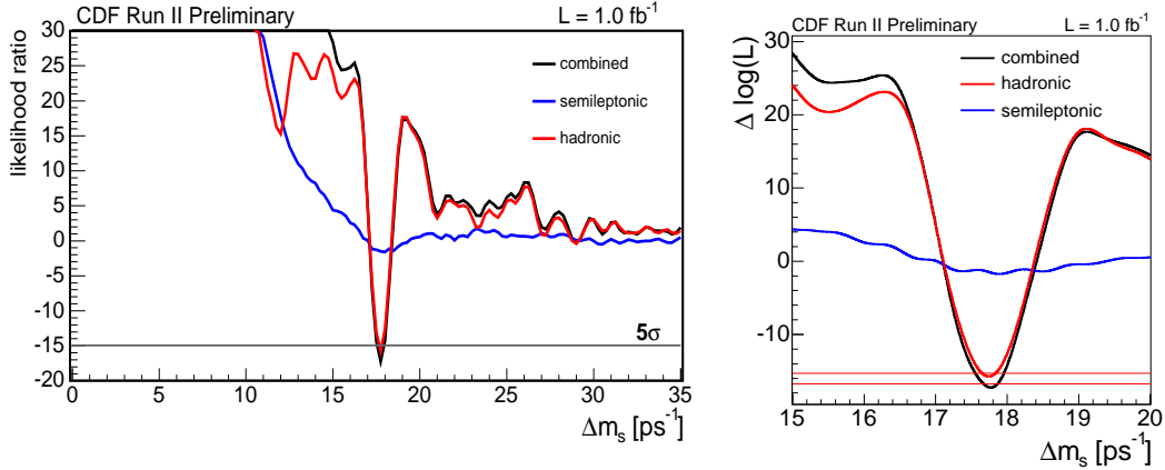
FIGURE B.7: Profil du rapport de probabilité: rapport de la fonction de vraisemblance en fonction de \Delta m_s (à gauche) avec un zoom sur la region [15, 20] \text{ps}^{-1} . La contribution hadronique (rouge), semileptonique (bleu) et leur combinaison (noir) sont montrées séparément .
