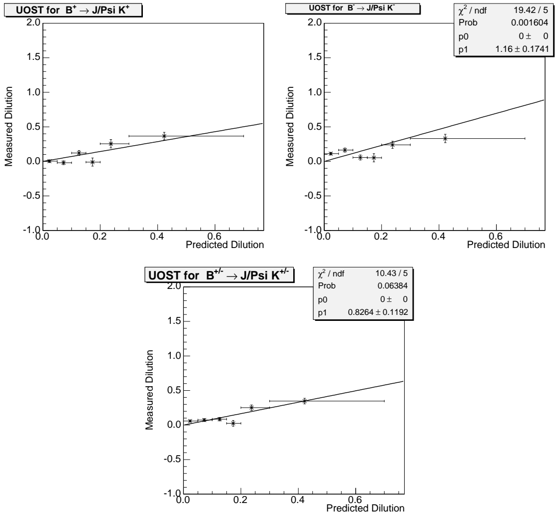
FIGURE B.12: Dilution mesurée en fonction de la dilution événement-par-événement pour B^+ (en haut à gauche), B^- (en haut à droite) et l'échantillon B^+ entiers (en bas). L'ajustement relatif est dessiné.
