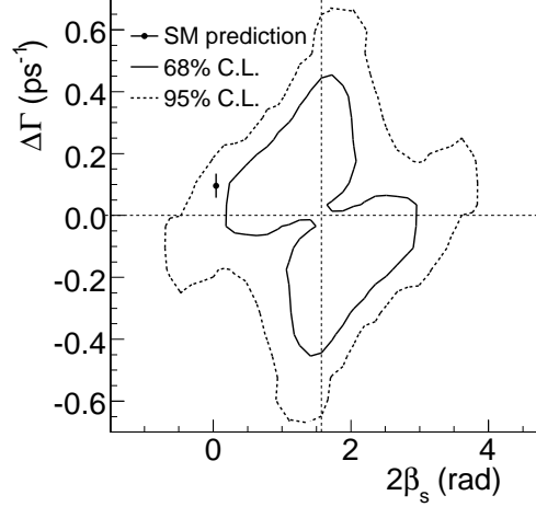
FIGURE B.14: A gauche: Le contours du niveau de confiance dans le plan \beta_s - \Delta\Gamma_s basé sur les algorithmes d'étiquetage de la saveur. Le niveaux de confiance a 68% sont indiqués en trait plein, ceux à 95% sont en trait à tiret. La solution avec \Delta\Gamma_s > 0 correspond à \cos(\delta_\perp) < 0 et \cos(\delta_\perp - \delta_\parallel) > 0 . Le contraire est vrai pour la solution avec \Delta\Gamma_s < 0 . Le point noir correspond à la prediction du Modèle Standard, \Delta\Gamma_s = 0.096 \text{ ps}^{-1} et \beta_s = 0.02 [75].
