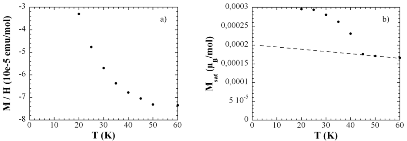
Figure 70 : Evolution de a) la partie linéaire à au champ des courbes d'aimantation et b) de l'aimantation à saturation ( M_{sat} ) en fonction de la température.
