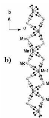
Figure 4: Réseau bidimensionnel dans 4 formé par les sites Mo et Mn1 dans le plan a) bc et b) vue suivant la direction c .
