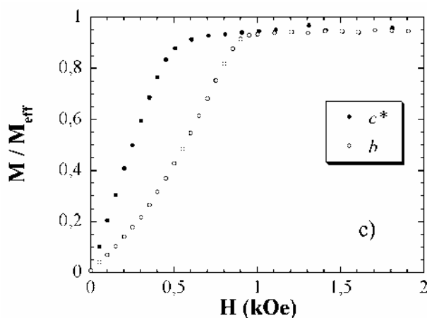
Figure 38 : Evolution de l'aimantation normalisée à M_{eff} en fonction du champ magnétique dans la partie bas champ pour a) 1, b) 2, c) 3 à 2 K.
