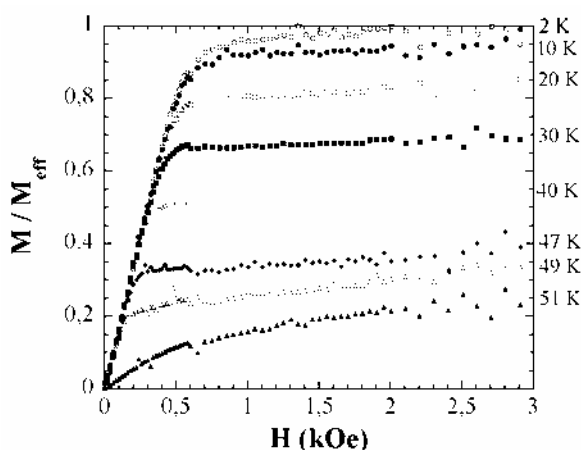
Figure 39 : Evolution de l'aimantation normalisée à M_{\text{eff}} de 2 en fonction du champ magnétique à différentes températures.
