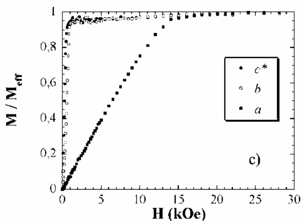
Figure 37 : Evolution de l'aimantation normalisée à M_{eff} en fonction du champ magnétique dans les directions b et les extrema de la rotation dans le plan a^*c pour a) 1, b) 2, c) 3 à 2 K.
