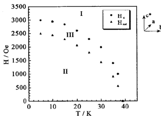
Figure 20 : Diagramme de phases de 2 lorsque le champ magnétique est appliqué parallèlement à la direction c^* selon ref.[42].
