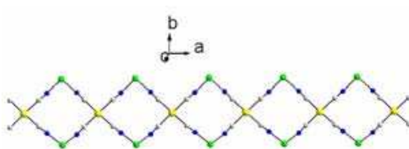
Figure 53 : Réseau « carré » dans 1.
