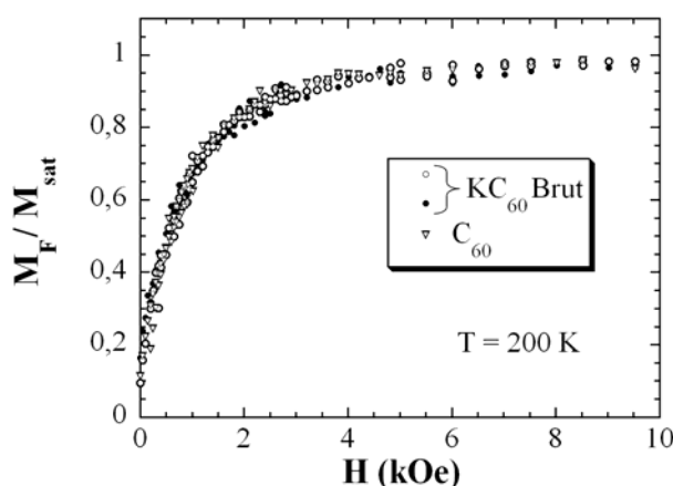
Figure 42 : Evolution de l'aimantation normalisée à l'aimantation à saturation ( M_{sat} ) en fonction du champ magnétique de deux échantillons bruts et du C_{60} .
