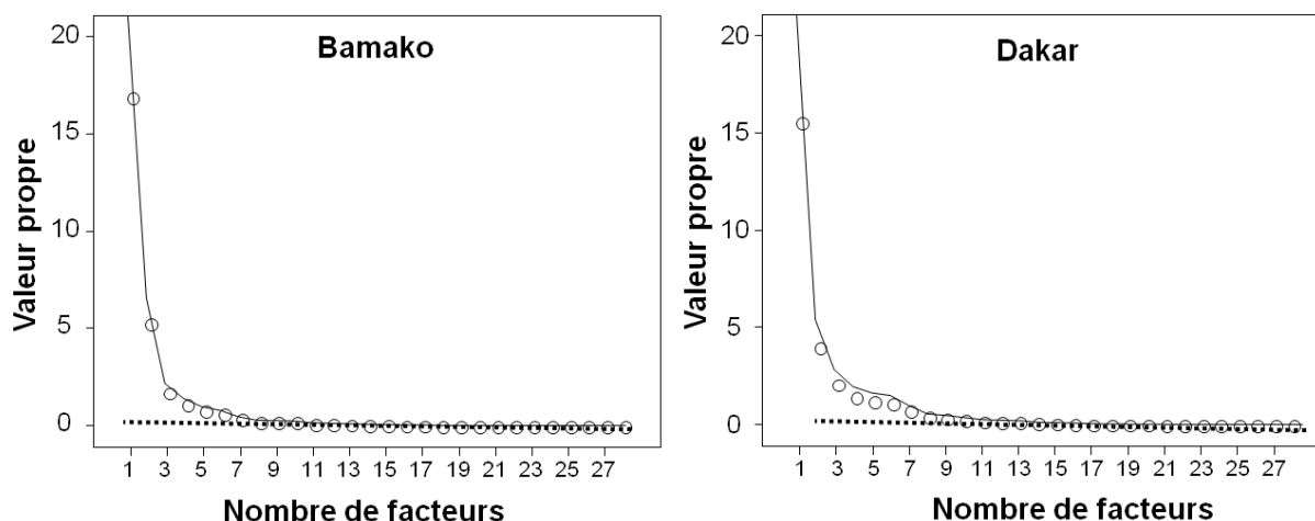
Figure IV.1: Courbe de décroissance des valeurs propres en fonction du nombre de facteurs : cas de Bamako et Dakar.
