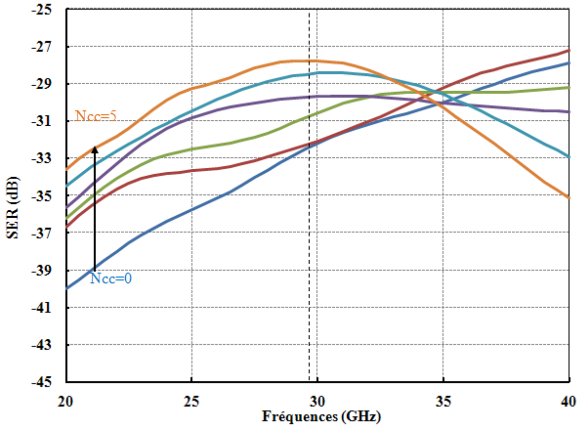
Figure III-16 : Variation fréquentielle de la SER pour les 6 différentes configurations. Ncc = Nombre de dipôles court-circuités
